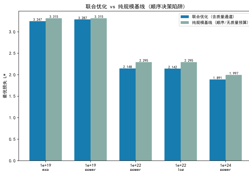
图 7.51 联合优化 vs 纯规模基线的最优损失（顺序决策陷阱：质量需预算预留）。
