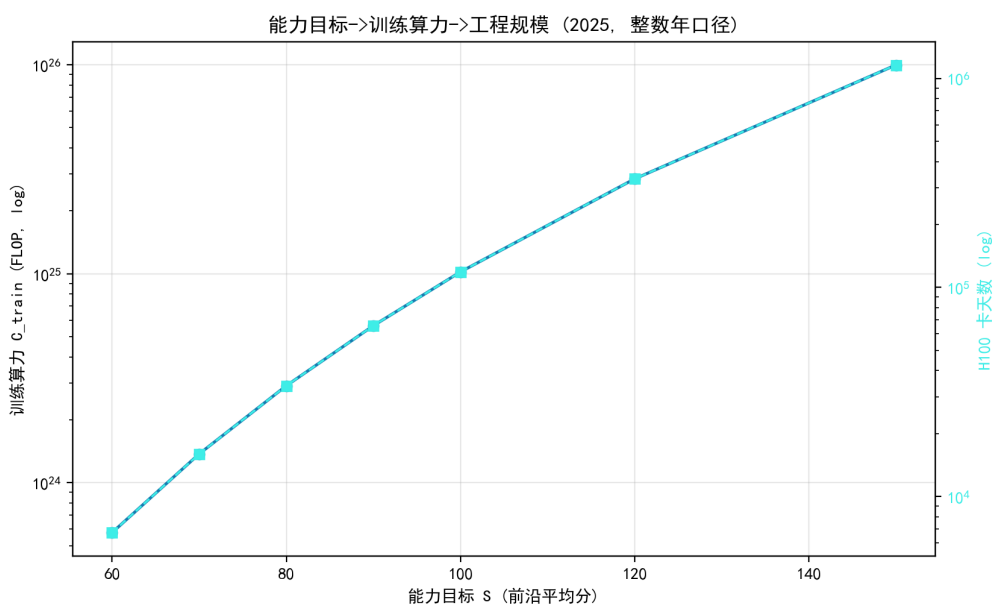
图 8.62 能力目标 \rightarrow 训练算力（对数轴）：S=90 约需 6.6 万卡天。
