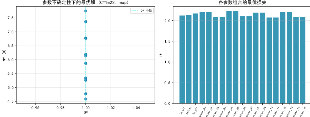
图 7.42 参数角点下的最优解： Q^*=1 稳定、 L^* 带宽 \pm 3.5\% 、 N^* \pm 28\% 。
