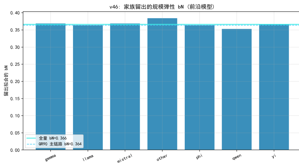
图 8.70 家族留下的规模弹性 b_N ：全家族稳定在 0.36 附近。
