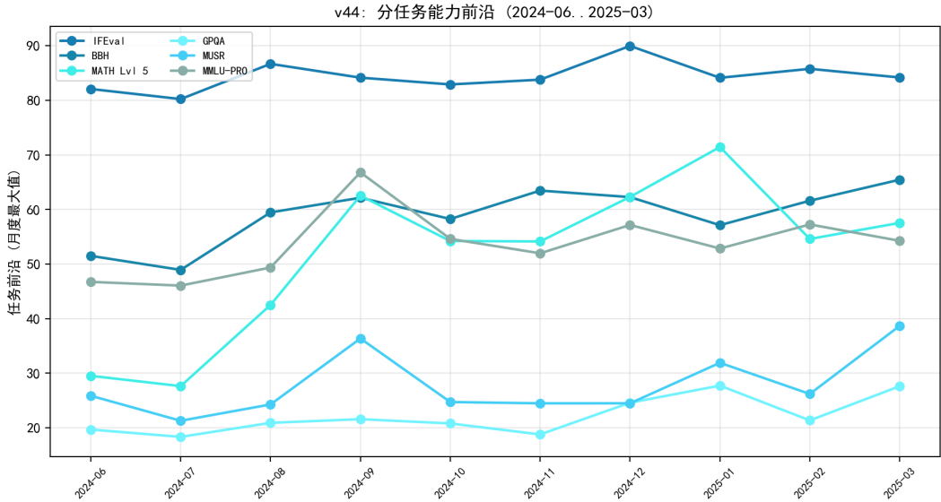
图 8.63 分任务能力前沿：推理类（MATH/GPQA/MUSR）增长快于知识/指令类。
