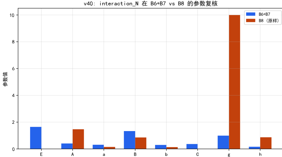
图 6.24 B8 原样 vs B6+B7 的参数对比：B8 质量项退化（ E = C = 0 ， g 撞界）。
