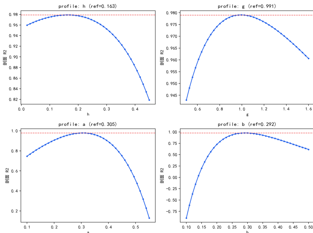
图 6.25 关键参数的剖面似然曲线（红色虚线为 90% 似然比阈值）。
