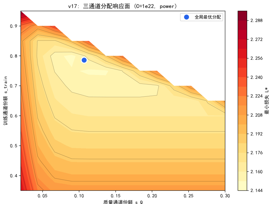
图 7.45 三通道分配响应面（ C = 10^{22} ，幂成本；蓝点为全局最优分配）。
