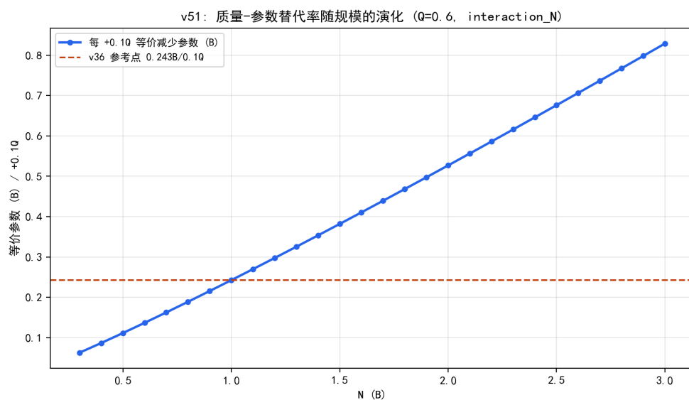
图 6.29 每 +0.1Q 等价减少的参数随规模的演化（近线性上升）。
