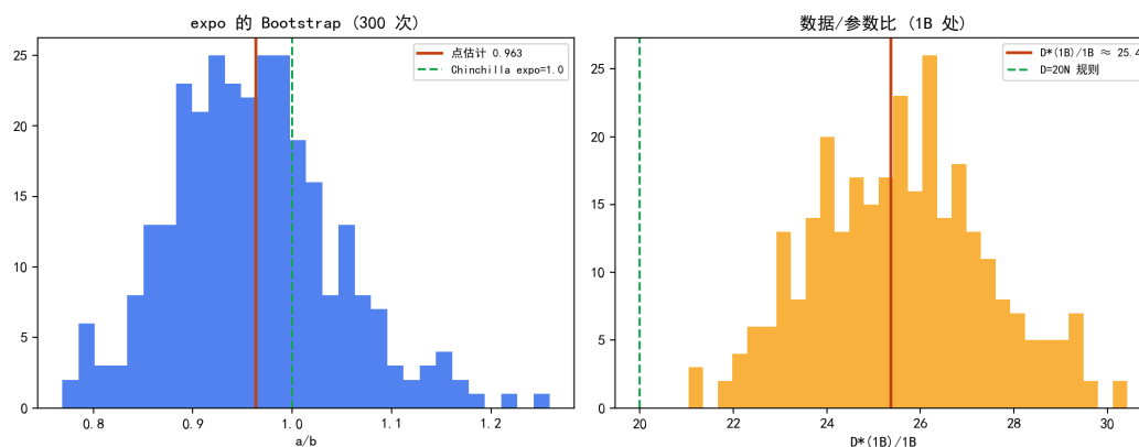
图 7.37 D^*(N) 参数 Bootstrap: 指数 CI 含 1.0, 常数 CI 高于 D = 20N 。
