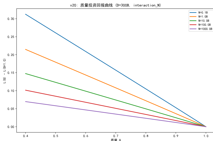
图 6.26 质量投资回报曲线 ( D = 300B ): L(Q) 相对 L(Q = 1) 随 N 变化。
