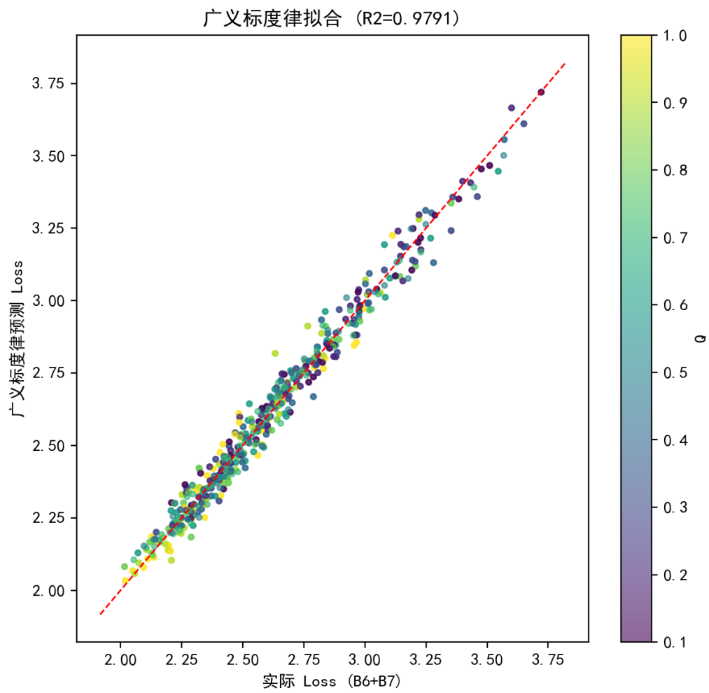
图 6.22 广义标度律在 B6+B7 数据上的拟合（质量-参数数量交互形式， R^2 = 0.979 ）。
