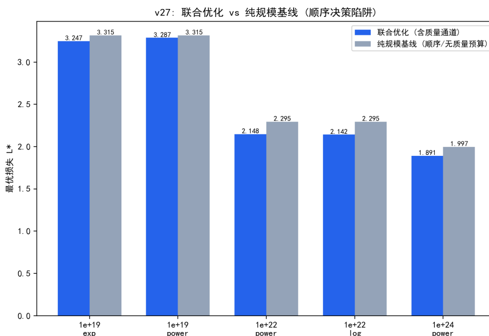
图 7.43 联合优化 vs 纯规模基线的最优损失（顺序决策陷阱：质量需预算预留）。
