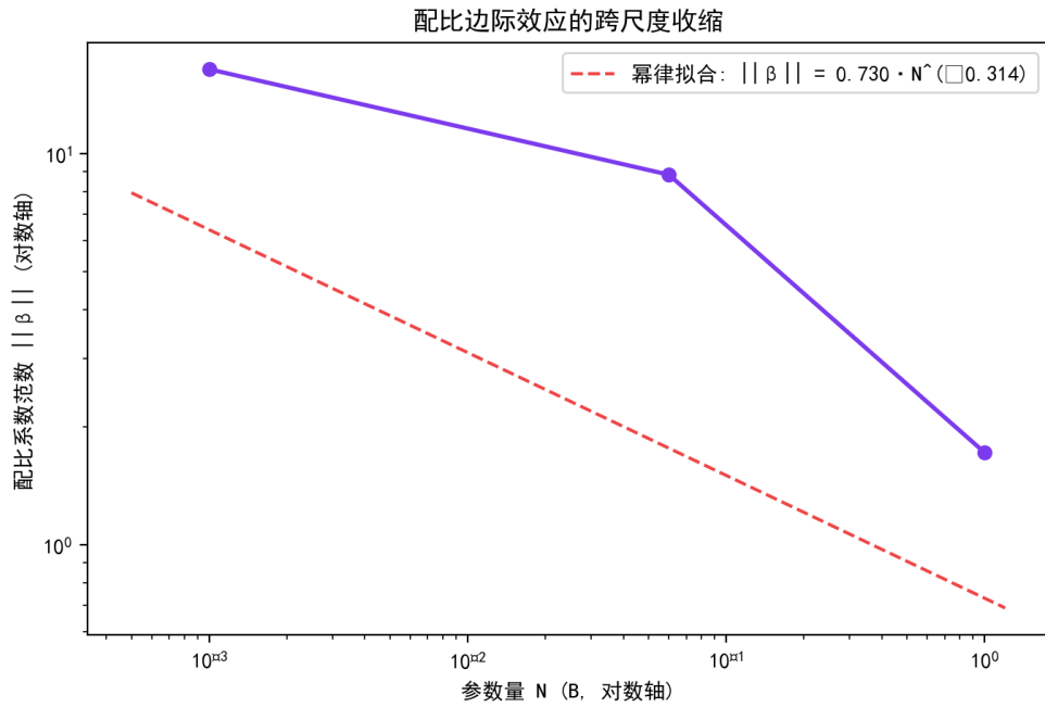
图 5.4 配比系数范数随模型规模幂律收缩 ( \kappa = 0.314 )。
