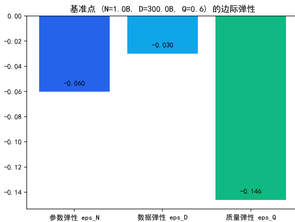
图 6.15 基准点处三个维度的损失弹性对比 (质量弹性最高)。
