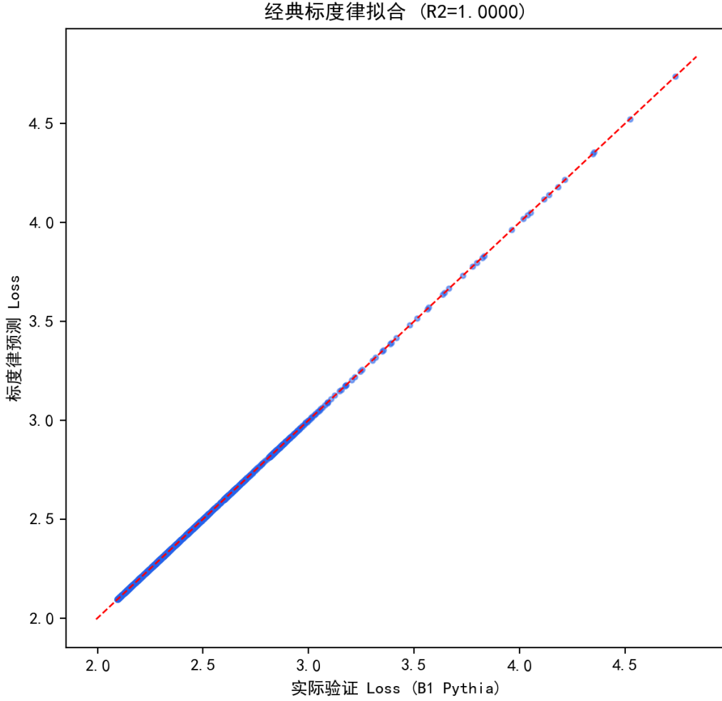
图 6.9 经典标度律在 B1 轨迹上的拟合与跨家族验证。
