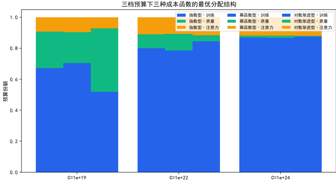
图 7.17 三档预算下三种质量成本函数的最优成本份额结构。
