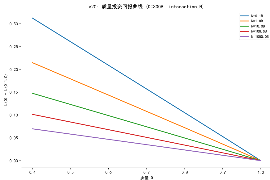
图 6.14 质量投资回报曲线 ( D = 300B ): L(Q) 相对 L(Q = 1) 随 N 变化。
