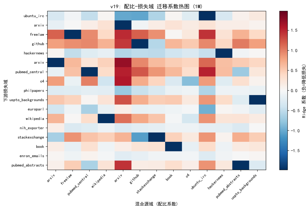
图 5.6 配比源域 \times 损失域迁移系数热图（1M 尺度，负值 = 压低损失）。
