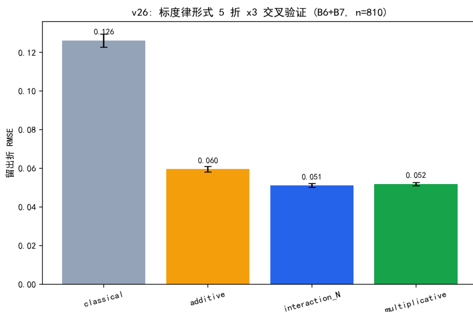
图 6.10 标度律形式 5 折交叉验证的留出 RMSE 对比。
