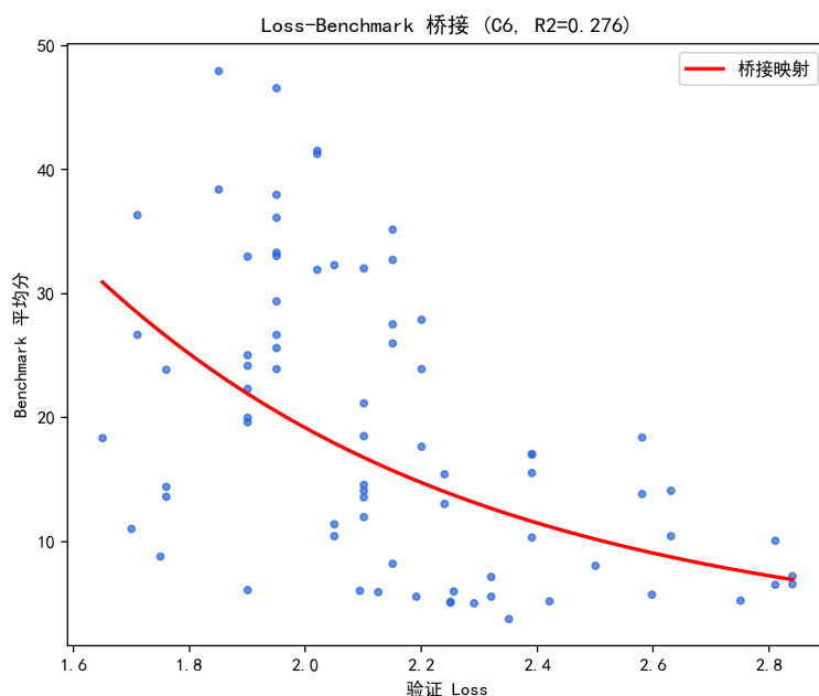
图 8.32 Loss–Benchmark 桥接映射（C6，75 个模型）。
