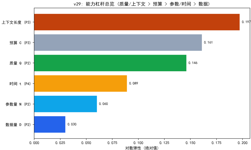
图 10.36 能力杠杆总览：各投入的对数弹性排序（质量/上下文 > 预算 > 参数/时间 > 数据）。
