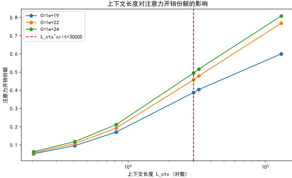
图 7.22 注意力开销份额随上下文长度的变化（红色虚线为临界点 30000）。
