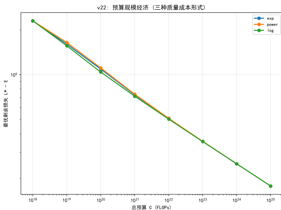
图 7.18 预算-最优损失的对数线性规律（三种质量成本形式）。
