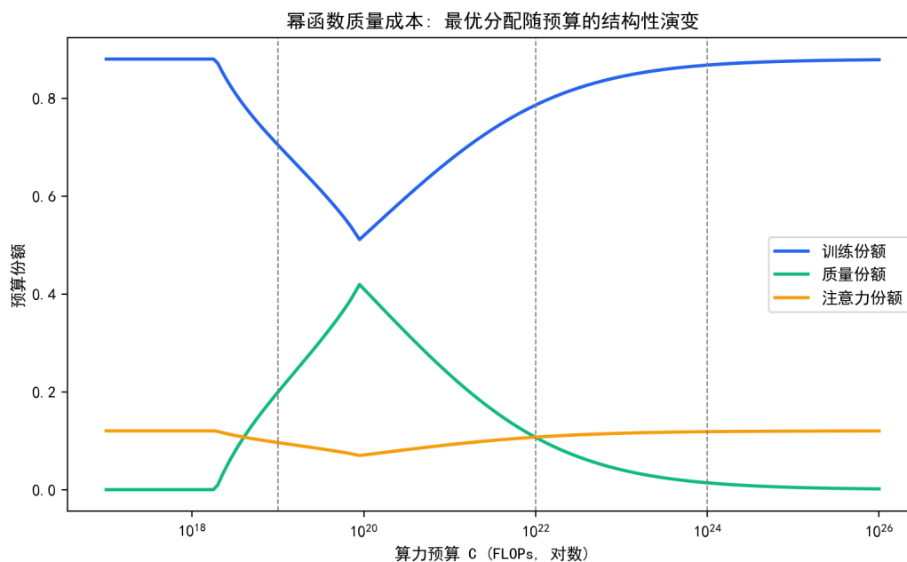
图 7.20 幂函数质量成本下最优成本份额随预算的结构性演变（竖线为三档预算）。
