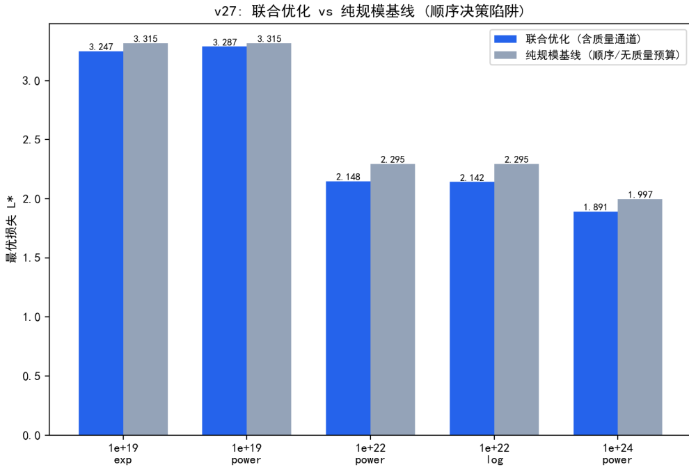
图 7.24 联合优化 vs 纯规模基线的最优损失 (顺序决策陷阱: 质量需预算预留)。
