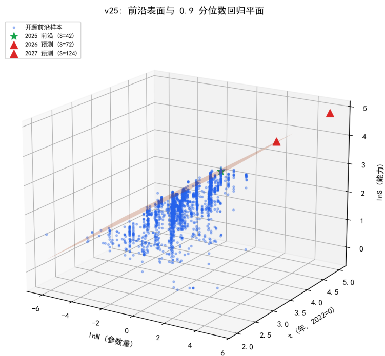
图 8.30 能力前沿 3D 表面与 0.9 分位数回归平面（星标 = 2025 前沿，三角 = 预测点）。
