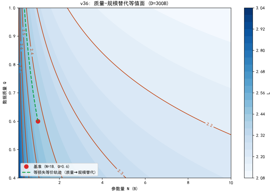
图 6.16 质量-规模替代等值面：等损失轨迹显示质量对参数的替代关系。
