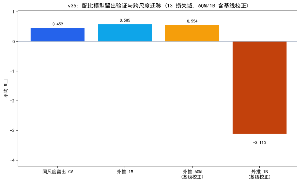
图 5.5 配比模型留出验证与跨尺度迁移（60M/1B 为基线校正口径）。
