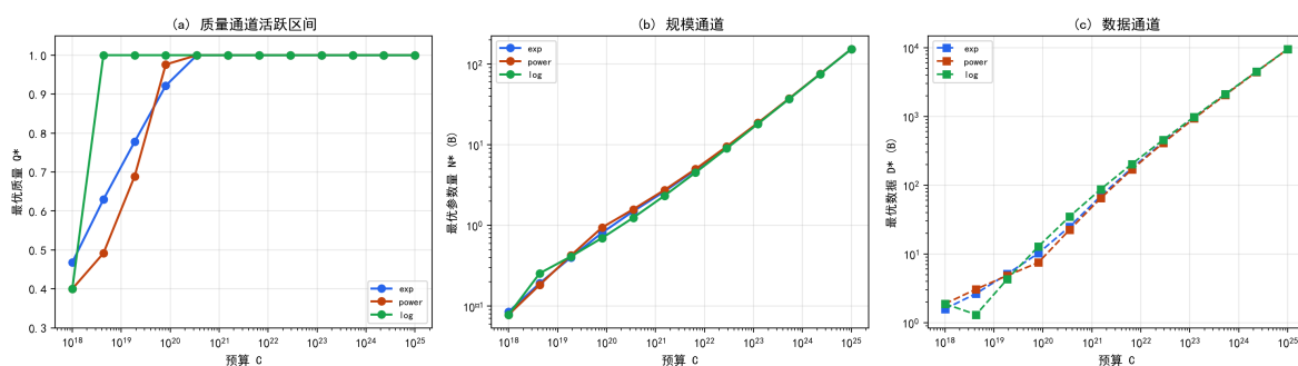
图 7.21 最优解族随预算轨迹：质量通道活跃区间由成本形式决定。
