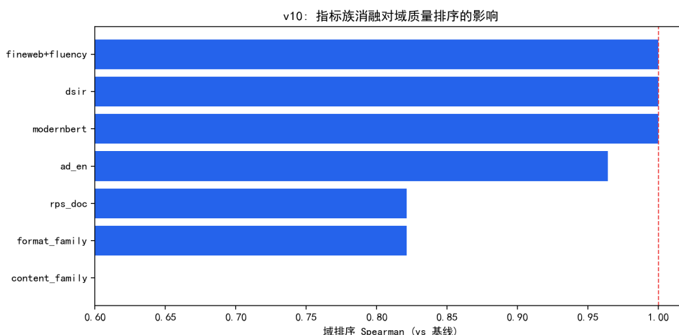
图 9.34 指标族消融对域质量排序的影响（红虚线为完全一致）。
