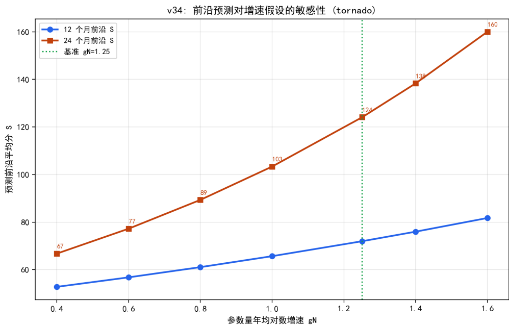
图 8.27 前沿预测对参数量增速假设 g_N 的敏感性（12/24 个月）。
