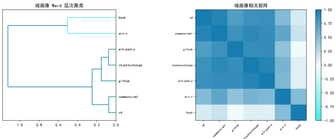
图 5.18 域画像层次聚类与相关矩阵：book 独树一帜、低质域聚簇。
