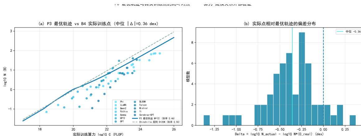
图 7.54 闭环对照: P3 最优轨迹与 B4 实际训练点 (左); 偏差分布 (右)。中位偏差 0.36 \text{ dex} , 优于 Chinchilla 规则 30%。
