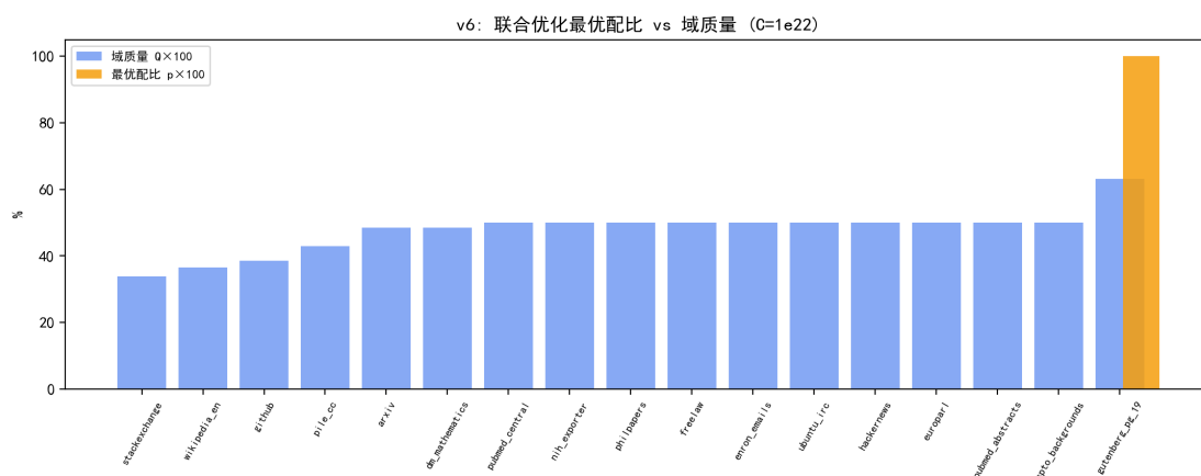
图 7.21 联合优化最优配比与域质量对比（ C = 10^{22} ）：配比向最高质量域（小说）集中。
