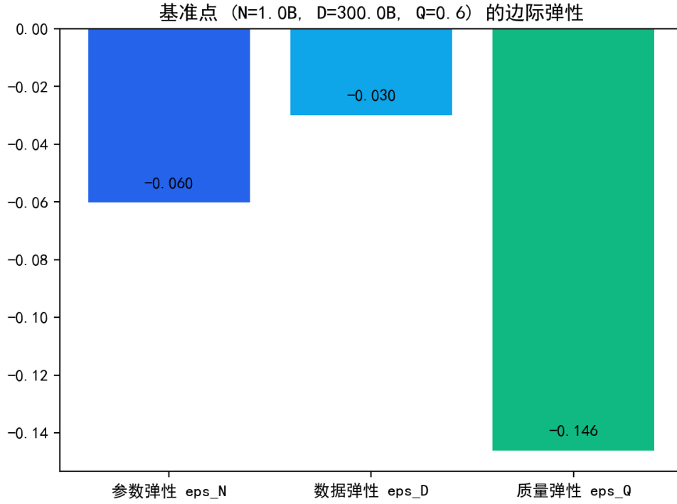
图 6.14 基准点处三个维度的损失弹性对比（质量弹性最高）。
