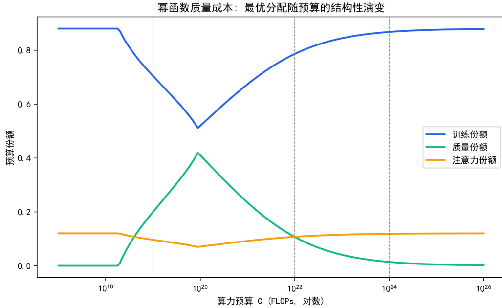
图 7.18 幂函数质量成本下最优成本份额随预算的结构性演变（竖线为三档预算）。
