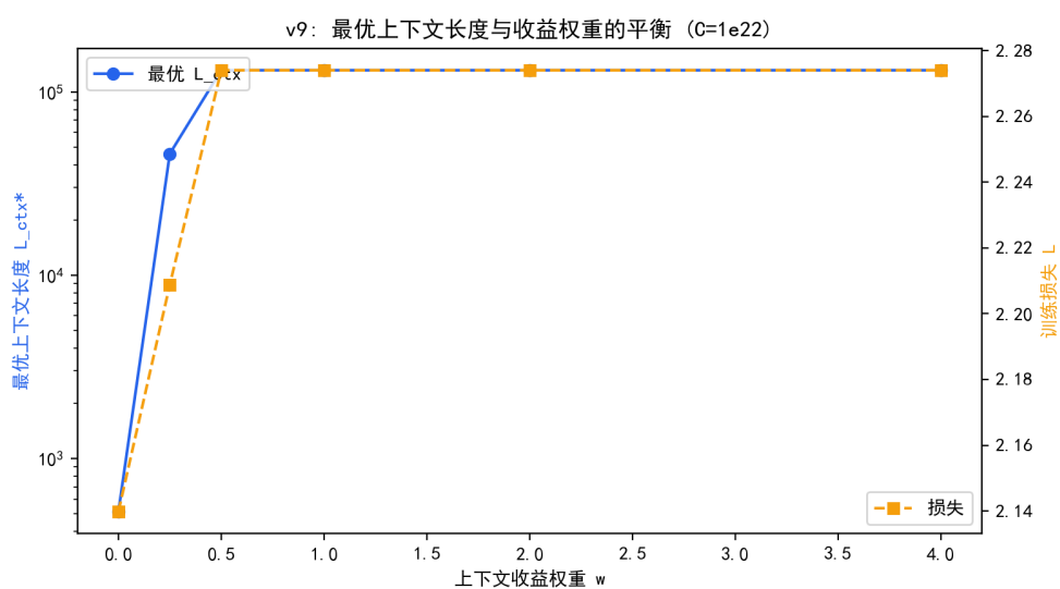
图 7.23 最优上下文长度与收益权重 w 的平衡 ( C = 10^{22} )。
