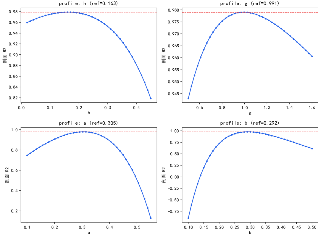
图 6.12 关键参数的剖面似然曲线（红色虚线为 90% 似然比阈值）。
