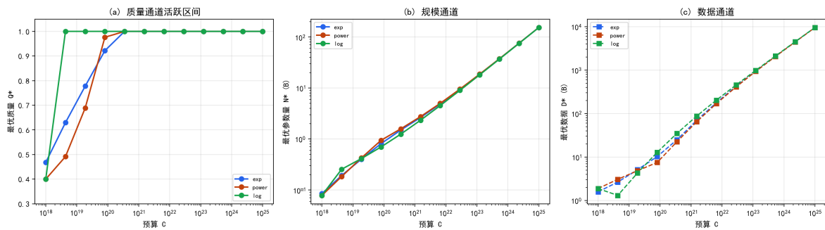
图 7.19 最优解族随预算轨迹：质量通道活跃区间由成本形式决定。
