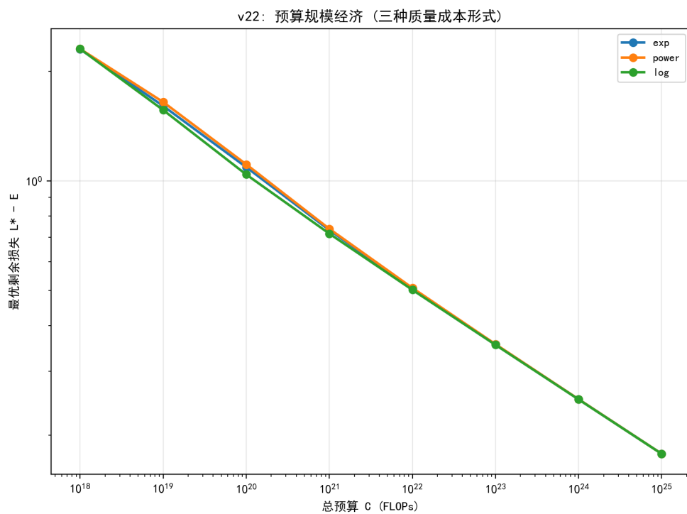
图 7.16 预算-最优损失的对数线性规律 (三种质量成本形式)。
