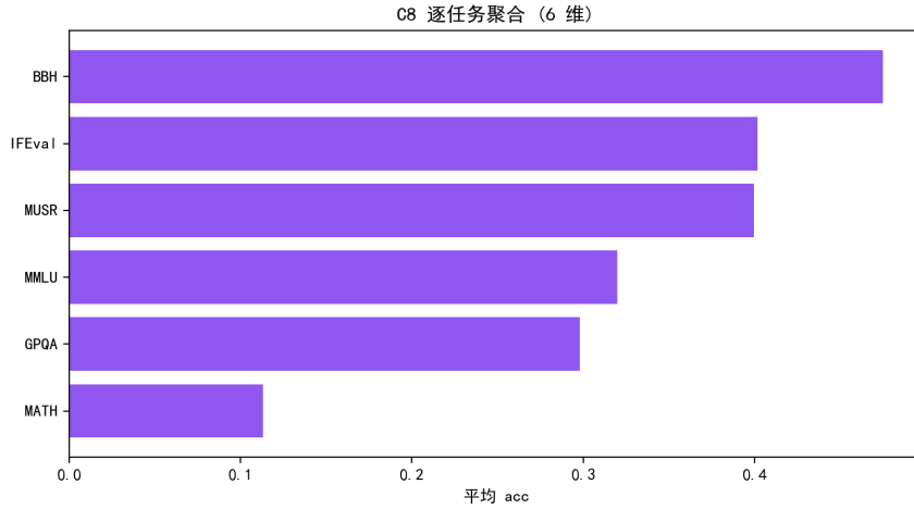
图 8.31 C8 逐任务聚合得分 (6 维)。
