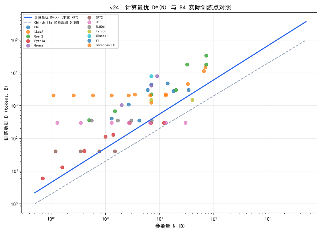
图 7.17 计算最优数据曲线 D^*(N) 、Chinchilla 经验规则与 B4 实际训练点。
