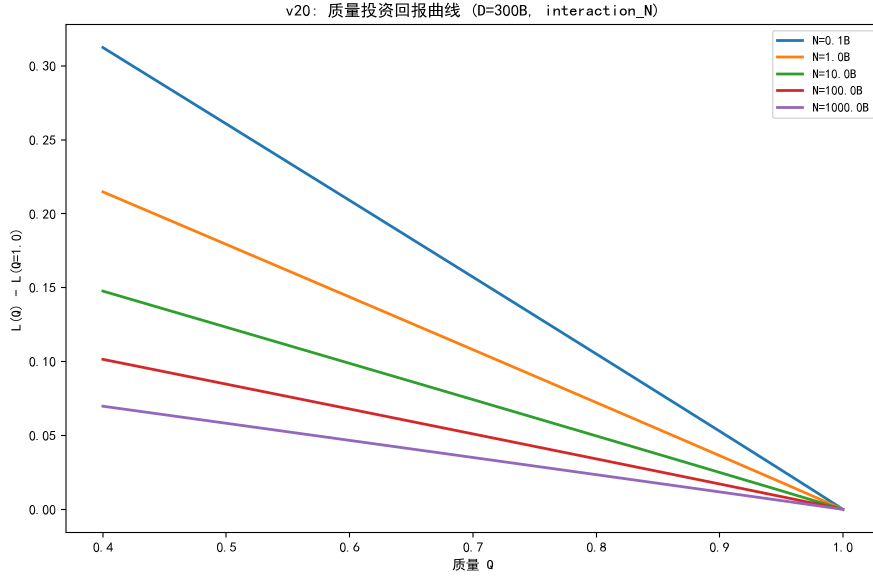
图 6.13 质量投资回报曲线 ( D = 300B ): L(Q) 相对 L(Q = 1) 随 N 变化。
