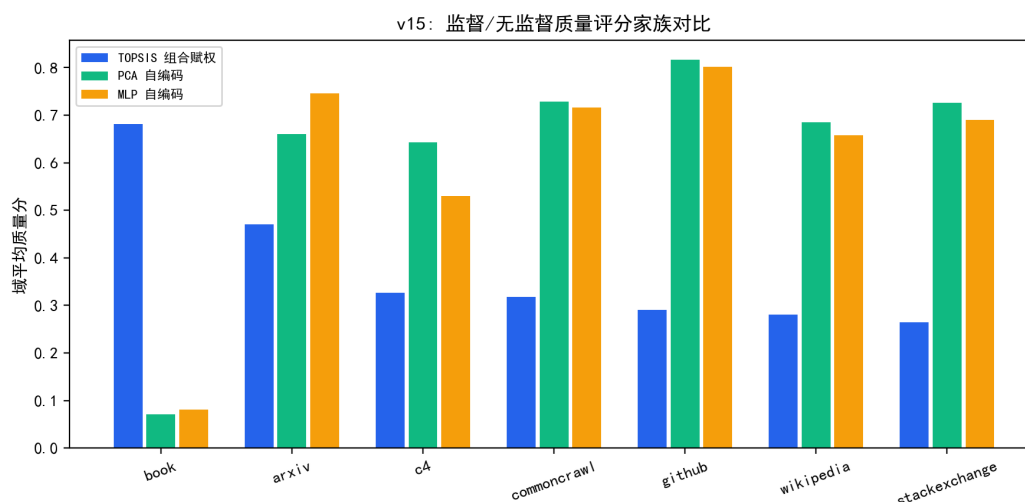
图 9.33 Topsis 组合赋权与自编码典型性评分的域级对照（方向相反）。
