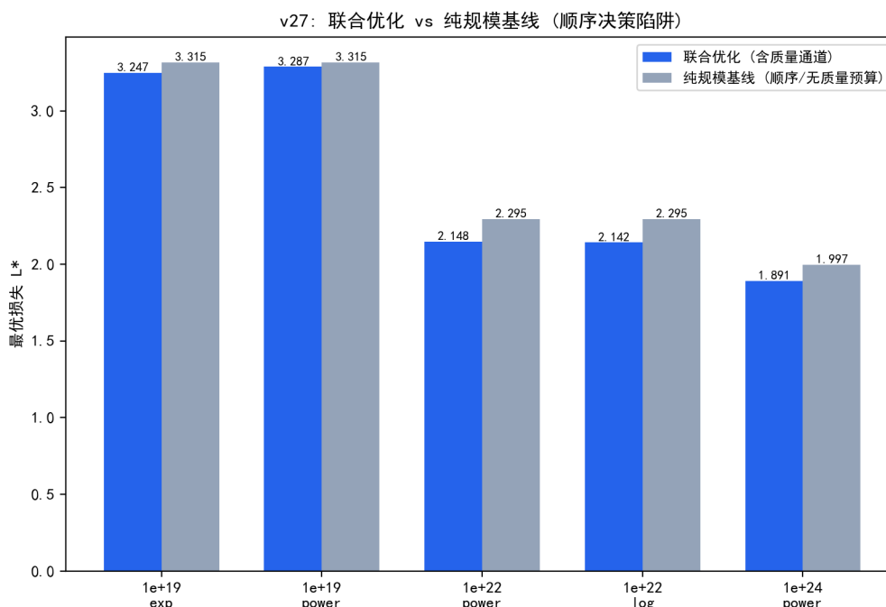
图 7.22 联合优化 vs 纯规模基线的最优损失（顺序决策陷阱：质量需预算预留）。
