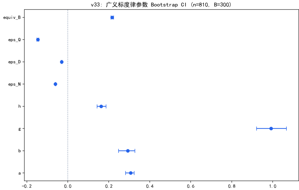
图 6.24 广义标度律参数与弹性的 Bootstrap 置信区间。
