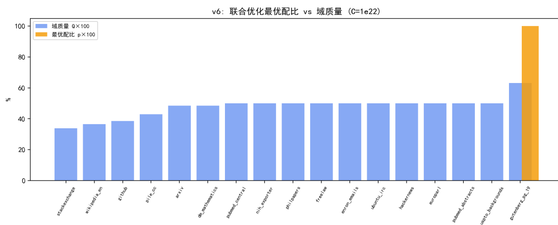
图 7.44 联合优化最优配比与域质量对比 ( C = 10^{22} ): 配比向最高质量域 (小说) 集中。
