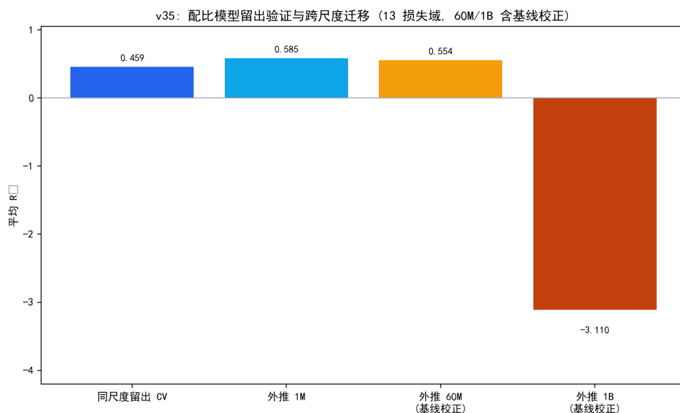
图 5.7 配比模型留出验证与跨尺度迁移（60M/1B 为基线校正口径）。
