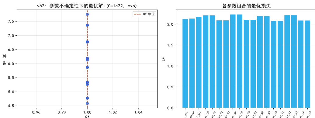
图 7.36 参数角点下的最优解：Q*=1 稳定、L* 带宽 \pm 3.5\% 、N* \pm 28\% 。
