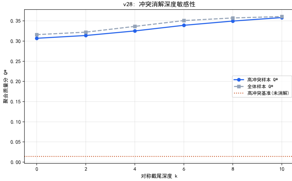
图 5.4 冲突消解深度敏感性：高冲突样本质量分随 k 单调上升。
