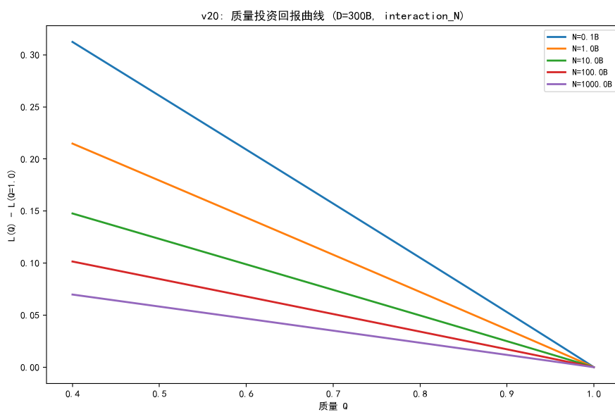
图 6.27 质量投资回报曲线（ D = 300B ）： L(Q) 相对 L(Q = 1) 随 N 变化。
