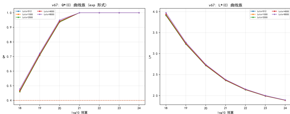
图 7.37 上下文长度 \times 预算响应面：L* 路径几乎不随 L_{ctx} 移动。
