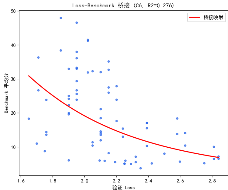
图 8.12 Loss–Benchmark 桥接映射（C6，75 个模型）。
