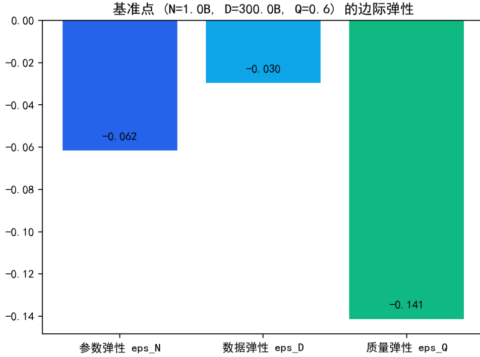
图 6.6 基准点处三个维度的损失弹性对比（质量弹性最高）。
