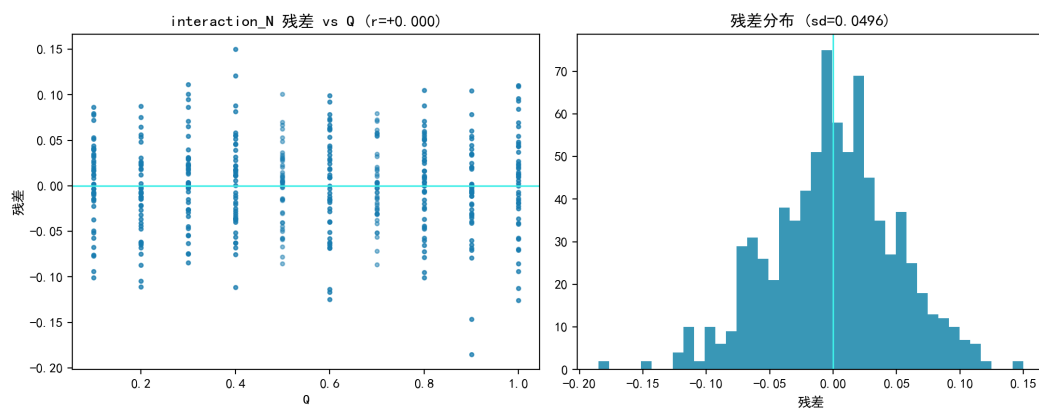
图 6.23 interaction_N 残差诊断：与 Q 无相关、分布近对称。
