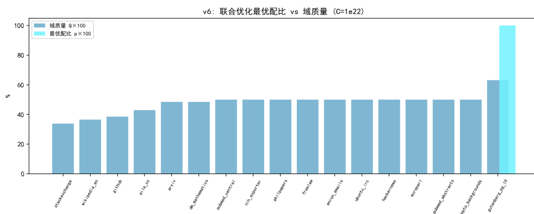
图 7.48 联合优化最优配比与域质量对比 ( C = 10^{22} )：配比向最高质量域（小说）集中。
