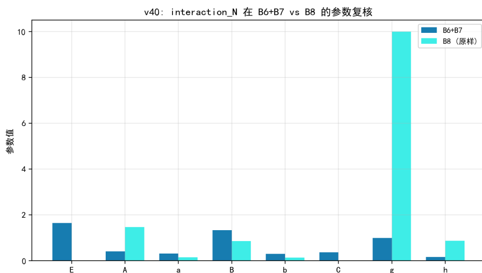
图 6.28 B8 原样 vs B6+B7 的参数对比：B8 质量项退化（ E = C = 0 ， g 撞界）。
