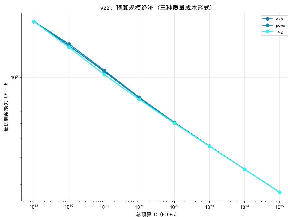
图 7.38 预算-最优损失的对数线性规律（三种质量成本形式）。
