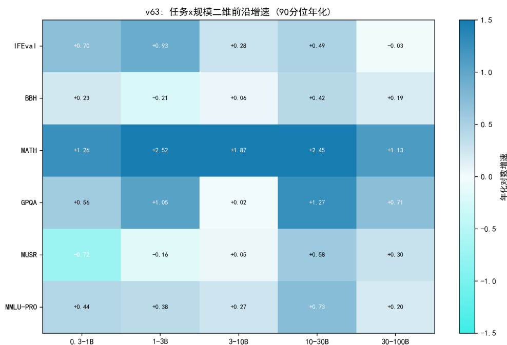
图 8.65 任务 × 规模二维前沿增速：MATH/GPQA 在 1–3B 与 10–30B 双峰。
