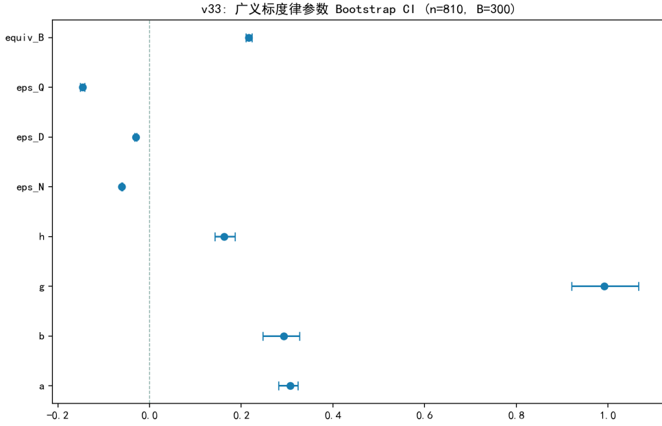
图 6.27 广义标度律参数与弹性的 Bootstrap 置信区间。
