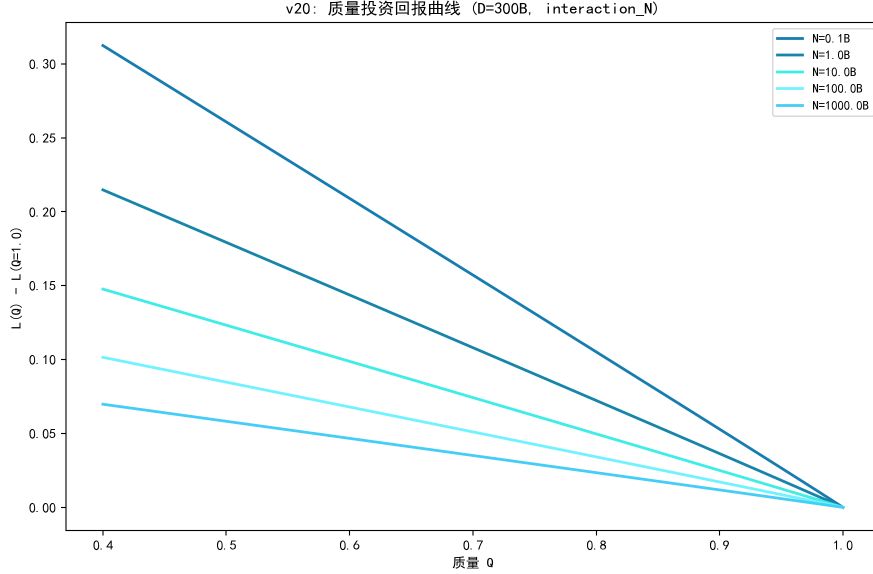
图 6.30 质量投资回报曲线 ( D = 300B ): L(Q) 相对 L(Q = 1) 随 N 变化。
