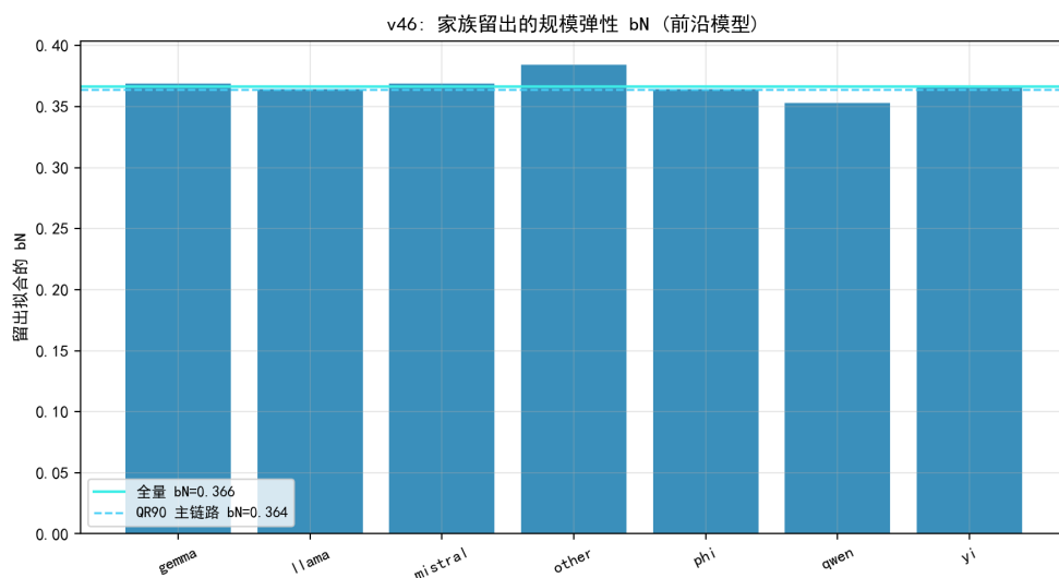
图 8.70 家族留出的规模弹性 b_N ：全家族稳定在 0.36 附近。
