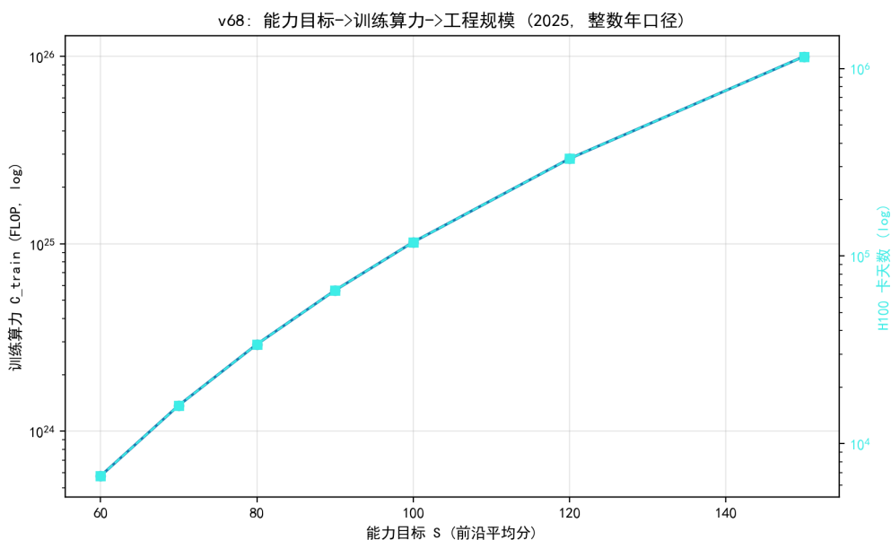
图 8.60 能力目标 → 训练算力（对数轴）：S=90 约需 6.6 万卡天。
