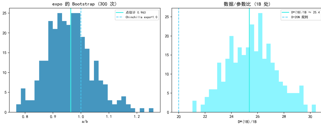
图 7.43 D^*(N) 参数 Bootstrap: 指数 CI 含 1.0, 常数 CI 高于 D = 20N 。
