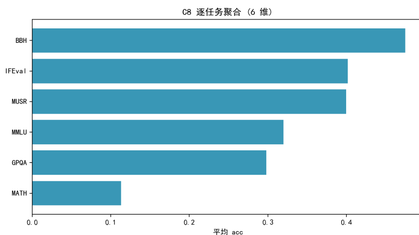
图 8.73 C8 逐任务聚合得分 (6 维)。
