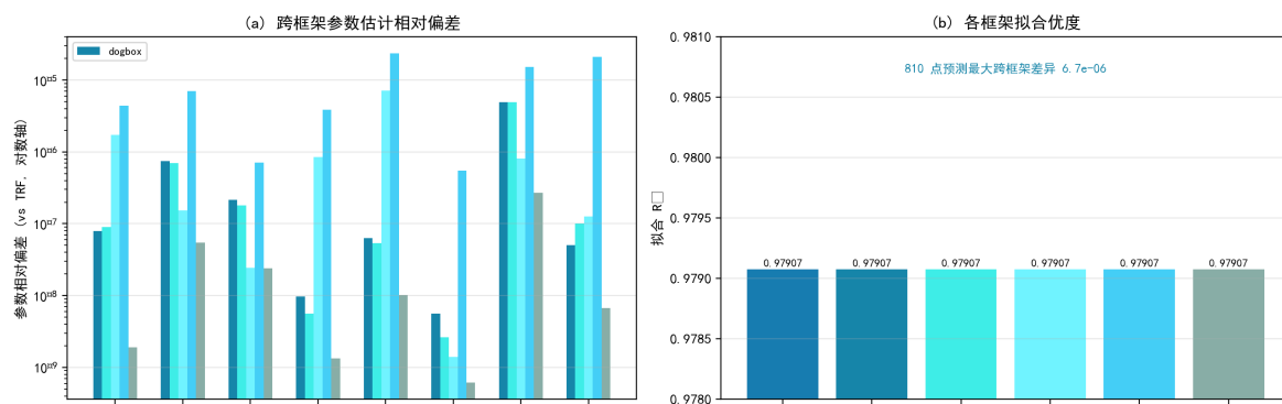
图 6.24 六框架跨框架拟合对比：参数最大相对极差 2.4 \times 10^{-3}\% ，预测差异 6.7 \times 10^{-6} ， R^2 全部为 0.979073。
