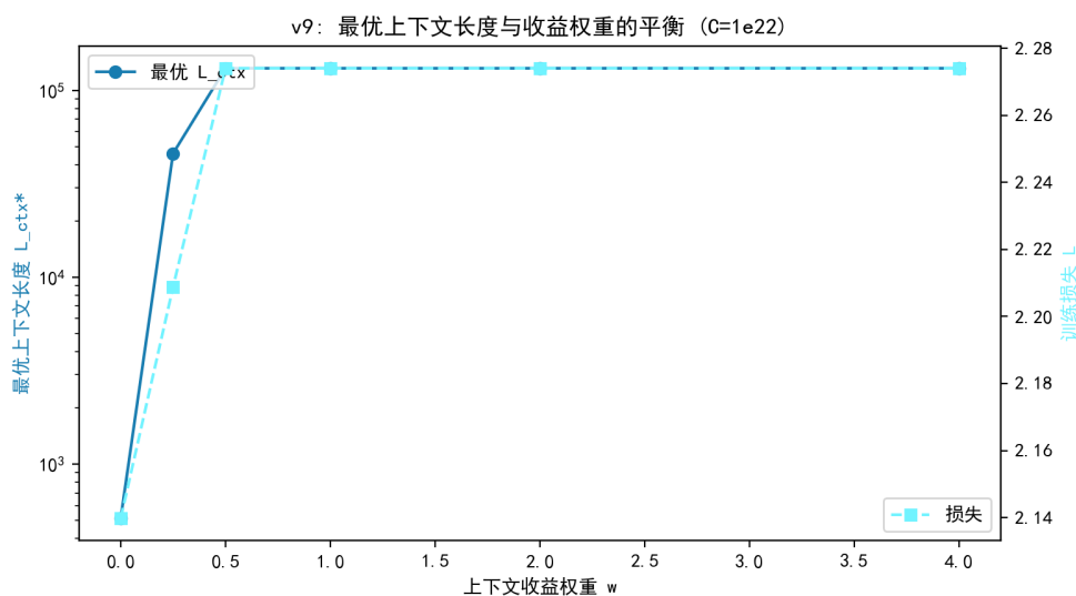
图 7.50 最优上下文长度与收益权重 w 的平衡 ( C = 10^{22} )。
