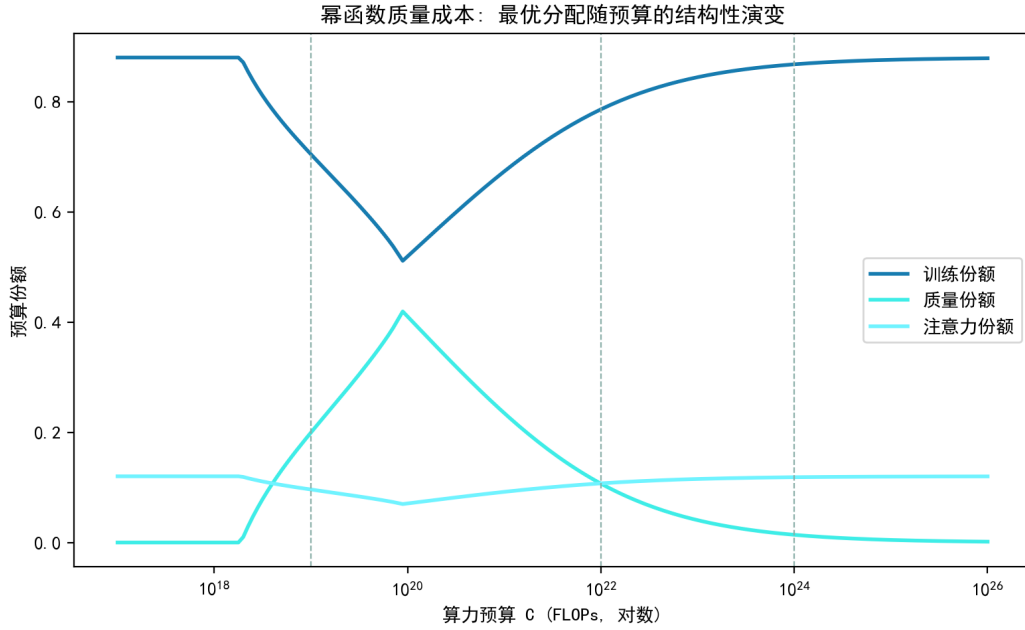
图 7.45 幂函数质量成本下最优成本份额随预算的结构性演变（竖线为三档预算）。
