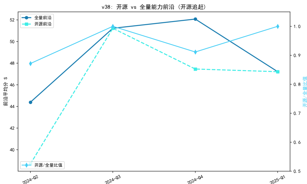
图 8.53 开源 vs 全量能力前沿：开源在 2024Q3/2025Q1 追平全量领跑。
