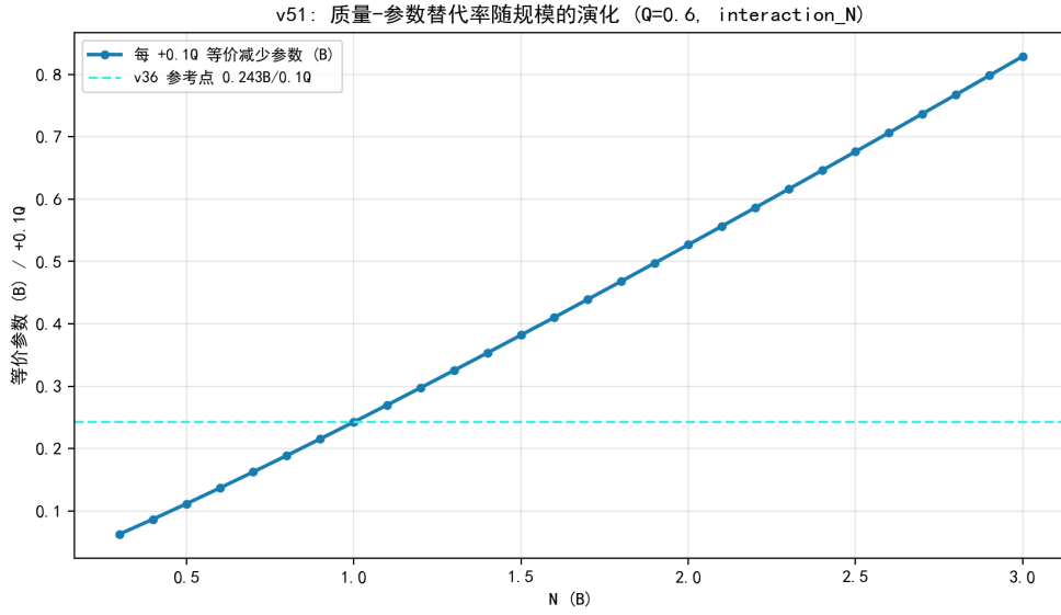
图 6.33 每 +0.1Q 等价减少的参数随规模的演化（近线性上升）。
