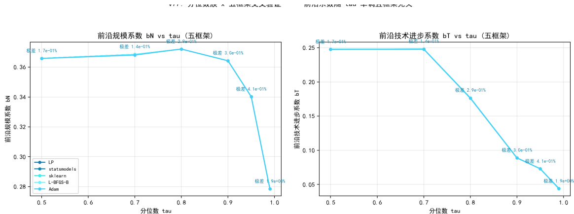
图 8.58 分位数族 \times 五框架：每个 \tau 上五框架一致； b_T 随 \tau 单调递减、 b_N 峰后回落。
