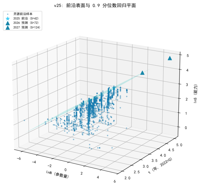
图 8.69 能力前沿 3D 表面与 0.9 分位数回归平面（星标 = 2025 前沿，三角 = 预测点）。
