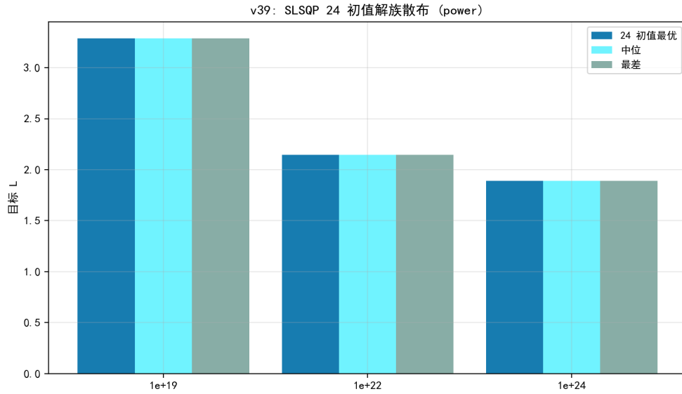
图 7.35 SLSQP 多初值解族散布：三档预算成功收敛初值全部落到同一最优。
