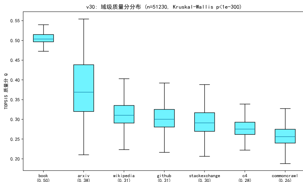
图 5.12 七域样本级质量分分布（箱线图，Kruskal-Wallis p < 10^{-300} ）。
