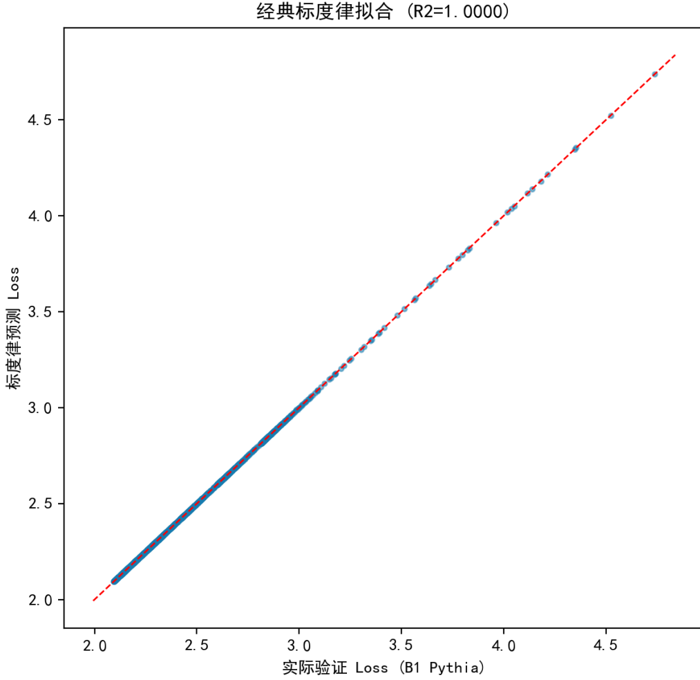
图 6.20 经典标度律在 B1 轨迹上的拟合与跨家族验证。
