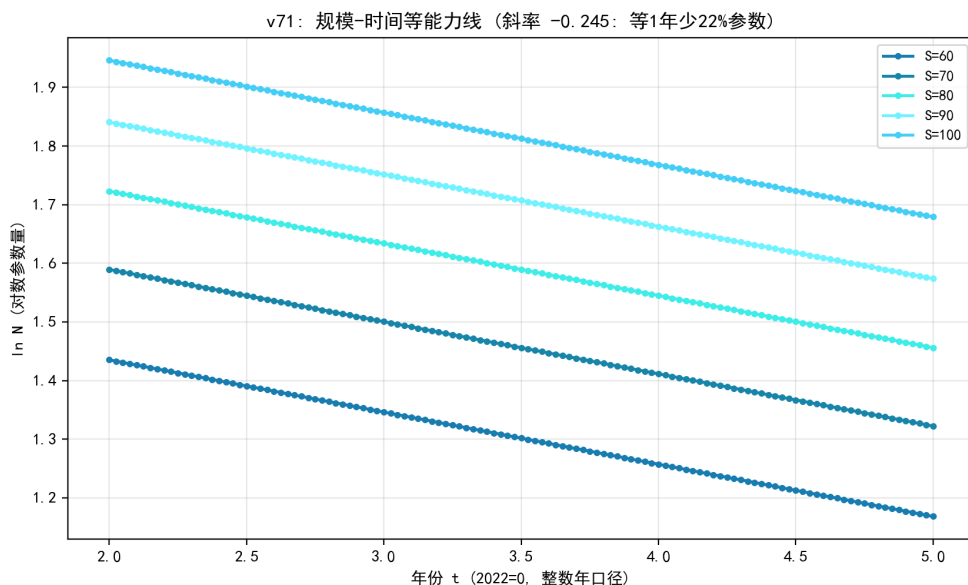
图 8.61 规模-时间等能力线：等 1 年少用 22% 参数（斜率 -0.245）。
