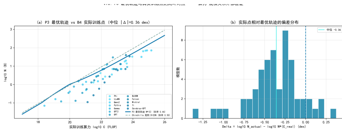
图 7.52 闭环对照：P3 最优轨迹与 B4 实际训练点（左）；偏差分布（右）。中位偏差 0.36 dex，优于 Chinchilla 规则 30%。
