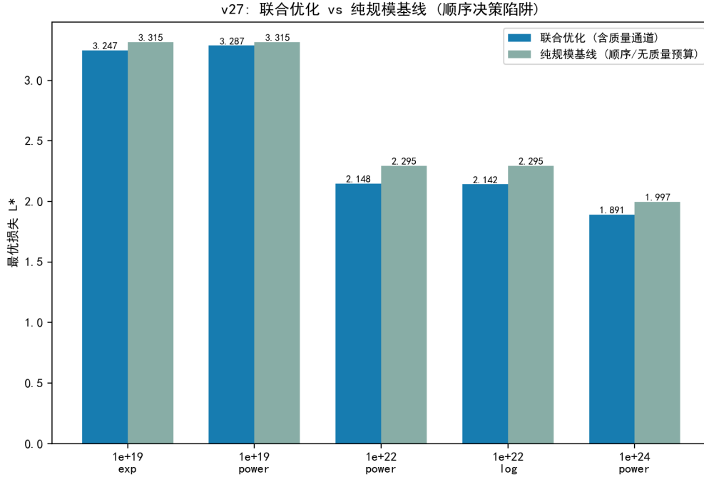
图 7.49 联合优化 vs 纯规模基线的最优损失（顺序决策陷阱：质量需预算预留）。
