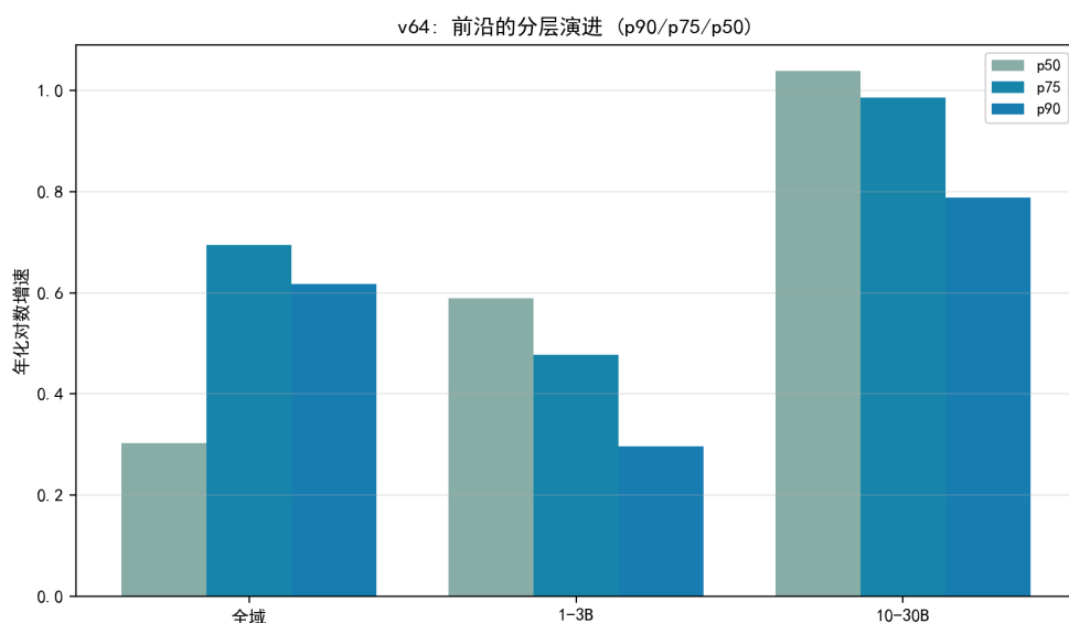
图 8.66 分层演进：全域顶层分化（ p90/p50 \approx 2 ），段内普惠（ p50 快于 p90 ）。
