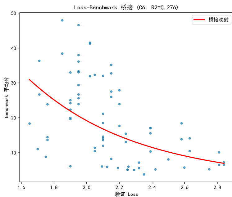
图 8.72 Loss-Benchmark 桥接映射 (C6, 75 个模型)。
