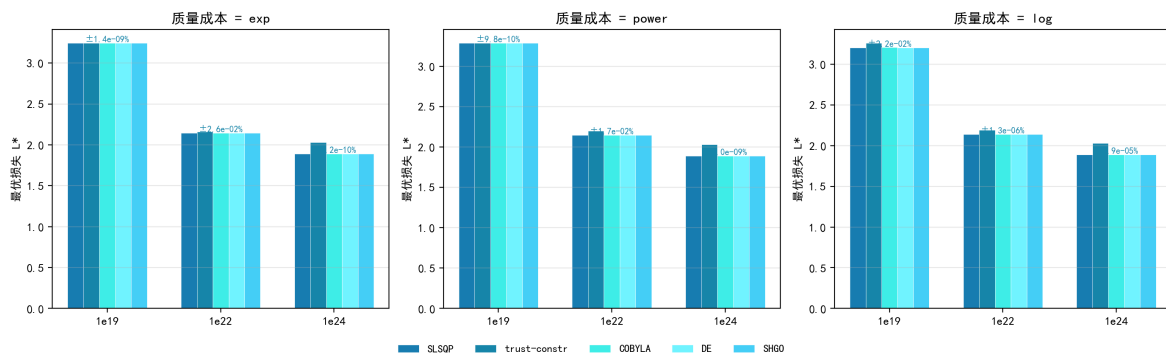
图 7.36 五框架求解对比：SLSQP/COBYLA/DE/SHGO 在 9 实例上一致到 10^{-6} 量级（括号为四框架最大相对偏差），trust-constr 内点法在边界角点最优处失稳。
