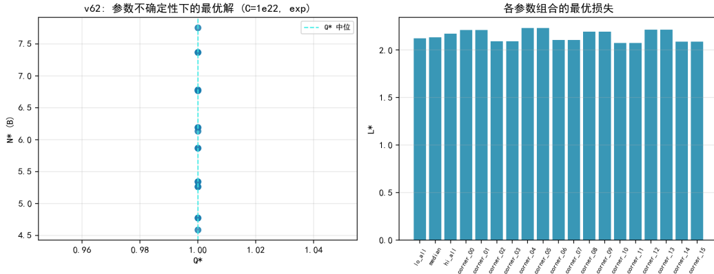
图 7.40 参数角点下的最优解： Q^*=1 稳定、 L^* 带宽 \pm 3.5\% 、 N^* \pm 28\% 。
