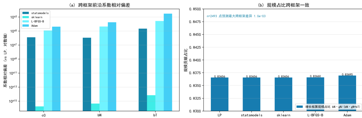
图 8.57 五框架分位数回归交叉验证：系数与规模贡献占比（83.7%）跨框架一致。
