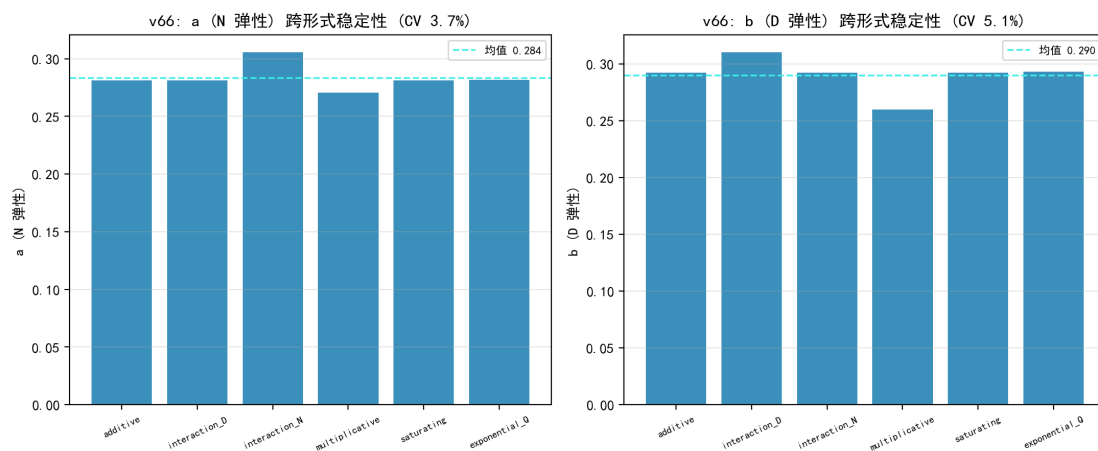
图 6.25 六形式共享参数：a/b 跨形式稳定 (CV<6%)、 (1-Q)^g 族 g \approx 1 。
