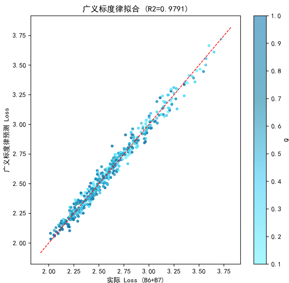
图 6.26 广义标度律在 B6+B7 数据上的拟合（质量-参数量交互形式， R^2 = 0.979 ）。
