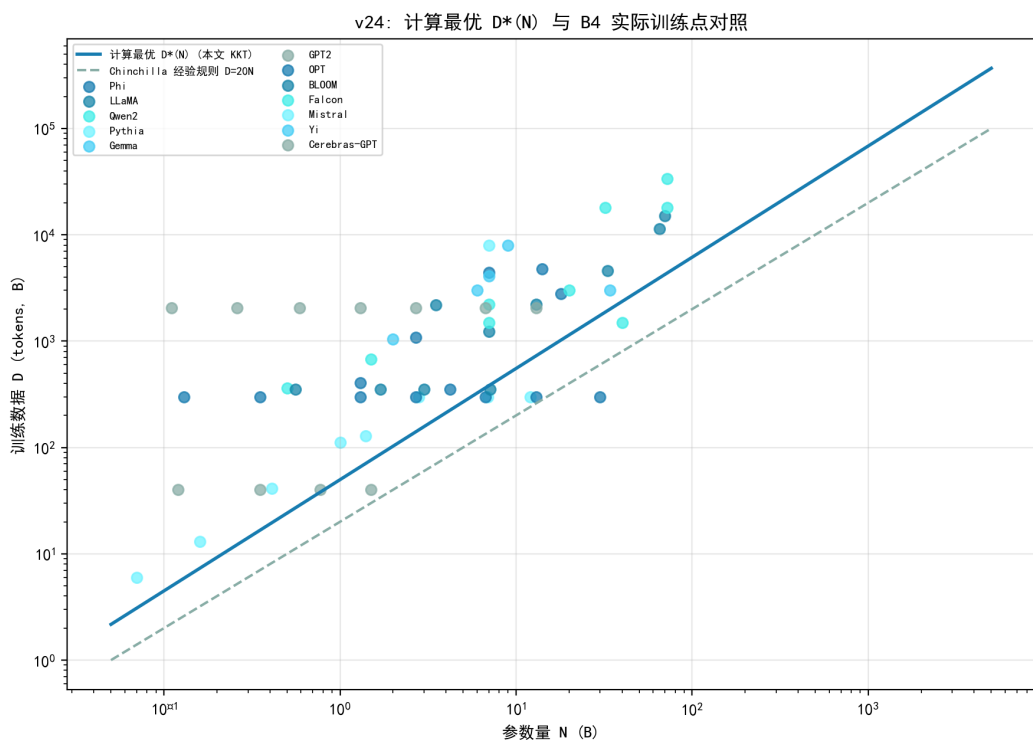
图 7.42 计算最优数据曲线 D^*(N) 、Chinchilla 经验规则与 B4 实际训练点。
