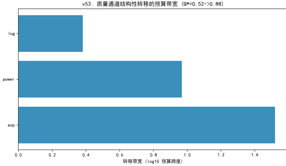
图 7.44 质量通道结构性转移的预算带宽 ( Q^* = 0.52 \rightarrow 0.88 )。
