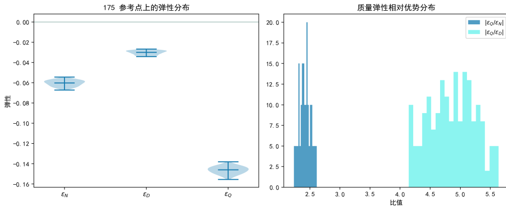
图 6.34 175 个参考点上弹性分布与质量弹性相对优势比值。
