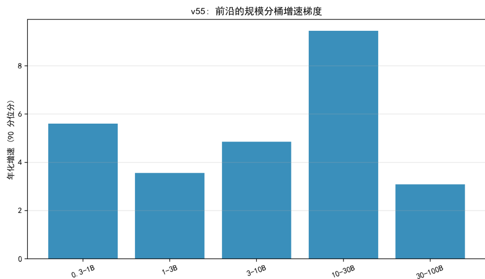
图 8.64 规模分桶的前沿年化增速：10-30B 甜点区最快，30-100B 最慢。
