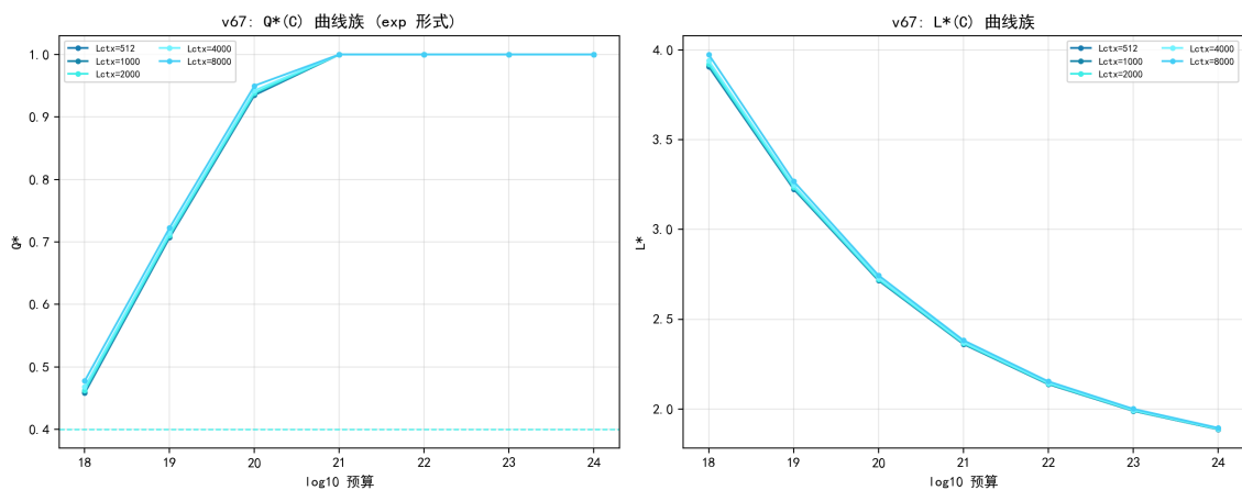
图 7.41 上下文长度 \times 预算响应面： L^* 路径几乎不随 L_{ctx} 移动。
