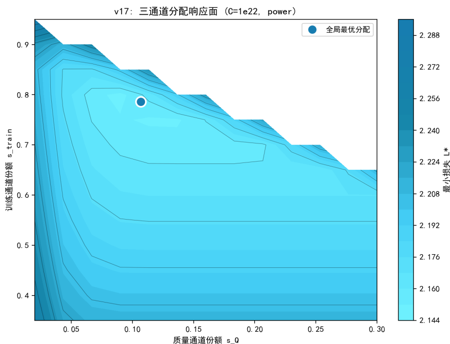
图 7.51 三通道分配响应面 ( C = 10^{22} , 幂成本; 蓝点为全局最优分配)。
