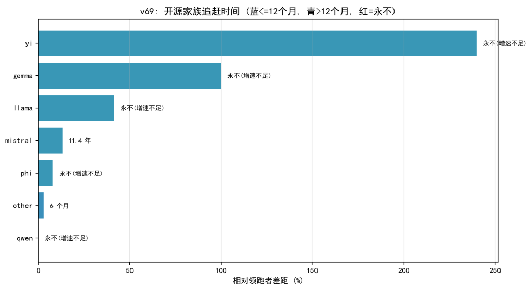
图 8.56 家族追赶时间：仅 other 可短期追平，Llama 近乎停滞。
