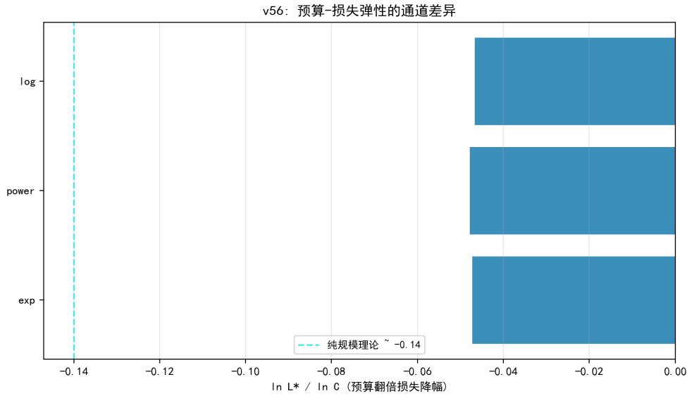
图 7.39 总损失口径的预算弹性：三形式几乎重合，低于超额口径斜率。
