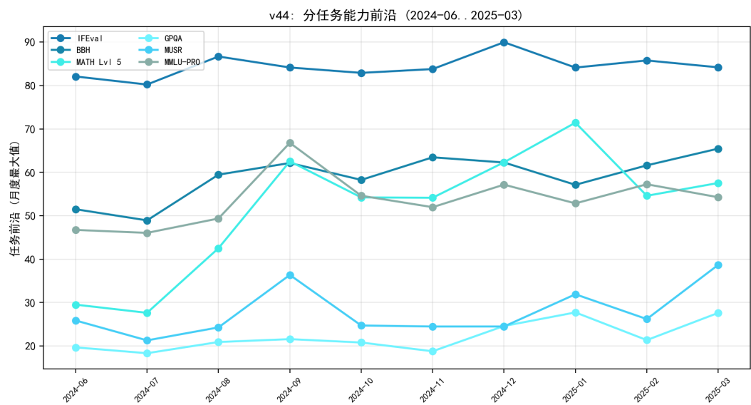
图 8.63 分任务能力前沿：推理类（MATH/GPQA/MUSR）增长快于知识/指令类。
