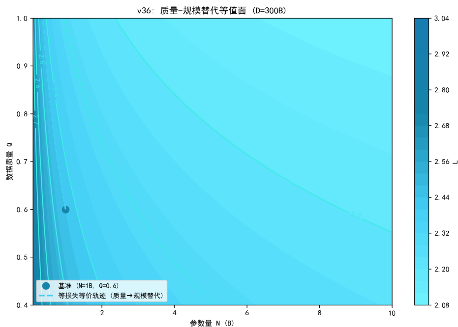
图 6.32 质量-规模替代等值面：等损失轨迹显示质量对参数的替代关系。
