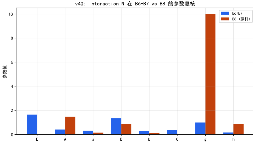
图 6.23 B8 原样 vs B6+B7 的参数对比：B8 质量项退化 ( E = C = 0 , g 撞界)。
