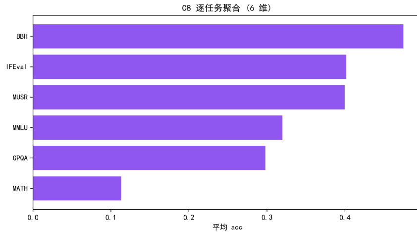
图 8.57 C8 逐任务聚合得分（6 维）。
