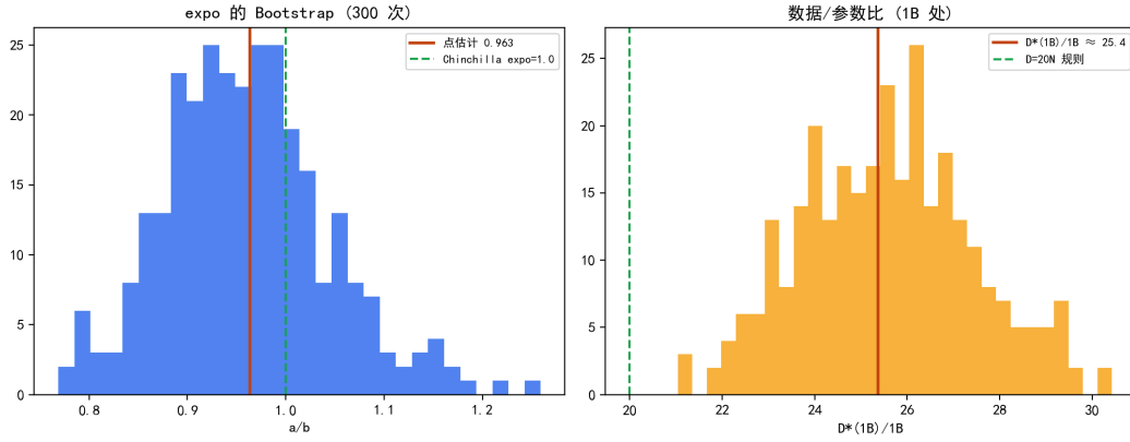
图 7.35 D^*(N) 参数 Bootstrap: 指数 CI 含 1.0, 常数 CI 高于 D = 20N 。
