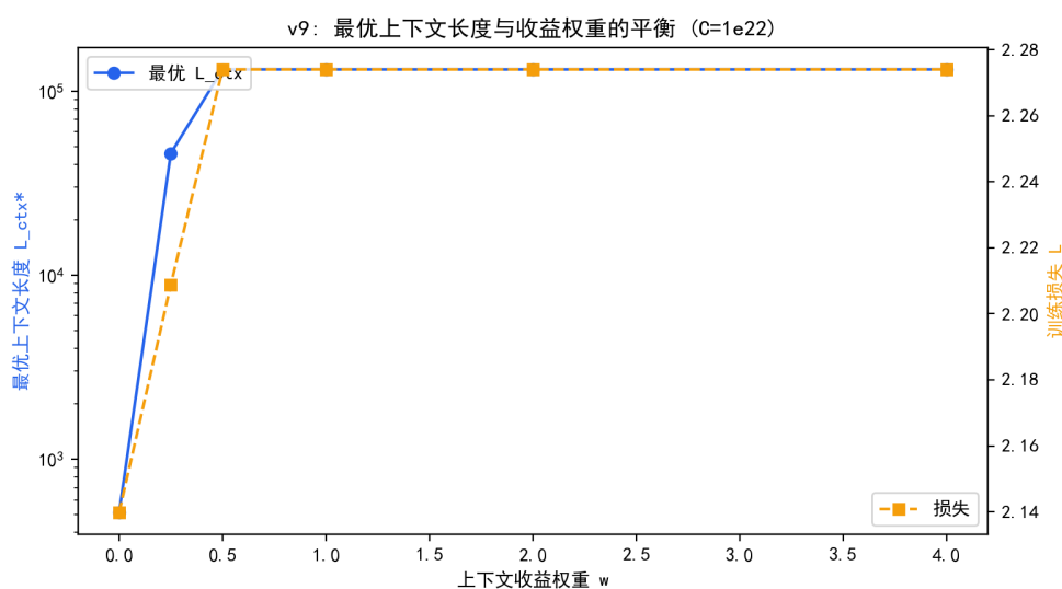
图 7.42 最优上下文长度与收益权重 w 的平衡（ C = 10^{22} ）。
