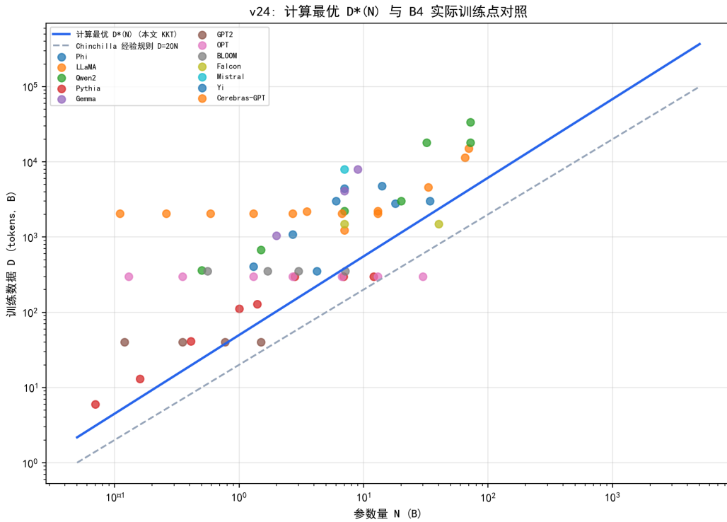
图 7.34 计算最优数据曲线 D^*(N) 、Chinchilla 经验规则与 B4 实际训练点。
