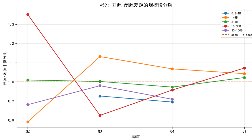
图 8.45 开源-闭源差距的规模段分解：中段持平、两端滞后约 10%。
