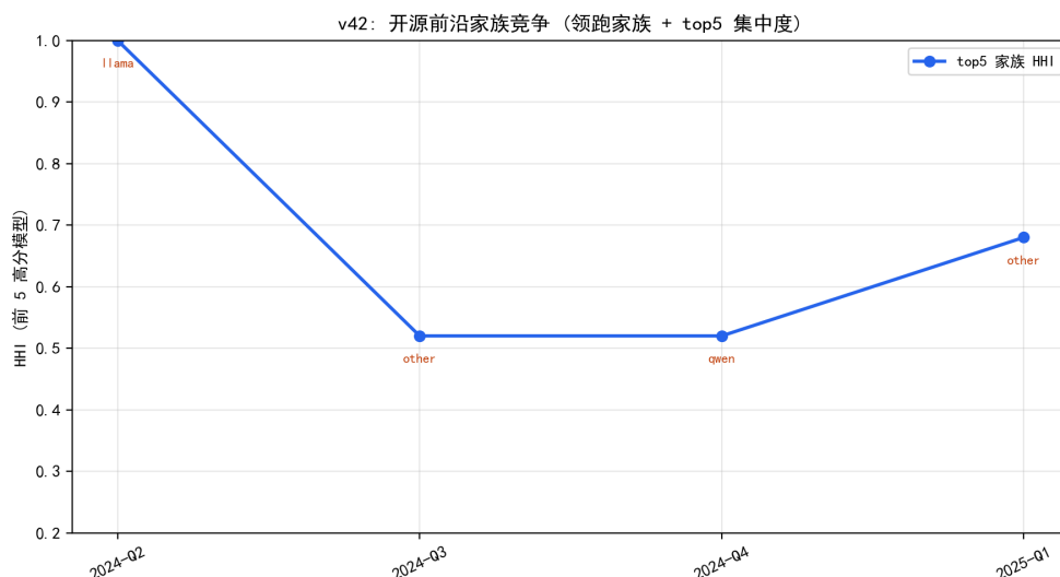
图 8.46 开源前沿家族竞争：领跑家族轮替与 top5 集中度（HHI）。
