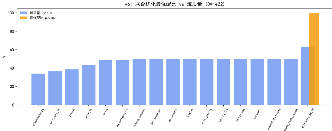
图 7.40 联合优化最优配比与域质量对比（ C = 10^{22} ）：配比向最高质量域（小说）集中。
