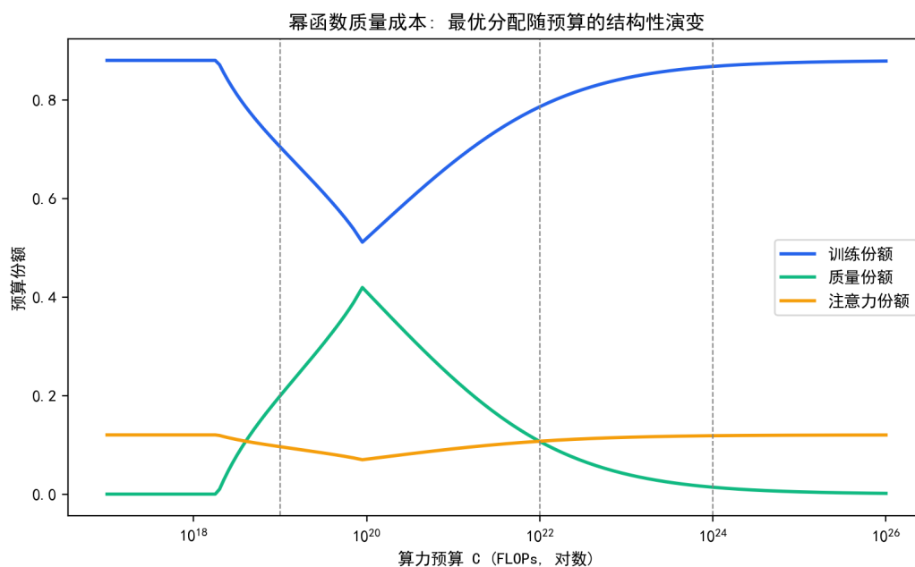
图 7.37 幂函数质量成本下最优成本份额随预算的结构性演变（竖线为三档预算）。
