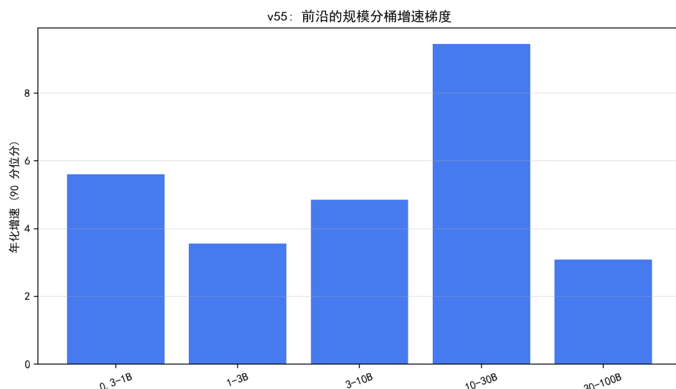
图 8.50 规模分桶的前沿年化增速：10–30B 甜点区最快，30–100B 最慢。
