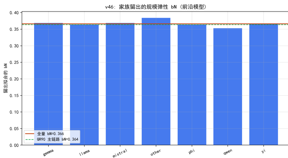
图 8.54 家族留下的规模弹性 b_N ：全家族稳定在 0.36 附近。
