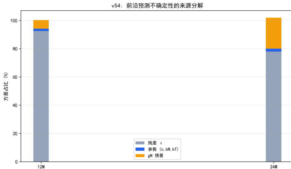
图 8.47 前沿预测不确定性的来源分解（12M/24M）。
