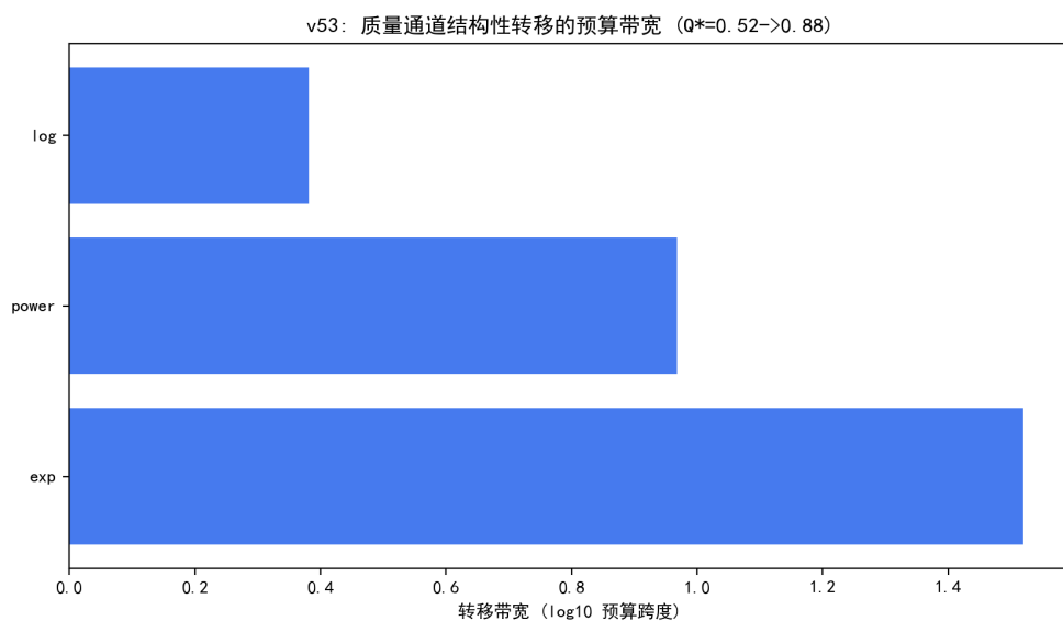
图 7.36 质量通道结构性转移的预算带宽 ( Q^* = 0.52 \rightarrow 0.88 )。
