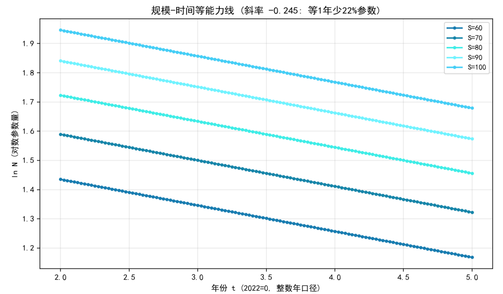
图 8.63 规模–时间等能力线： 等 1 年少用 22% 参数（斜率 -0.245 ）。
