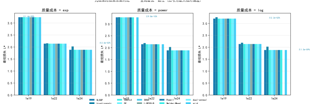
图 7.38 九框架求解对比：SLSQP/COBYLA/DE/SHGO/L-BFGS-B/Powell/Nelder-Mead/ 双退火/网格在 9 实例上一致到 10^{-6} 量级（括号为九路径最大相对偏差），trust-constr 内点法在边界角点最优处失稳。
