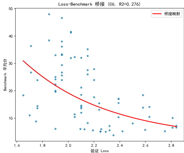
图 8.74 Loss-Benchmark 桥接映射（C6，75 个模型）。
