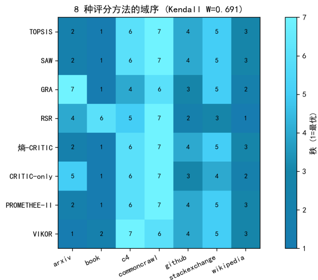
图 5.1 八种评分方法的七域域序（加权/折衷五方法高度一致，秩法偏离）。
