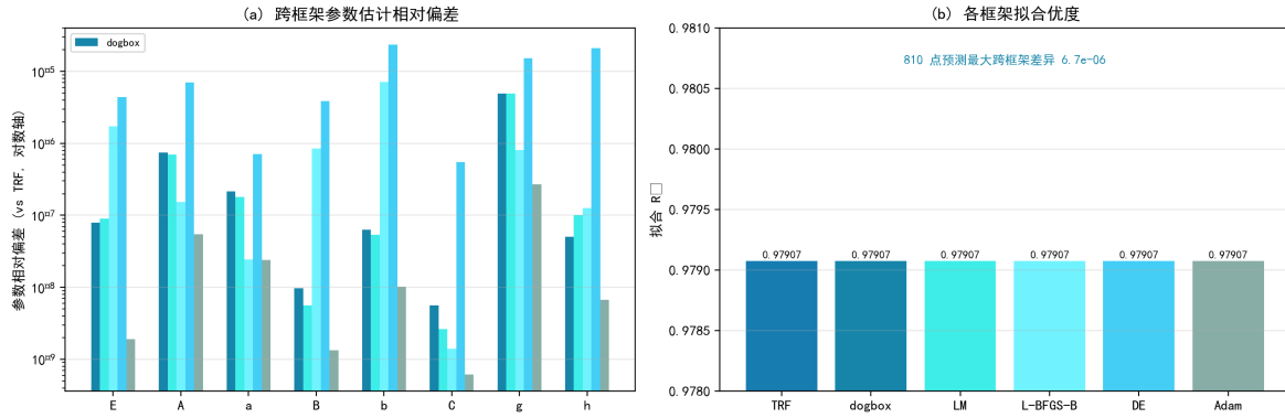
图 6.26 六框架跨框架拟合对比：参数最大相对极差 2.4 \times 10^{-3}\% ，预测差异 6.7 \times 10^{-6} ， R^2 全部为 0.979073。
