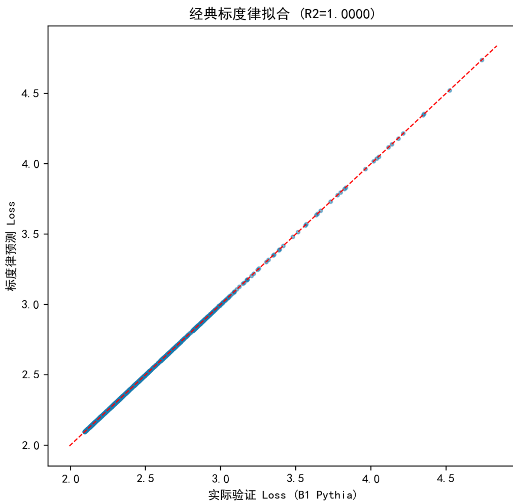
图 6.21 经典标度律在 B1 轨迹上的拟合与跨家族验证。
