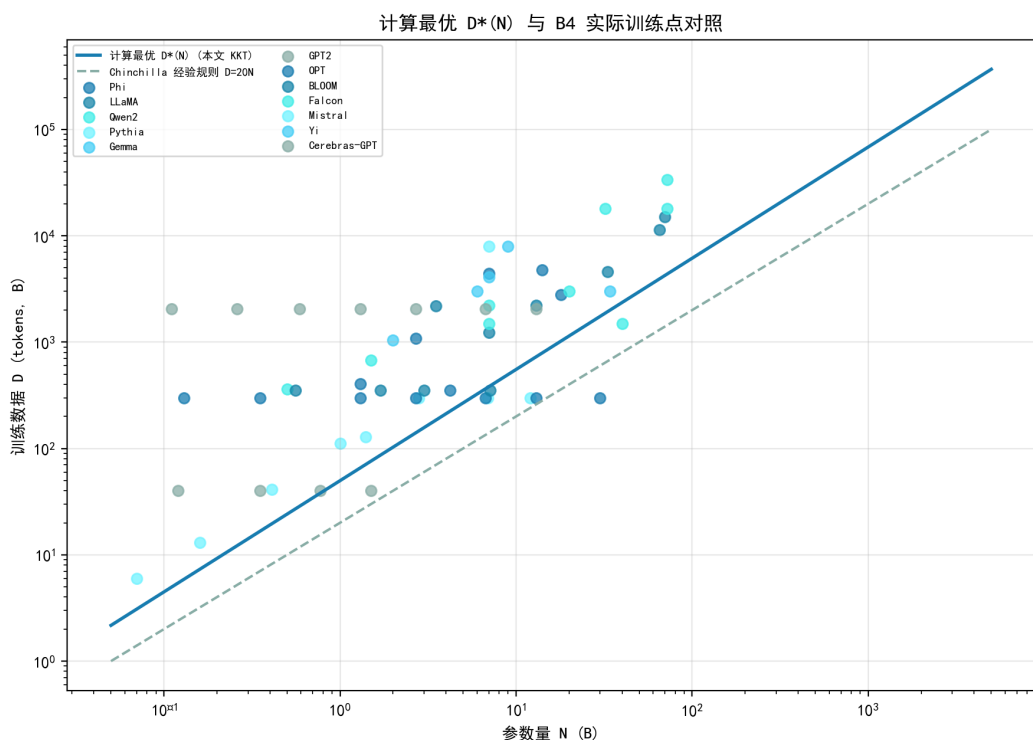
图 7.44 计算最优数据曲线 D^*(N) 、Chinchilla 经验规则与 B4 实际训练点。
