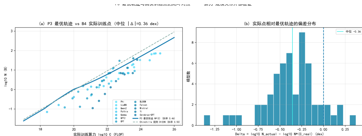
图 7.54 闭环对照: P3 最优轨迹与 B4 实际训练点 (左); 偏差分布 (右)。中位偏差 0.36 \text{ dex} , 优于 Chinchilla 规则 30%。
