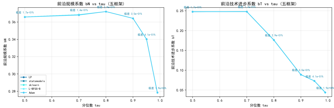
图 8.60 分位数族 \times 五框架：每个 \tau 上五框架一致； b_T 随 \tau 单调递减、 b_N 峰后回落。
