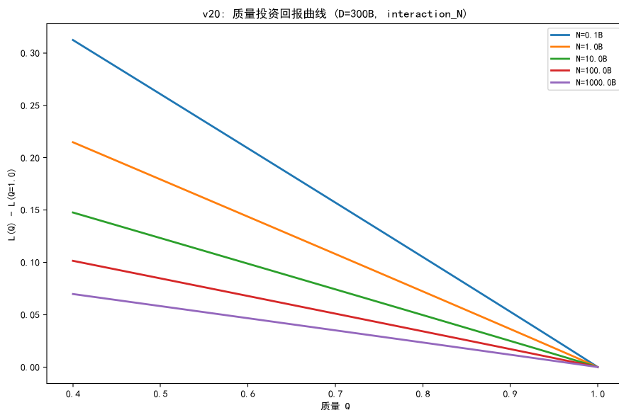
图 6.22 质量投资回报曲线 ( D = 300B ): L(Q) 相对 L(Q = 1) 随 N 变化。
