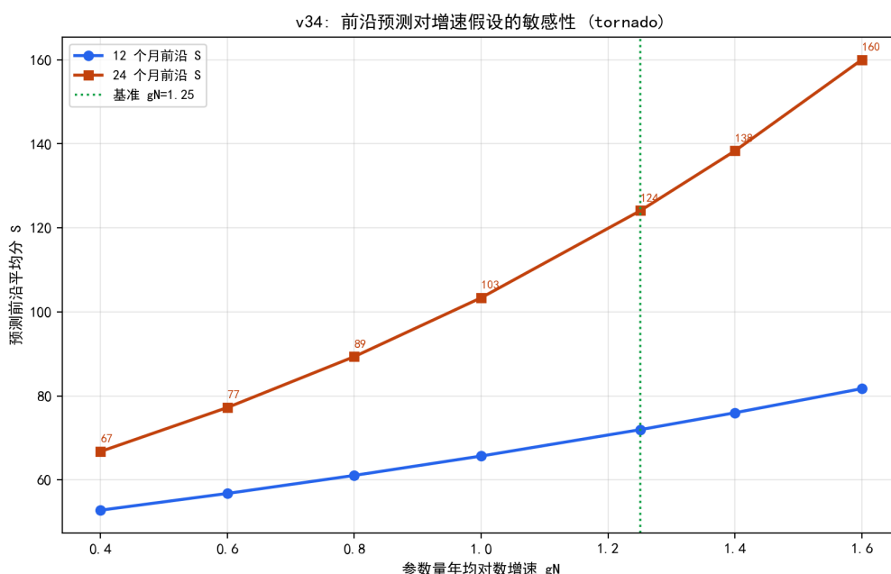
图 8.44 前沿预测对参数量增速假设 g_N 的敏感性（12/24 个月）。
