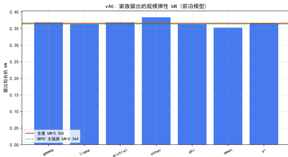
图 8.50 家族留下的规模弹性 b_N ：全家族稳定在 0.36 附近。
