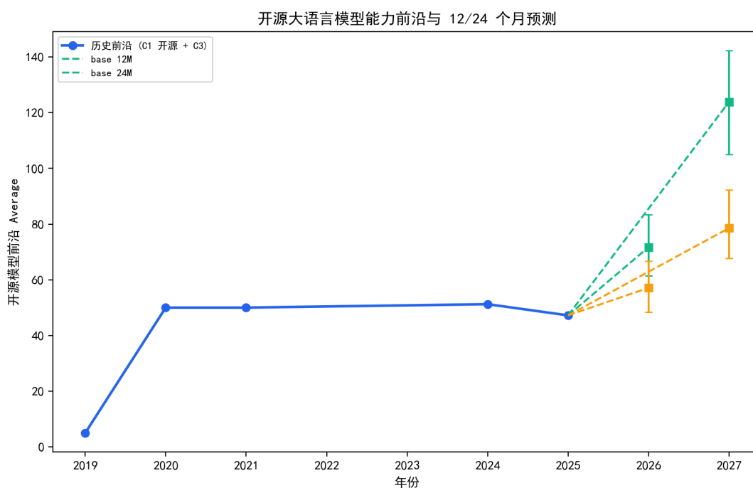
图 8.48 开源模型能力前沿（历史点）与 12/24 个月预测（基础/放缓情景，90% 区间）。
