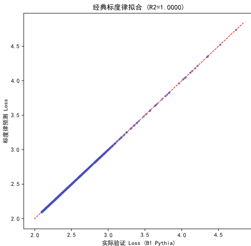
图 6.15 经典标度律在 B1 轨迹上的拟合与跨家族验证。
