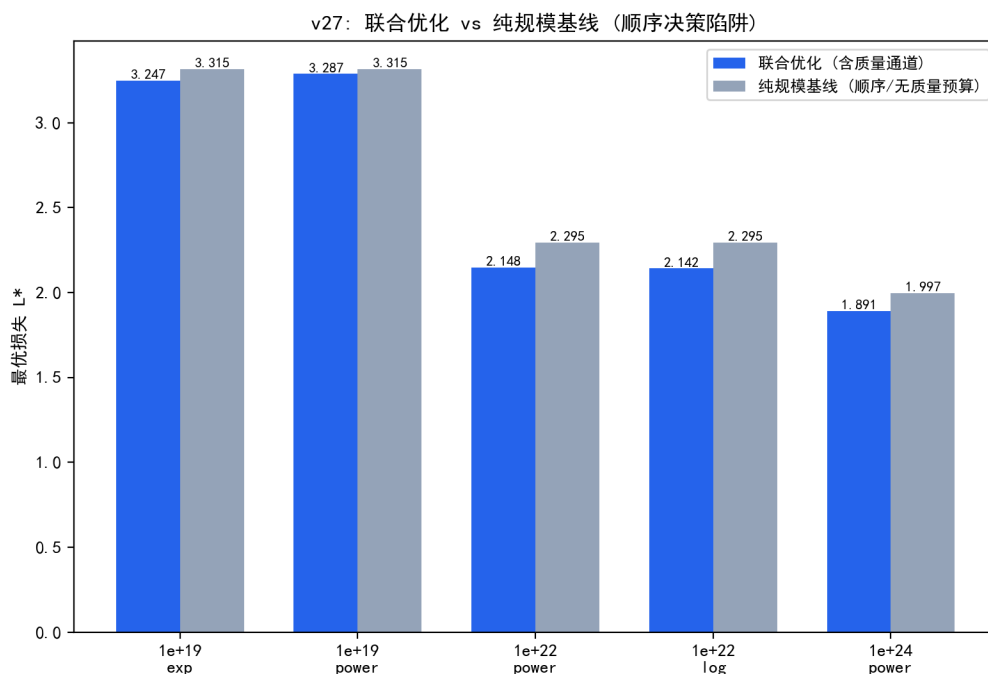
图 7.38 联合优化 vs 纯规模基线的最优损失（顺序决策陷阱：质量需预算预留）。
