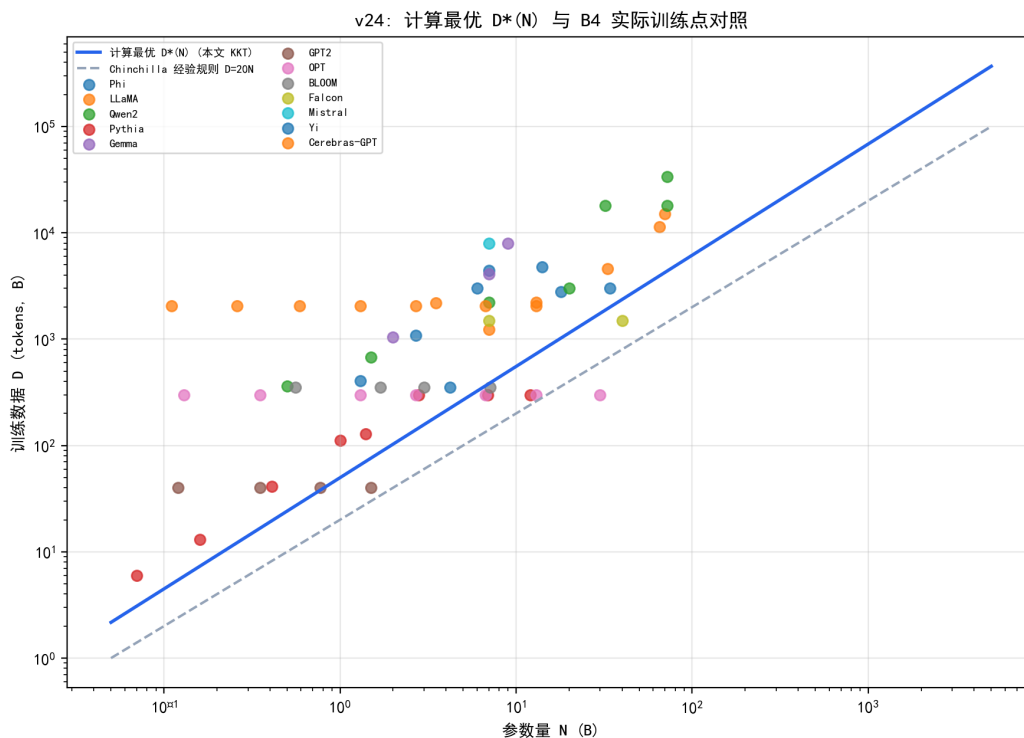
图 7.31 计算最优数据曲线 D^*(N) 、Chinchilla 经验规则与 B4 实际训练点。
