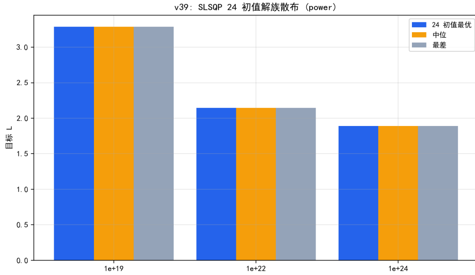
图 7.27 SLSQP 24 初值解族散布：三档预算全部初值收敛到同一最优。
