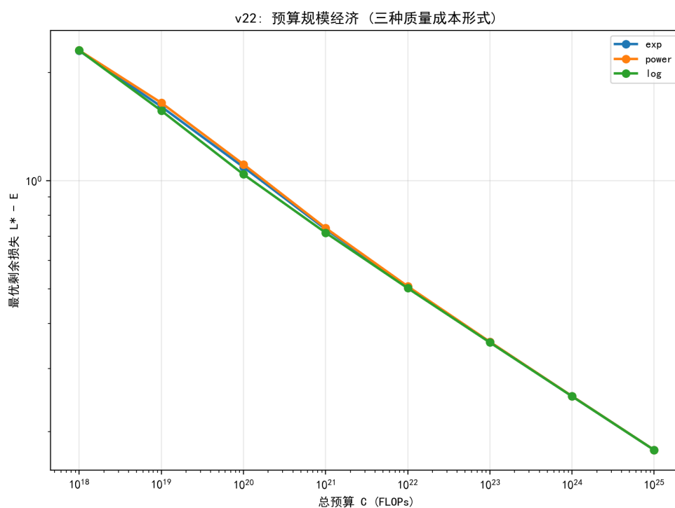
图 7.29 预算-最优损失的对数线性规律（三种质量成本形式）。
