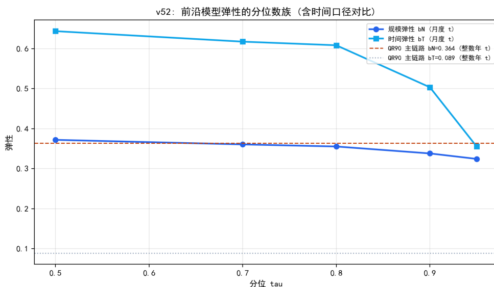
图 9.54 前沿弹性的分位数族与时间口径对比（ b_N 稳健， b_T 对口径敏感）。
