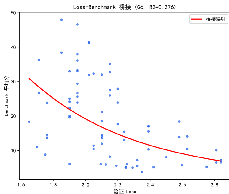
图 8.52 Loss-Benchmark 桥接映射（C6，75 个模型）。
