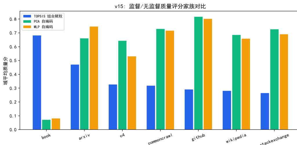
图 9.56 TOPSIS 组合赋权与自编码典型性评分的域级对照（方向相反）。
