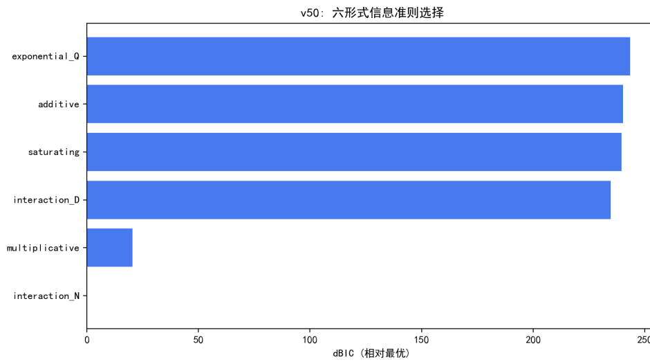
图 6.17 六种形式的 BIC/AIC 选择：interaction_N 决定性胜出。
