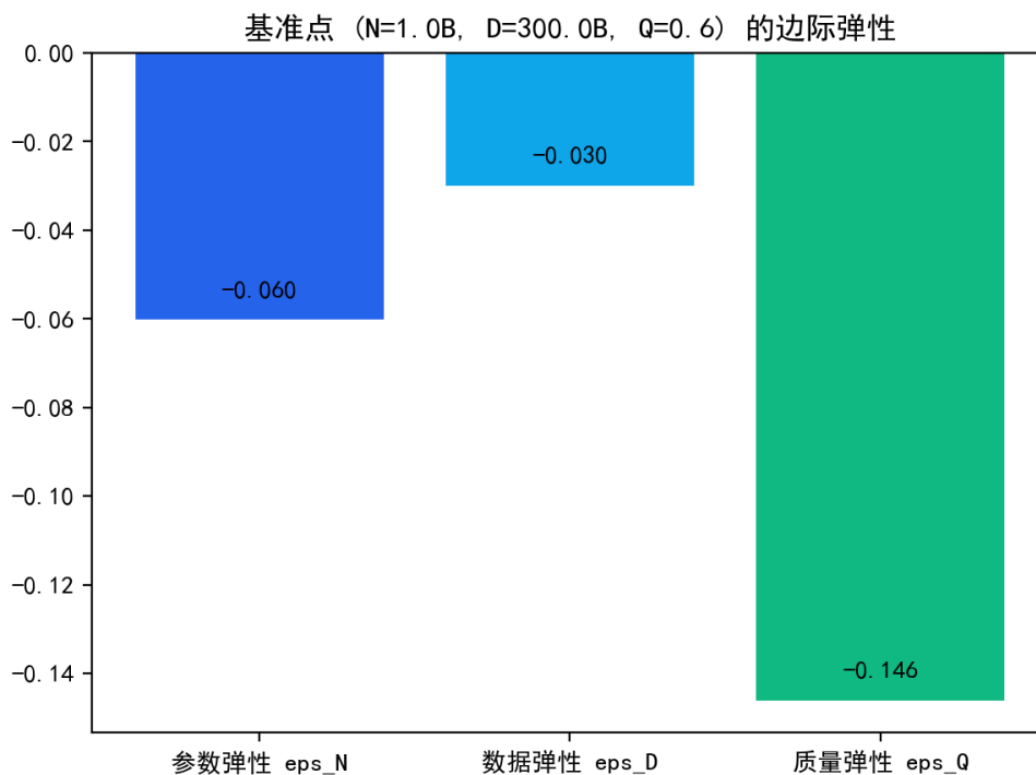
图 6.23 基准点处三个维度的损失弹性对比（质量弹性最高）。
