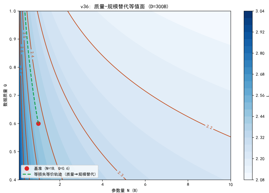
图 6.24 质量-规模替代等值面：等损失轨迹显示质量对参数的替代关系。
