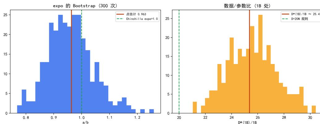
图 7.32 D^*(N) 参数 Bootstrap: 指数 CI 含 1.0, 常数 CI 高于 D = 20N 。
