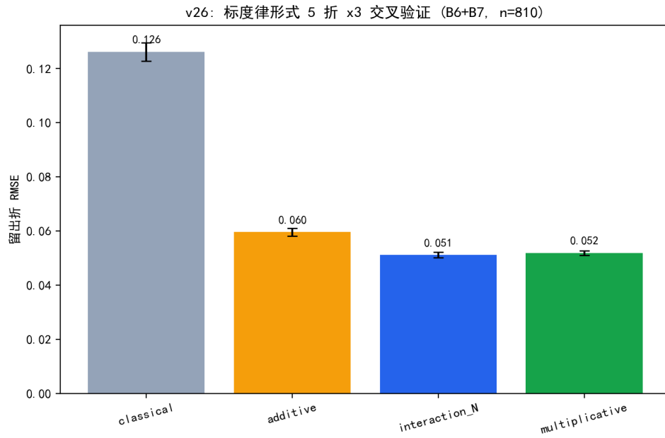
图 6.16 标度律形式 5 折交叉验证的留出 RMSE 对比。
