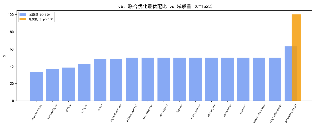
图 7.29 联合优化最优配比与域质量对比（ C = 10^{22} ）：配比向最高质量域（小说）集中。
