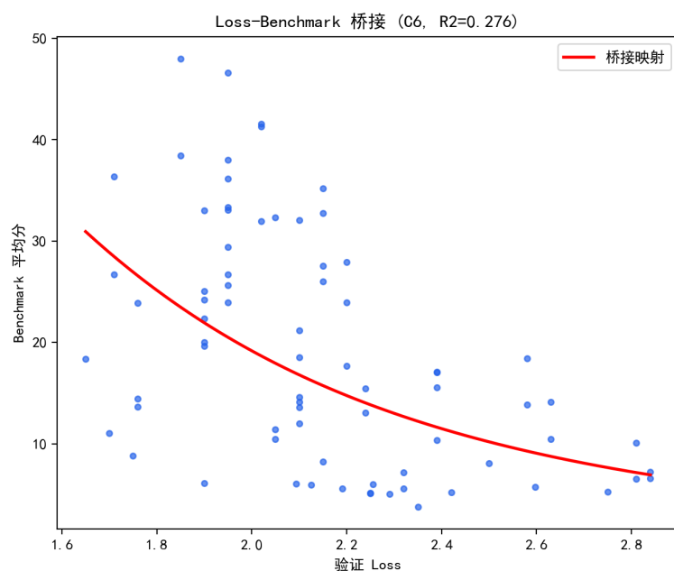
图 8.41 Loss-Benchmark 桥接映射（C6，75 个模型）。
