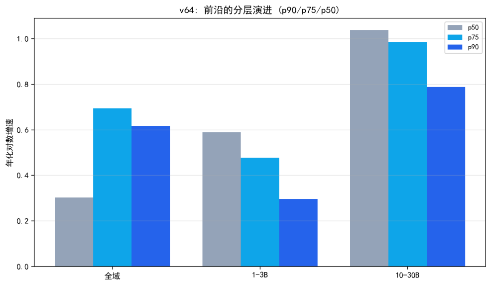
图 8.57 分层演进：全域顶层分化（p90/p50≈2），段内普惠（p50 快于 p90）。
