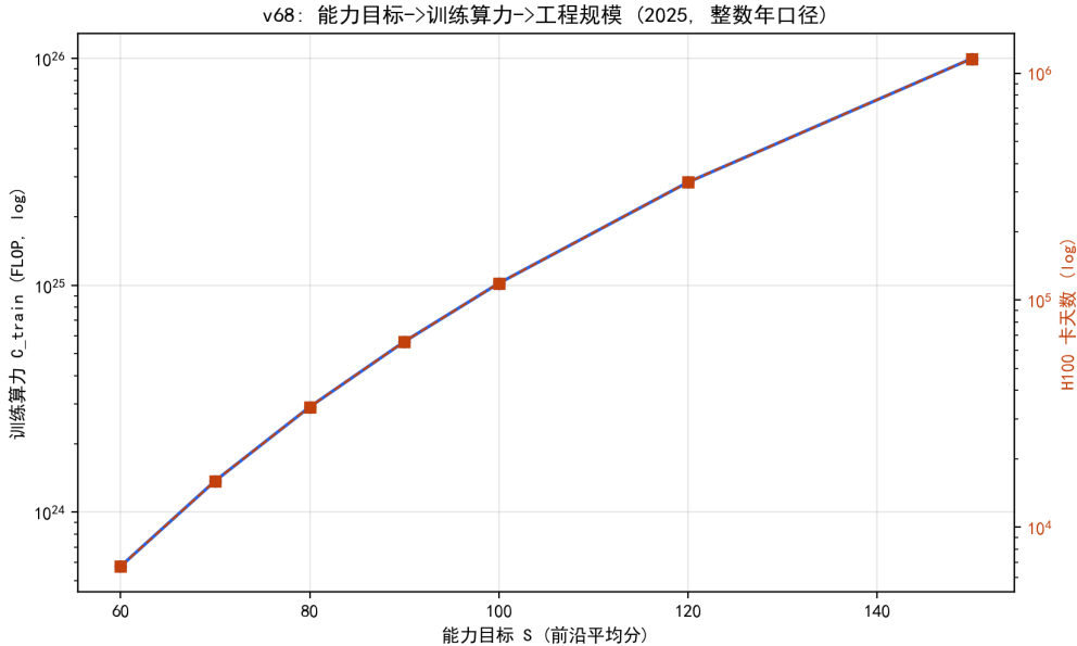
图 8.52 能力目标 → 训练算力（对数轴）： S=90 约需 6.6 万卡天。
