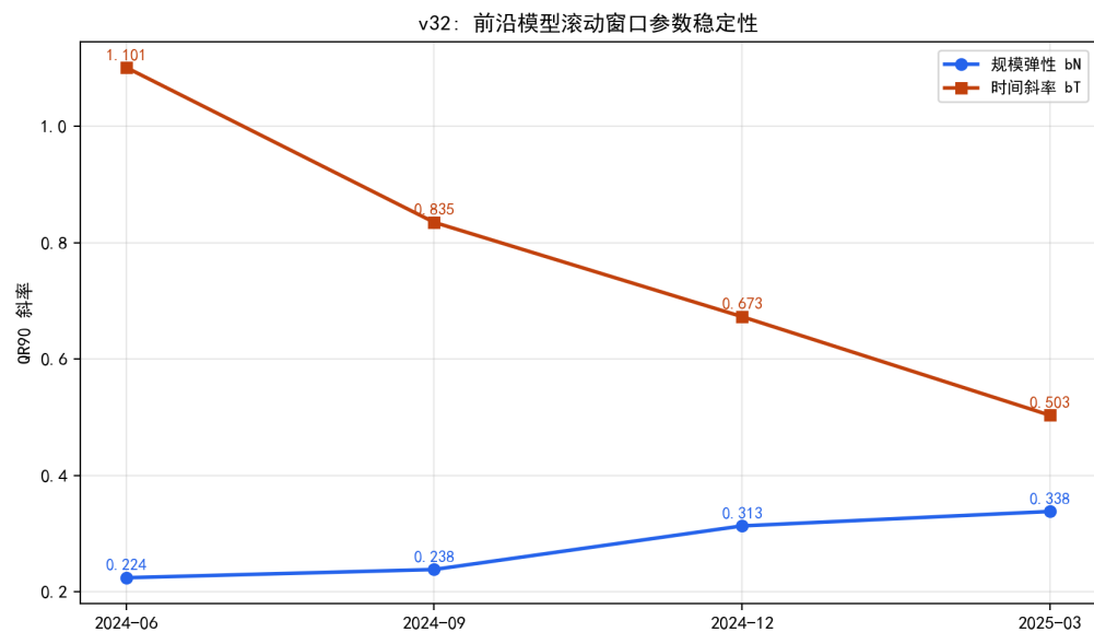
图 8.58 前沿 QR90 滚动窗口参数：规模弹性上升、时间斜率持续下降。
