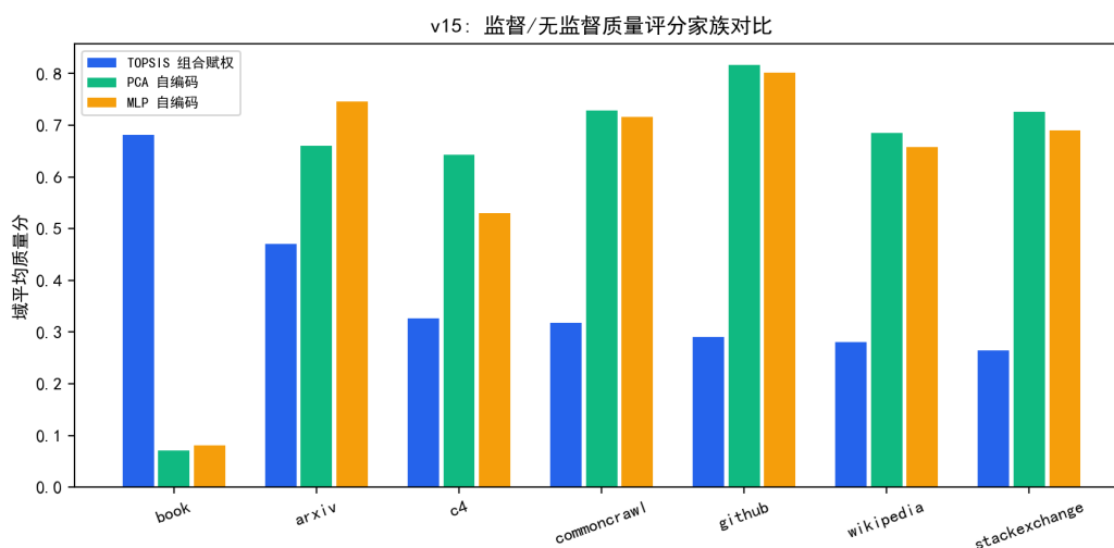
图 9.67 TOPSIS 组合赋权与自编码典型性评分的域级对照（方向相反）。
