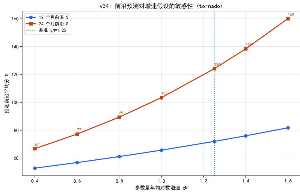
图 8.53 前沿预测对参数量增速假设 g_N 的敏感性（12/24 个月）。
