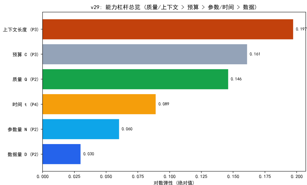
图 10.68 能力杠杆总览：各投入的对数弹性排序（质量/上下文 > 预算 > 参数/时间 > 数据）。
