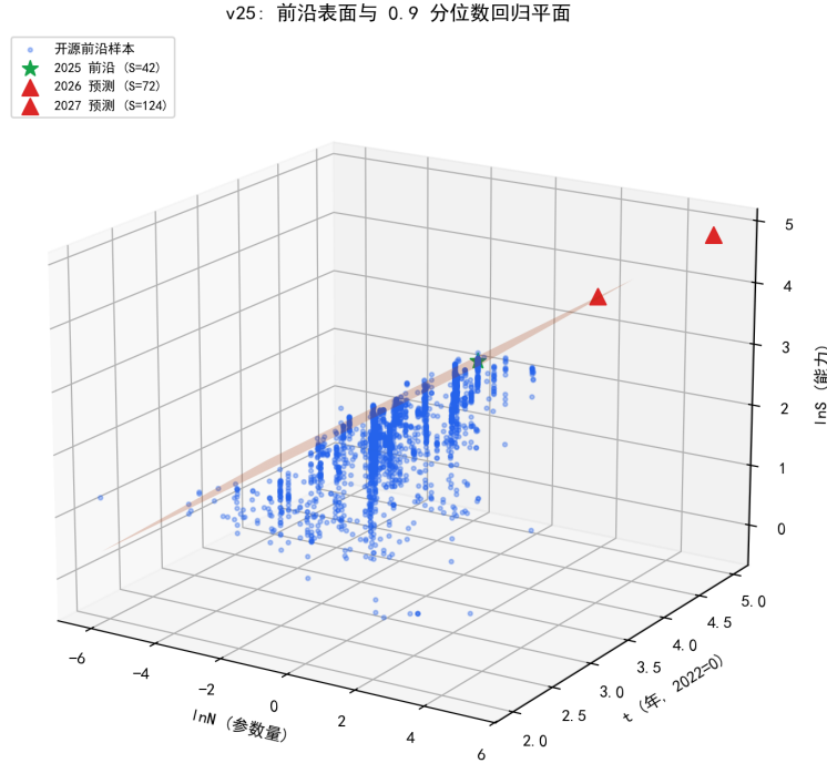
图 8.60 能力前沿 3D 表面与 0.9 分位数回归平面（星标 = 2025 前沿，三角 = 预测点）。
