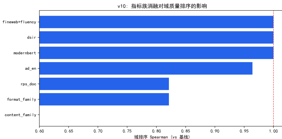
图 9.66 指标族消融对域质量排序的影响（红虚线为完全一致）。
