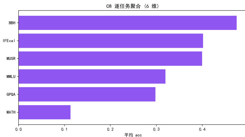
图 8.64 C8 逐任务聚合得分 (6 维)。
