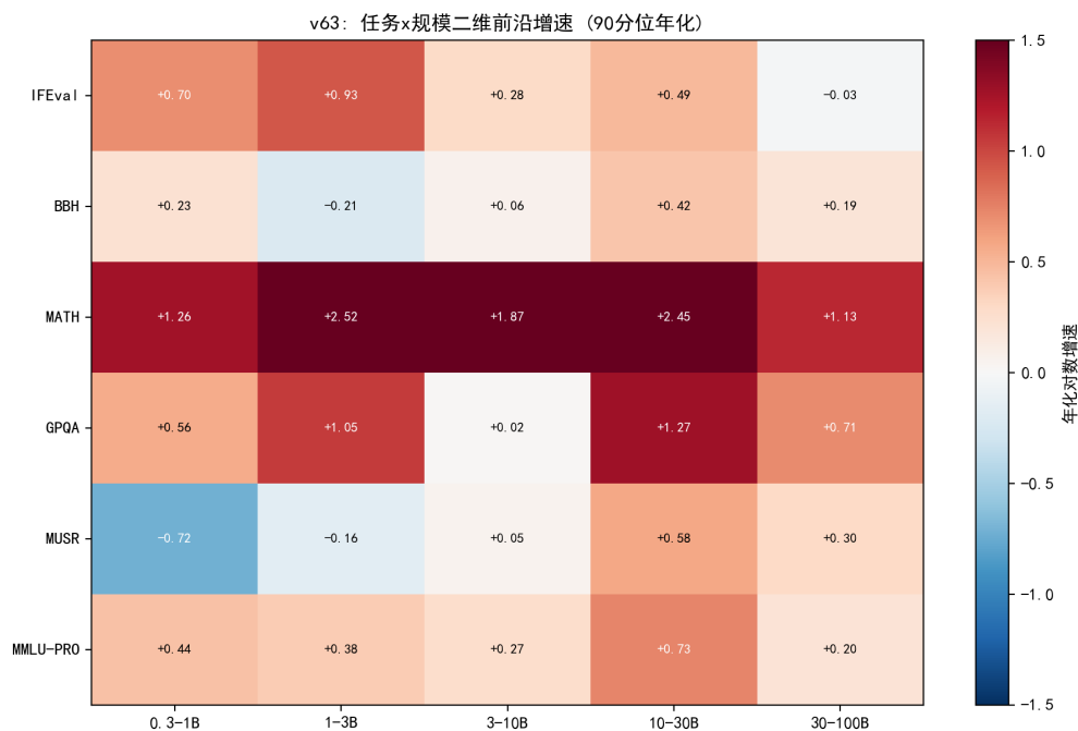
图 8.56 任务 × 规模二维前沿增速：MATH/GPQA 在 1-3B 与 10-30B 双峰。
