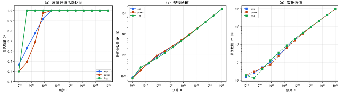
图 7.23 最优解族随预算轨迹：质量通道活跃区间由成本形式决定。
