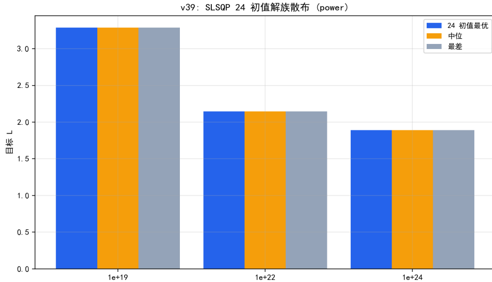
图 7.18 SLSQP 24 初值解族散布：三档预算全部初值收敛到同一最优。
