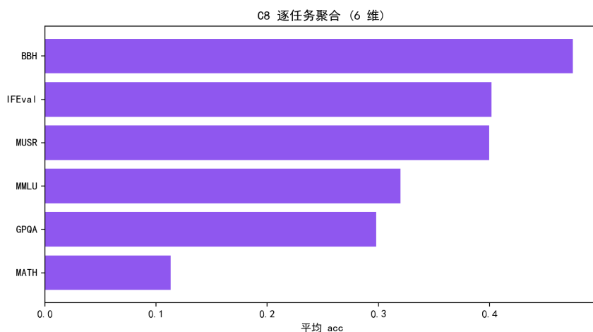
图 8.36 C8 逐任务聚合得分（6 维）。
