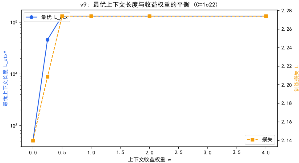
图 7.27 最优上下文长度与收益权重 w 的平衡 ( C = 10^{22} )。
