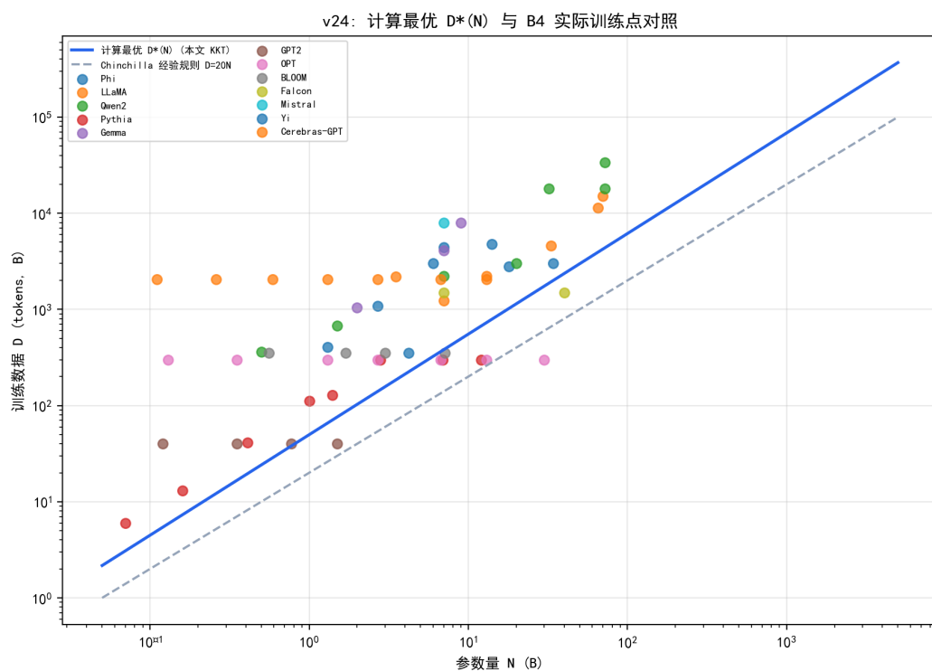
图 7.21 计算最优数据曲线 D^*(N) 、Chinchilla 经验规则与 B4 实际训练点。
