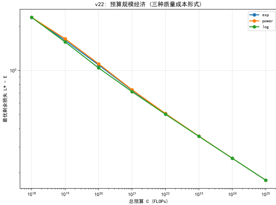
图 7.20 预算-最优损失的对数线性规律（三种质量成本形式）。
