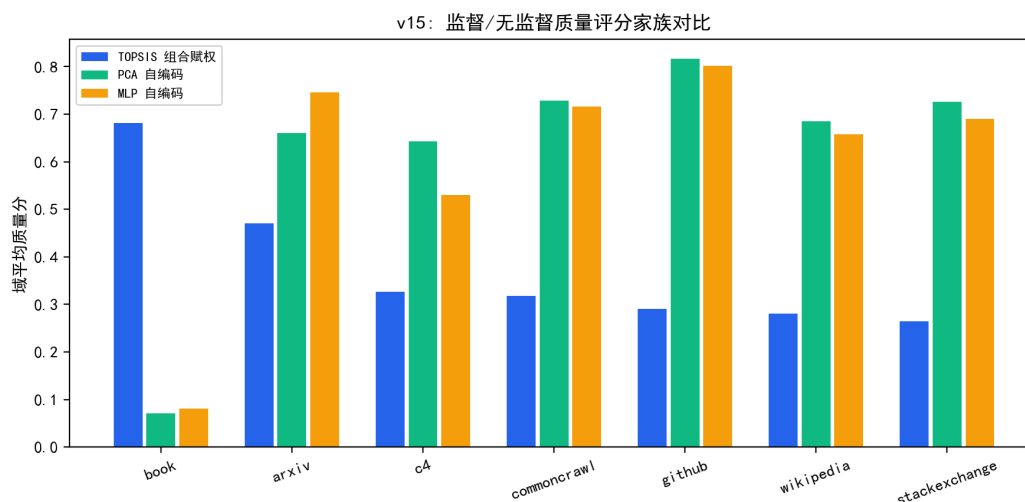
图 9.66 TOPSIS 组合赋权与自编码典型性评分的域级对照（方向相反）。
