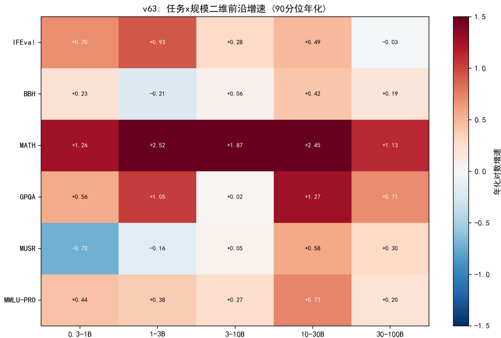
图 8.55 任务 × 规模二维前沿增速：MATH/GPQA 在 1-3B 与 10-30B 双峰。
