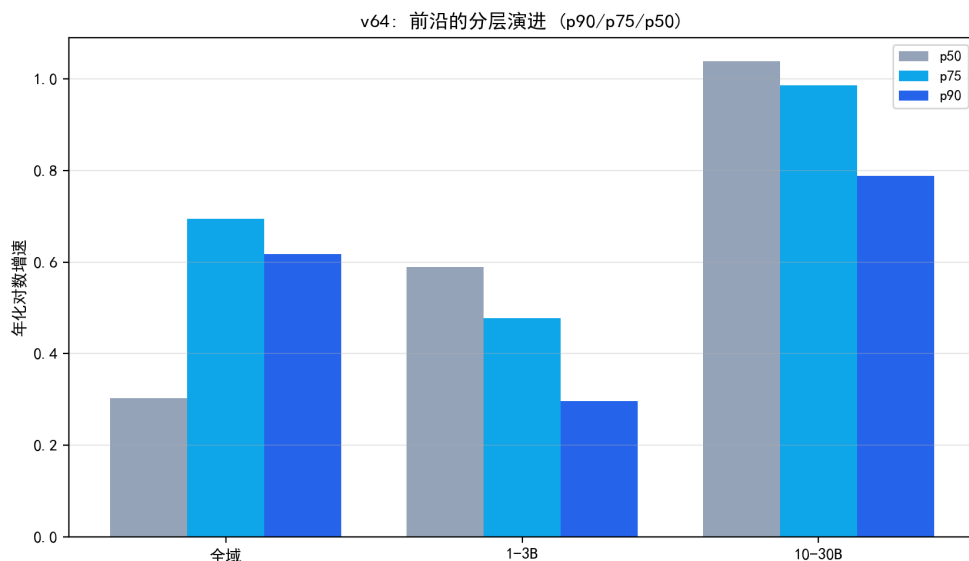
图 8.56 分层演进：全域顶层分化（ p90/p50 \approx 2 ），段内普惠（p50 快于 p90）。
