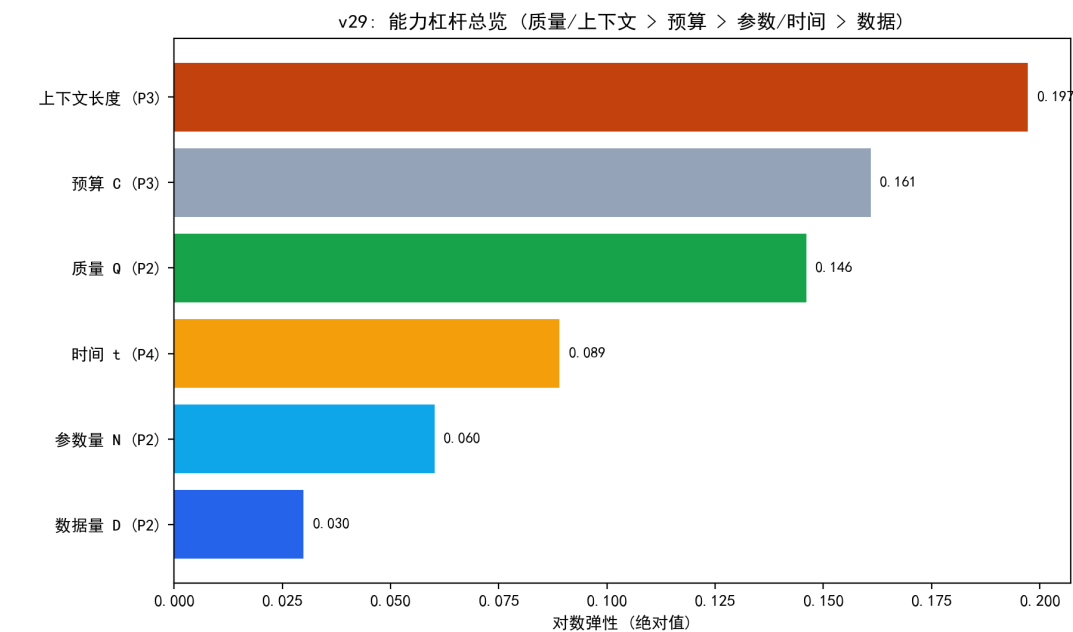
图 10.67 能力杠杆总览：各投入的对数弹性排序（质量/上下文 > 预算 > 参数/时间 > 数据）。
