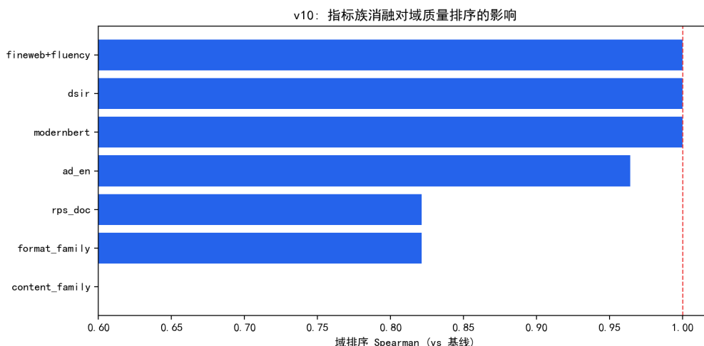
图 9.65 指标族消融对域质量排序的影响（红虚线为完全一致）。
