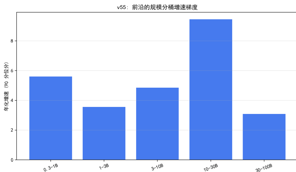
图 8.54 规模分桶的前沿年化增速：10-30B 甜点区最快，30-100B 最慢。
