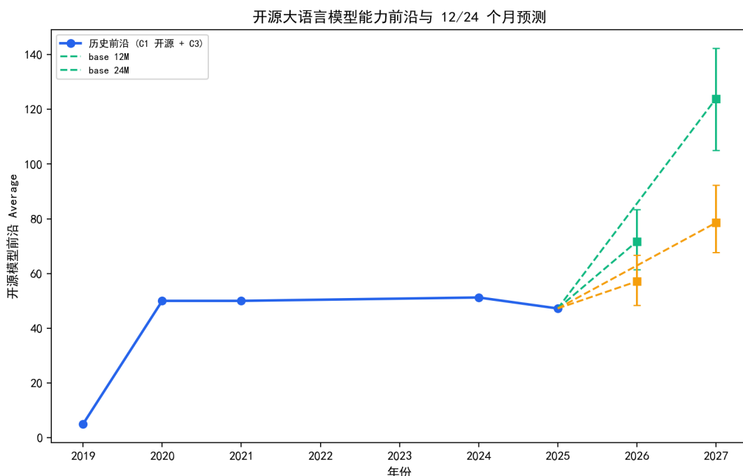
图 8.58 开源模型能力前沿（历史点）与 12/24 个月预测（基础/放缓情景，90% 区间）。
