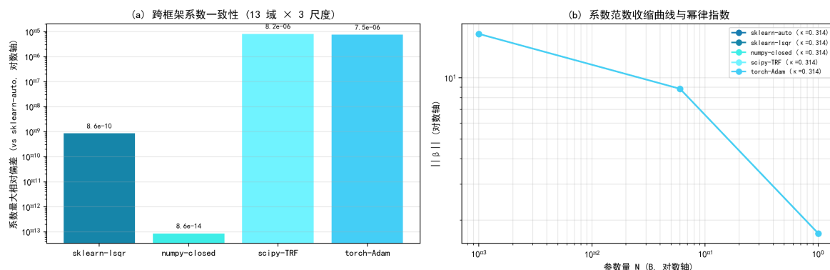
图 5.8 五框架岭回归交叉验证:系数范数收缩曲线完全重合, \kappa = 0.314031 (极差 3 \times 10^{-10} )。
