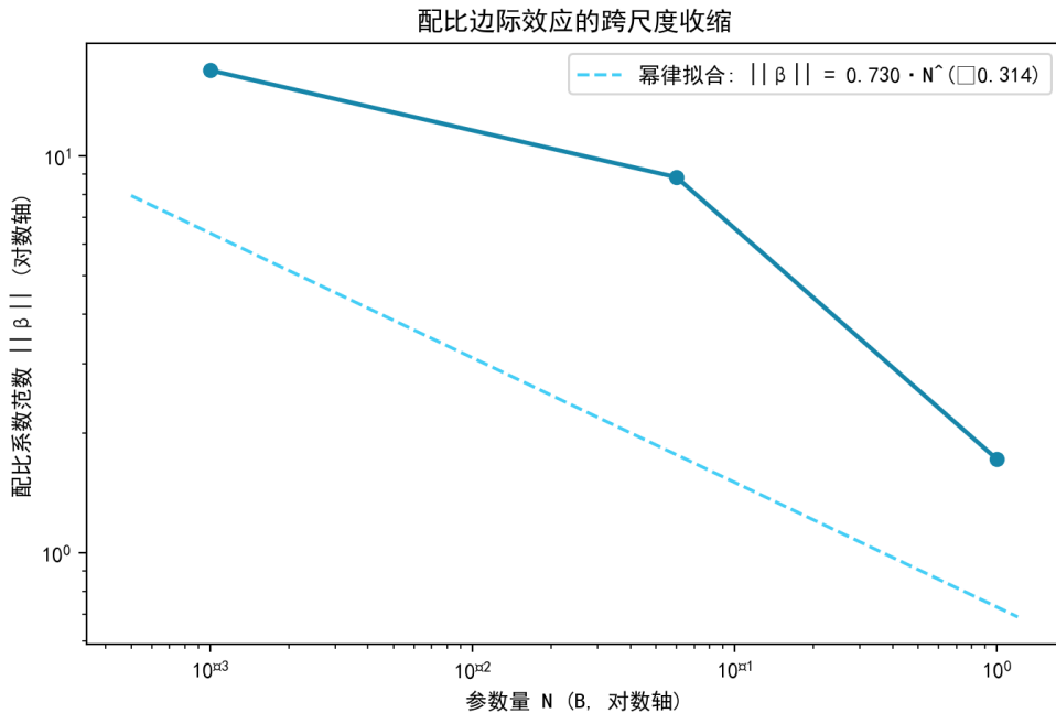
图 5.7 配比系数范数随模型规模幂律收缩（ \kappa = 0.314031 ）。
