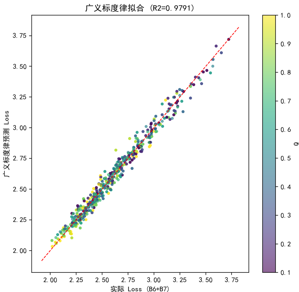
图 6.9 广义标度律在 B6+B7 数据上的拟合（质量-参数数量交互形式， R^2 = 0.979 ）。
