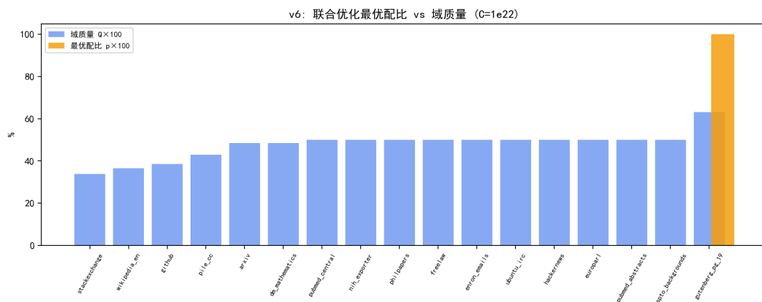
图 7.18 联合优化最优配比与域质量对比 ( C = 10^{22} ): 配比向最高质量域 (小说) 集中。
