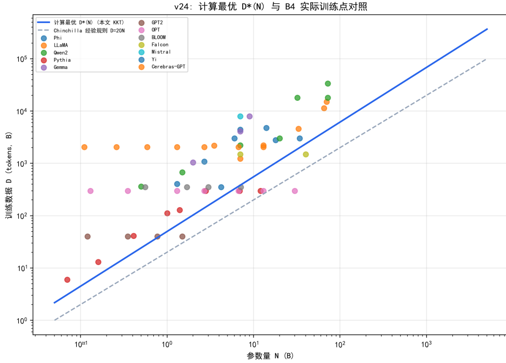
图 7.15 计算最优数据曲线 D^*(N) 、Chinchilla 经验规则与 B4 实际训练点。
