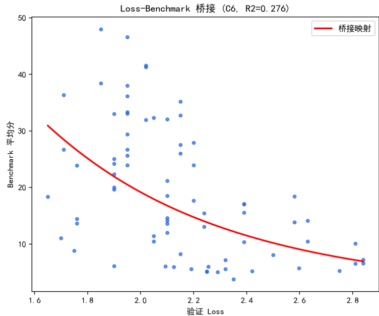
图 8.25 Loss-Benchmark 桥接映射（C6，75 个模型）。
