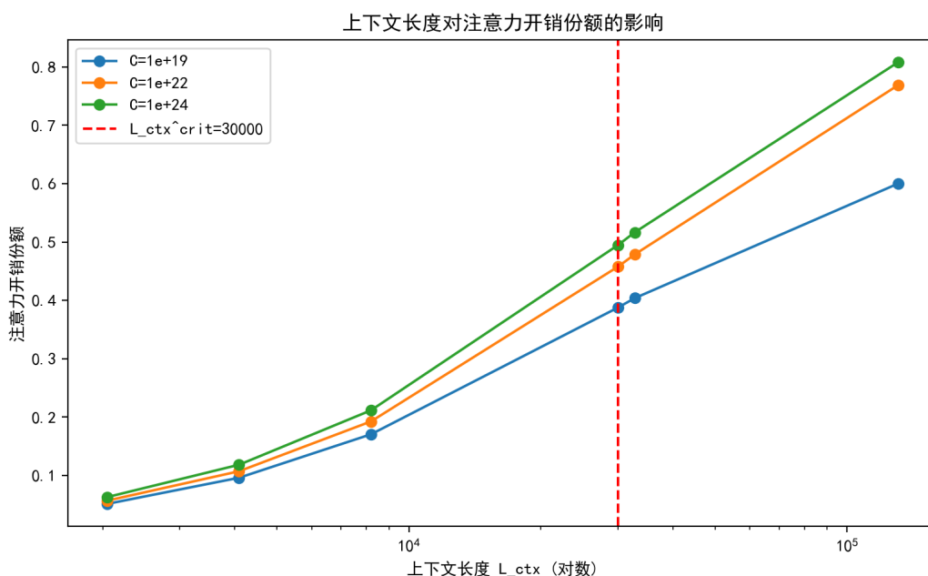
图 7.17 注意力开销份额随上下文长度的变化（红色虚线为临界点 30000）。
