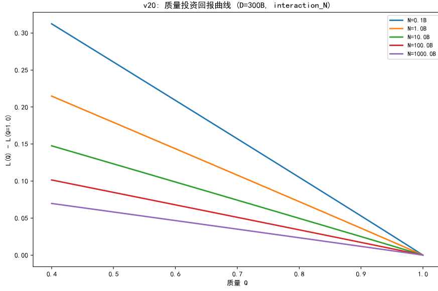
图 6.11 质量投资回报曲线 ( D = 300B ): L(Q) 相对 L(Q = 1) 随 N 变化。
