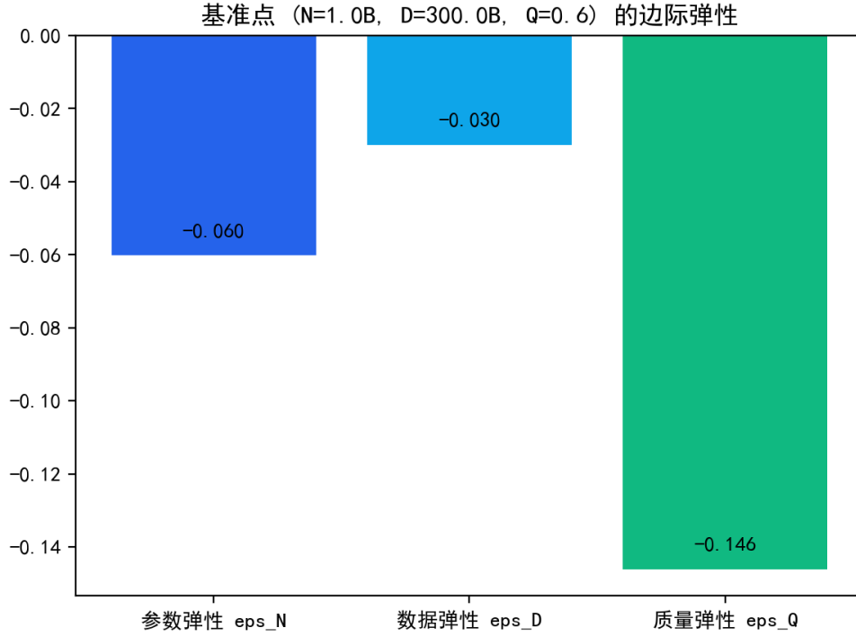
图 6.12 基准点处三个维度的损失弹性对比（质量弹性最高）。
