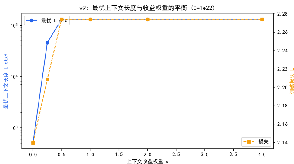
图 7.20 最优上下文长度与收益权重 w 的平衡 ( C = 10^{22} )。
