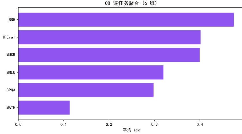
图 8.26 C8 逐任务聚合得分 (6 维)。
