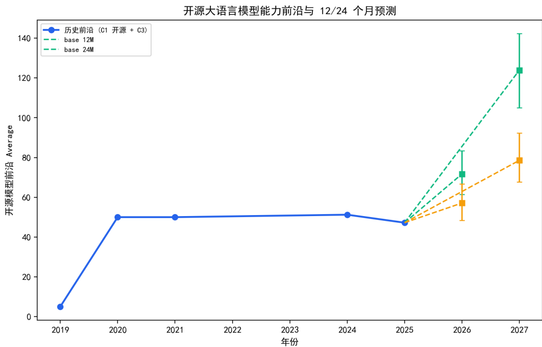
图 8.22 开源模型能力前沿（历史点）与 12/24 个月预测（基础/放缓情景，90% 区间）。
