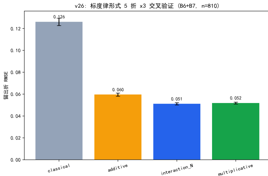
图 6.8 标度律形式 5 折交叉验证的留出 RMSE 对比。
