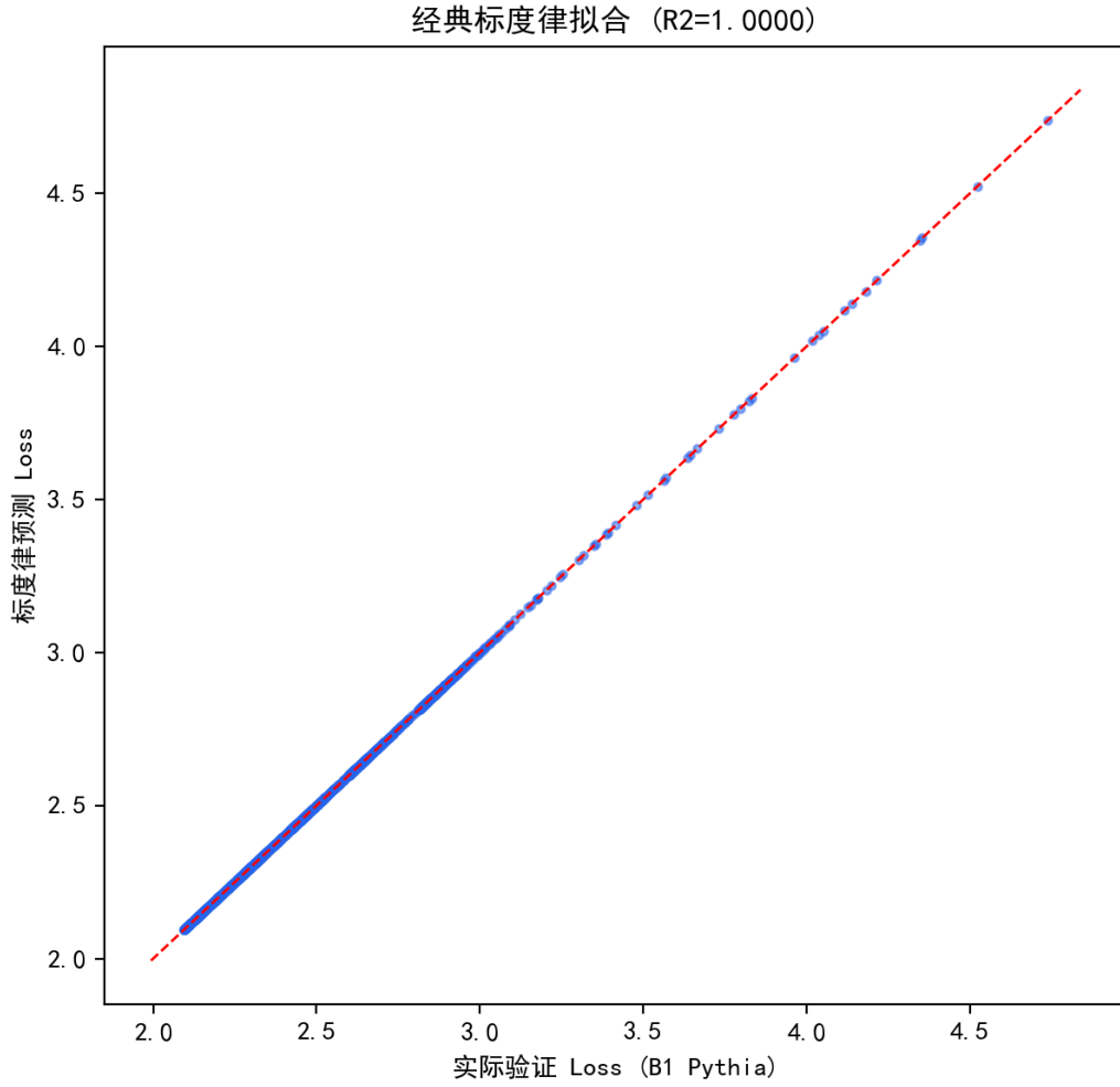
图 6.7 经典标度律在 B1 轨迹上的拟合与跨家族验证。
