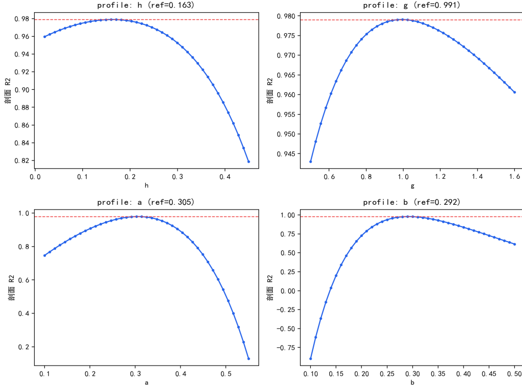
图 6.10 关键参数的剖面似然曲线（红色虚线为 90% 似然比阈值）。
