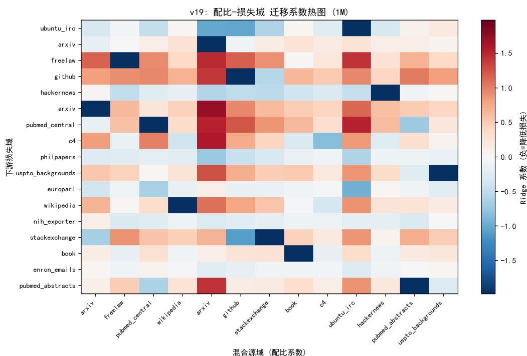
图 5.5 配比源域 \times 损失域迁移系数热图 (1M 尺度，负值 = 压低损失)。
