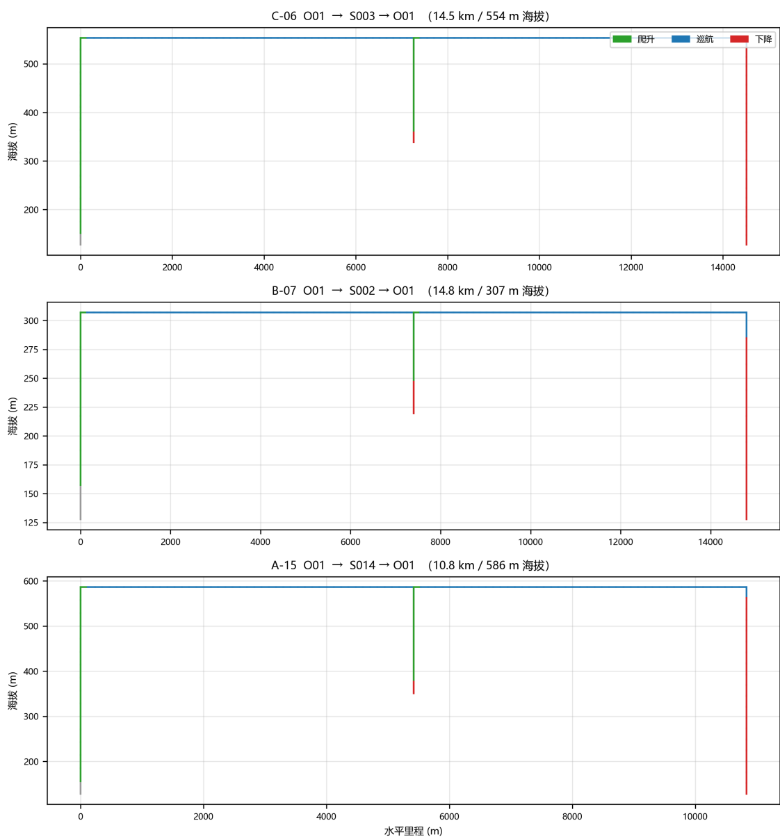
图 5.11 代表性架次高度剖面(爬升-巡航-下降相位着色):体现航线严格贴地形走廊+50 m 巡航、终点下降至服务区上方 30 m 投送
