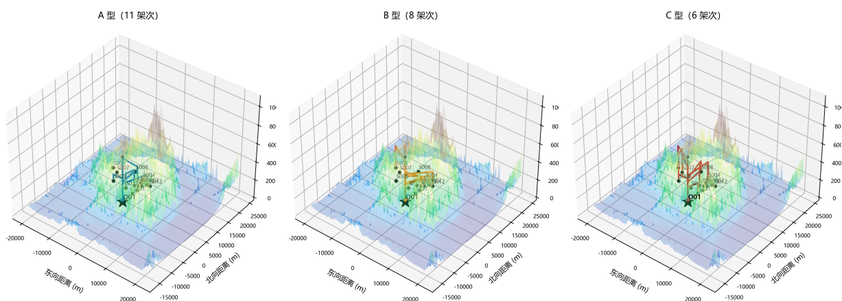
图 5.10 分机型三维航线：C 型 6 架次构成重区满载走廊，B 型 8 架次以三箱满载链覆盖轻区与中距区，A 型 11 架次执行短途轻载与尾箱投送
