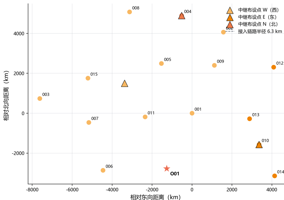
图 6.17 三个中继布设点及其接入链路半径示意（虚线圆半径 6.3 km）
