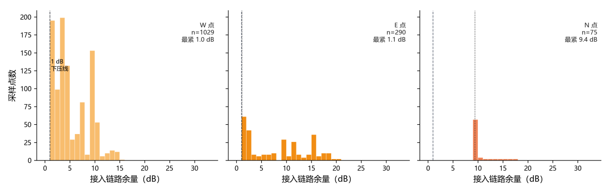
图 7.23 三个布设点接入链路余量分布（虚线为 1 dB 下压线）
