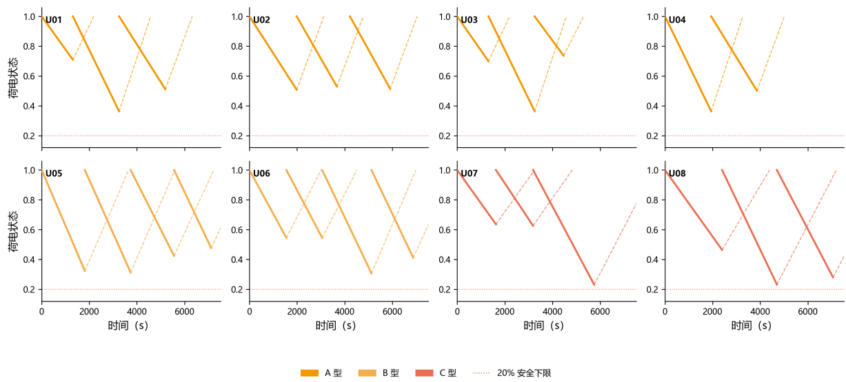
图 5.15 8 架无人机的荷电状态轨迹（实线为飞行段，虚线为充电段）
