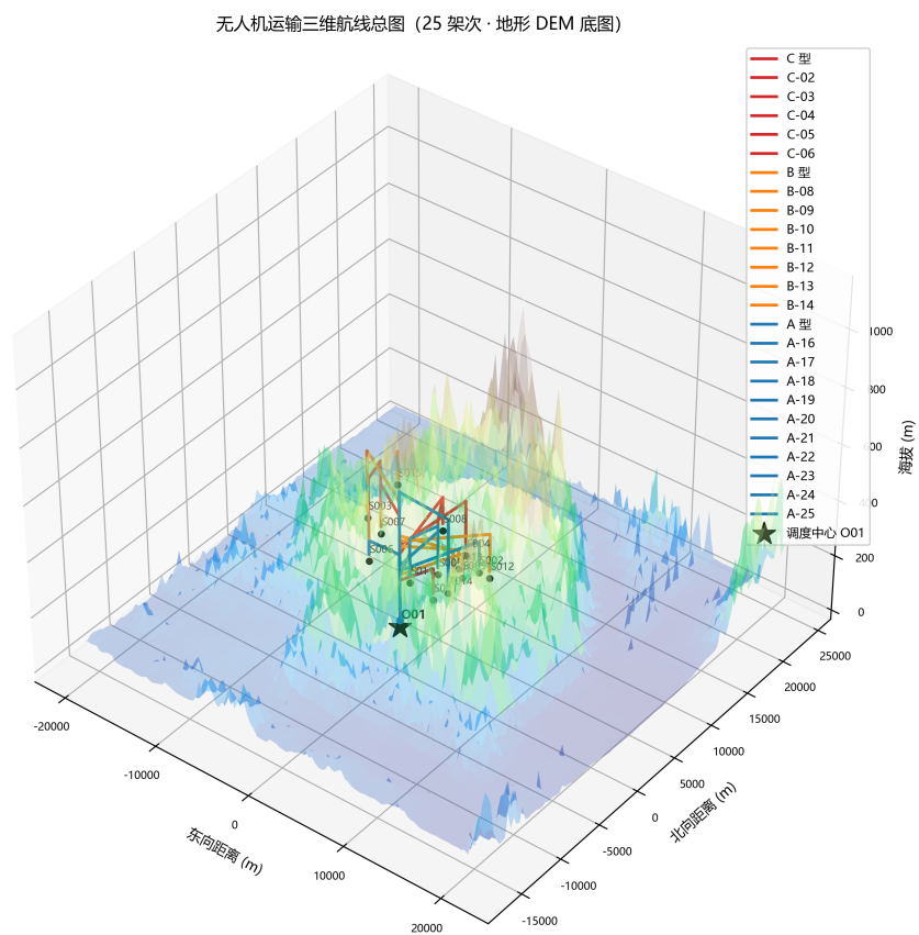
图 5.9 均衡方案三维航线总图 (30 m DEM 地形底图；按机型着色：C 型红色远距重载走廊、B 型橙色满载链、A 型蓝色短途轻载；统一视角 elev=26°、azim=-58°)
