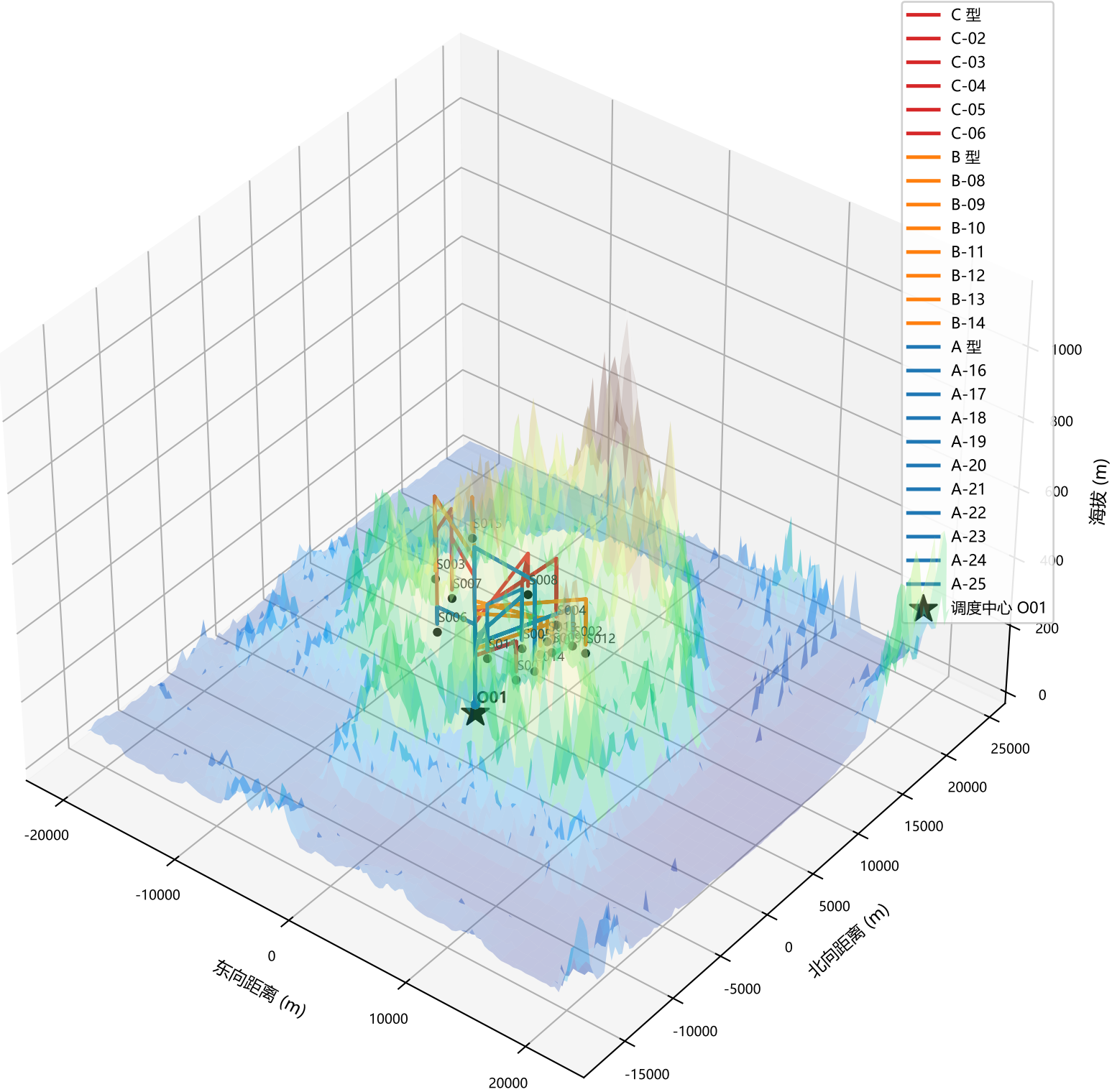
无人机运输三维航线总图 (25 架次 · 地形 DEM 底图)
