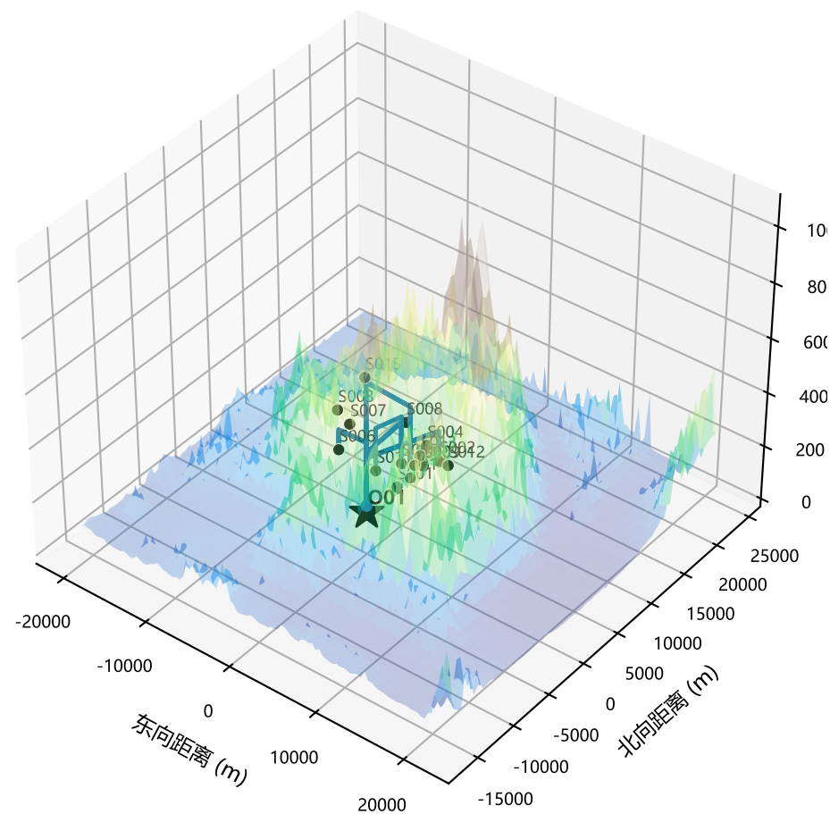
A 型 (11 架次)
