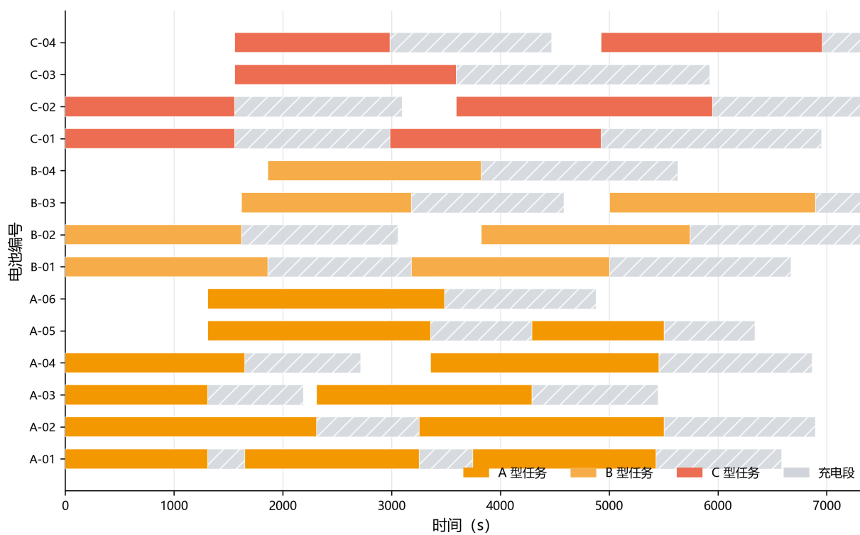
图 5.11 14 组共享电池的任务与充电时间线（斜纹为充电段）
