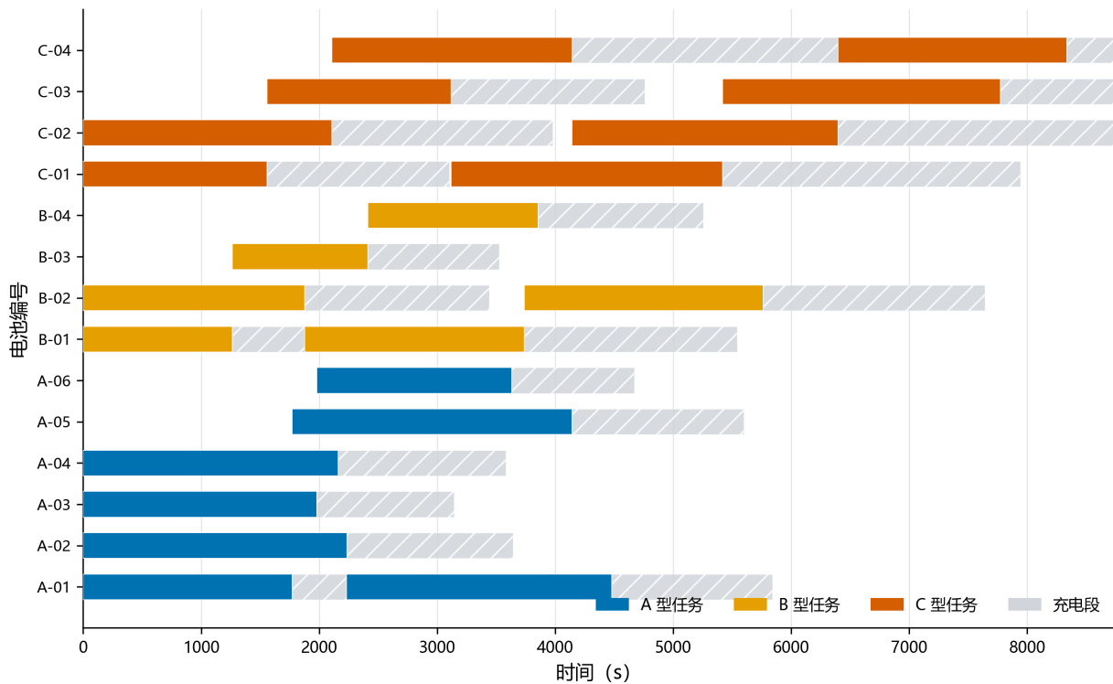
图 5.8 14 组共享电池的任务与充电时间线（斜纹为充电段）
