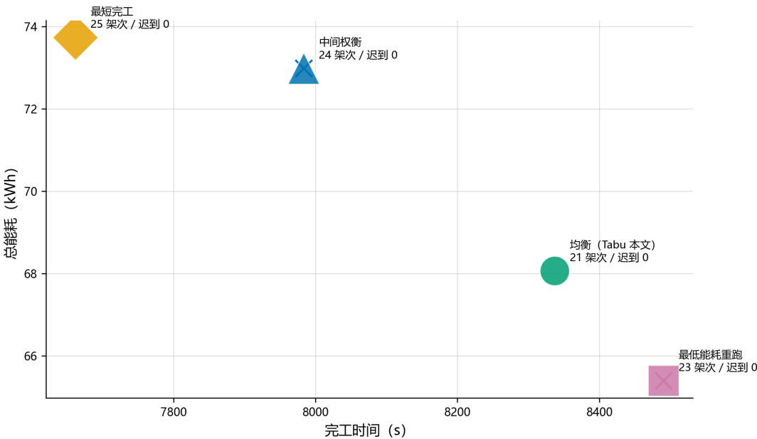
图 5.5 问题二多目标权衡（气泡大小为架次数）
