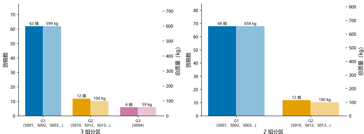
图 8.17 三组与两组方案各组货箱数与总质量对比
