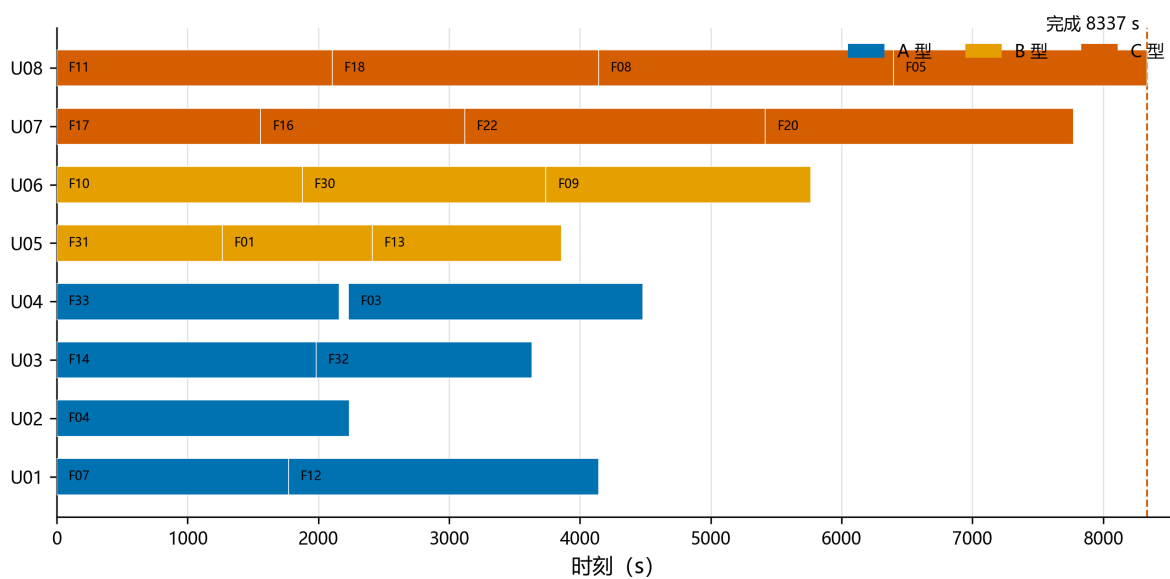
图 5.7 问题二均衡方案的运输任务甘特图（按无人机分泳道）
