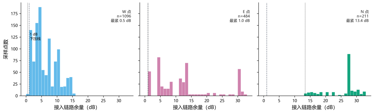
图 7.15 三个布设点接入链路余量分布（虚线为 1 dB 下压线）
