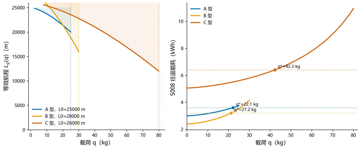
图 4.2 左：等效航程随载荷收缩曲线；右：三机型到 S008 往返能耗随载荷变化及能量上限交点
