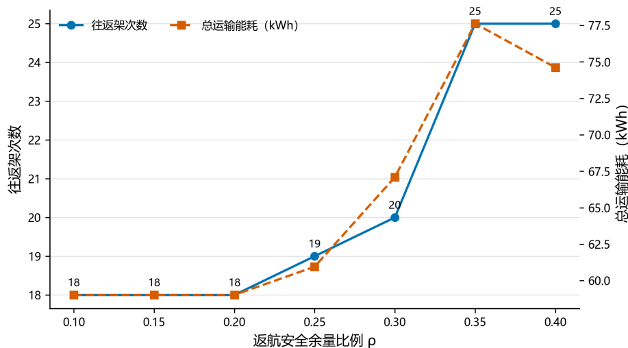
图 7.14 返航安全余量比例对架次数与总能耗的影响
