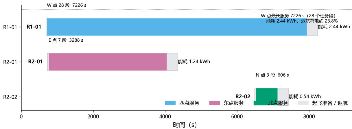
图 6.11 两架中继三个服务时段的时间线（浅灰为起飞准备与返航）
