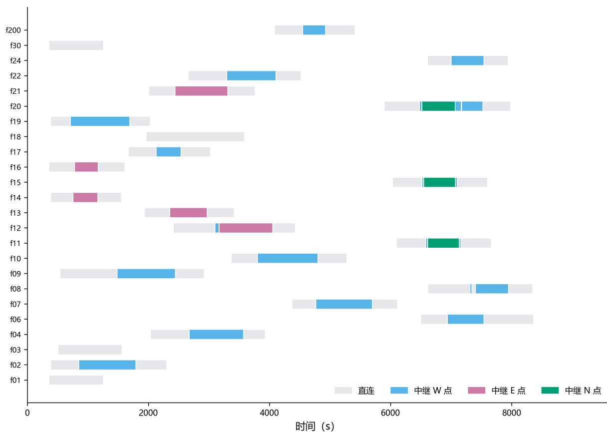
图 6.12 各运输架次的通信保障方式时间线（浅灰为直连，彩色为中继）
