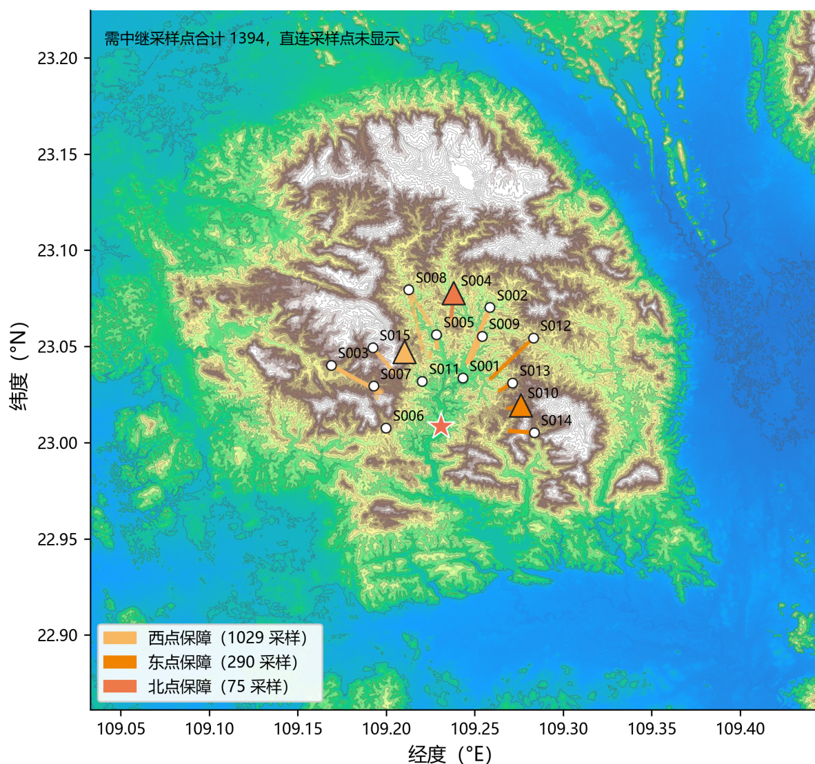
图 6.15 1394 个需中继采样点按布设点的归属分布 (DEM 底图)
