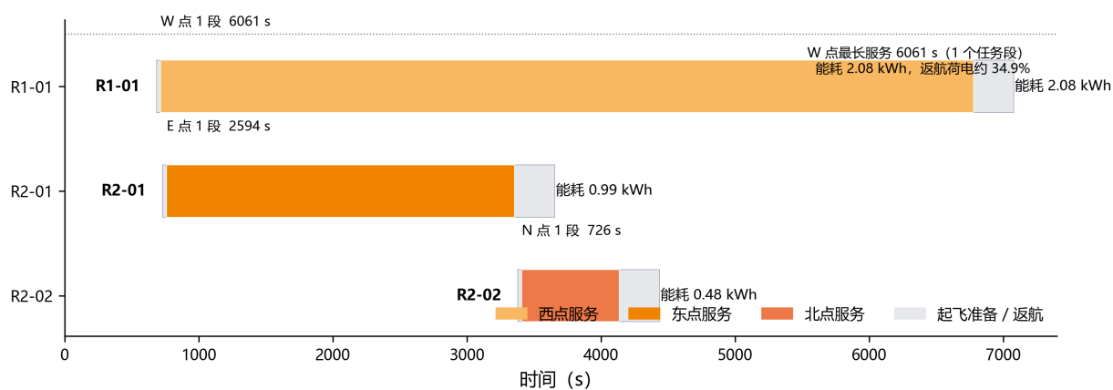
图 6.16 两架中继三个服务时段的时间线 (浅灰为起飞准备与返航)
