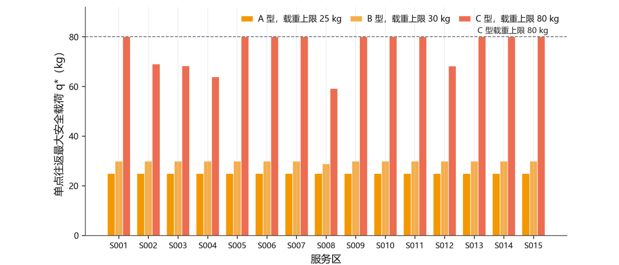
图 5.5 三机型在各服务区的最大安全载荷对比
