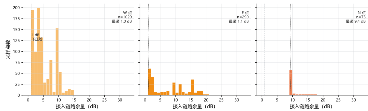
图 8.23 三个布设点接入链路余量分布（虚线为 1 dB 下压线）
