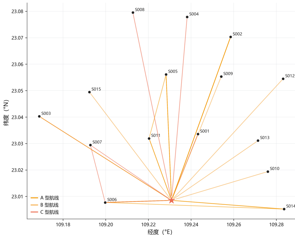
图 6.8 问题二均衡方案航线网络（按机型着色）
