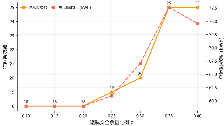
图 8.22 返航安全余量比例对架次数与总能耗的影响
