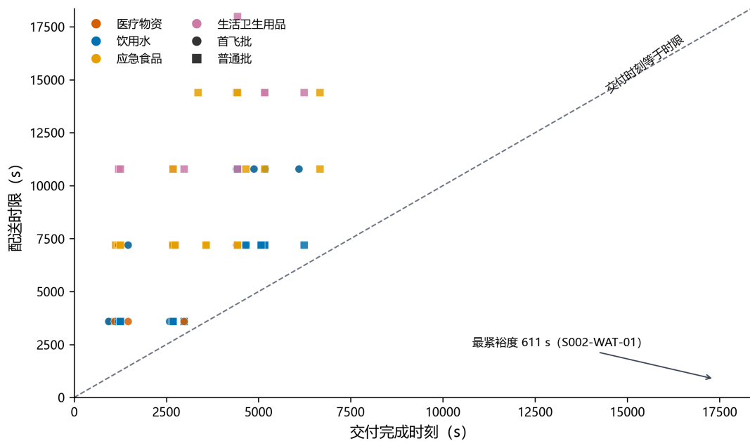
图 5.9 逐箱交付时刻与配送时限（圆点为首飞批，方块为普通批）
