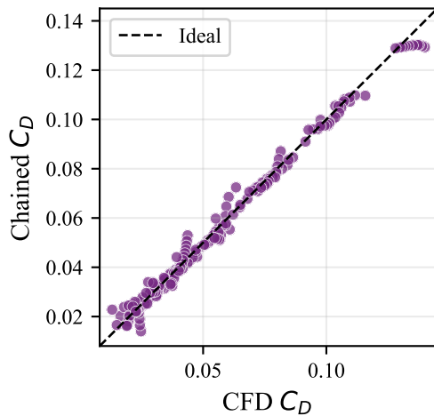
(d) MLP aero — C_D
