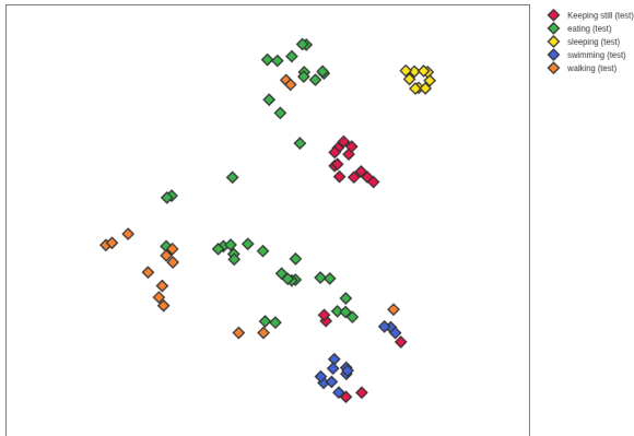
Fig. 3: アジアゾウデータセットにおけるt-SNE可視化結果. ホッキョクグマと比較してクラスタの分離が不明瞭
