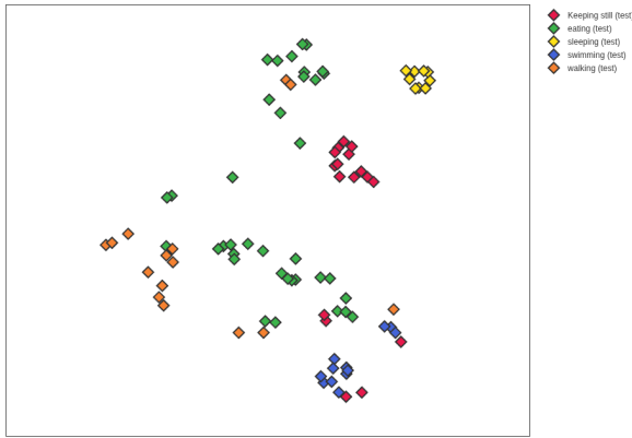
Fig. 4: アジアゾウデータセットにおけるt-SNE可視化結果. ホッキョクグマと比較してクラスタの分離が不明瞭
