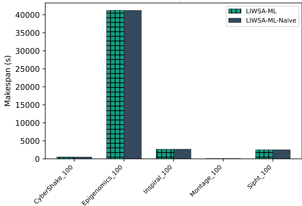
Makespan
