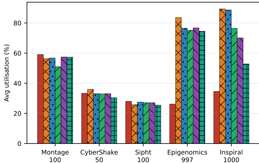
VM resource utilisation
