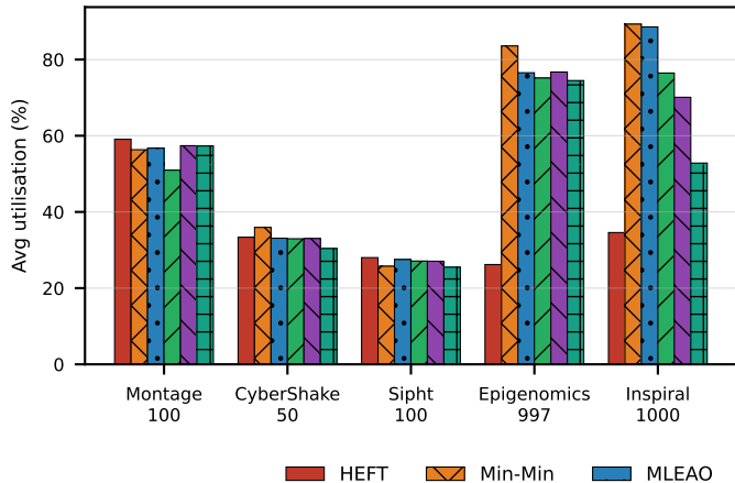
VM resource utilisation
