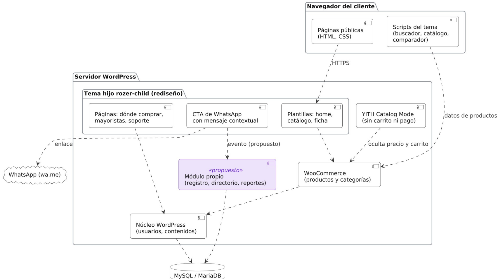
V3-05 · Diagrama de componentes de la web renovada (adaptado de D-19)
