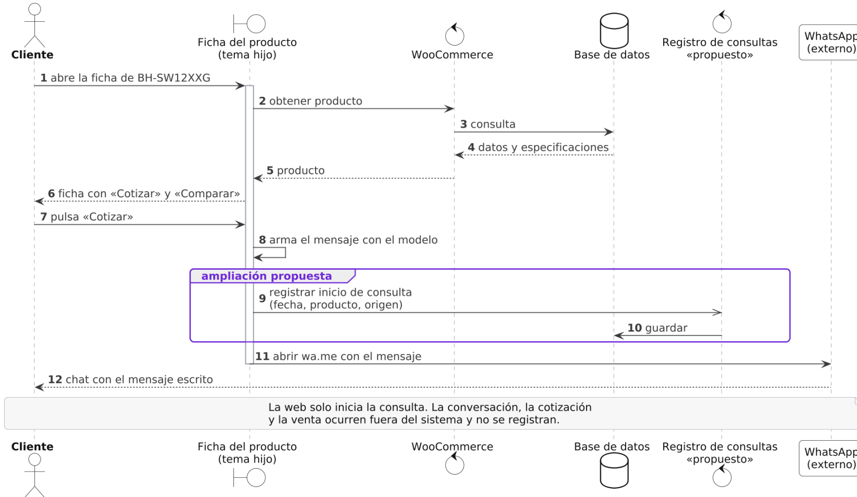
V3-03 · Secuencia: consulta de un producto por WhatsApp (adaptado de D-14)
