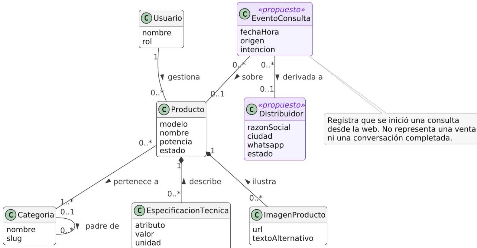
V3-04 · Diagrama de clases del dominio (adaptado de D-07)
