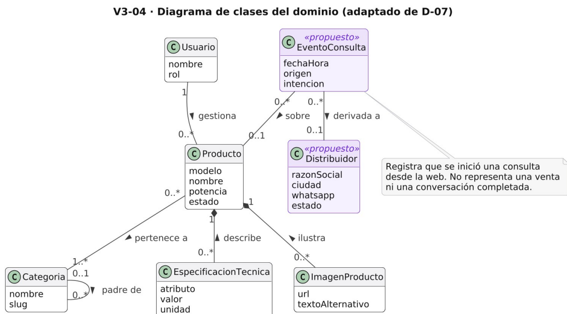
Figura 9. Clases del dominio
