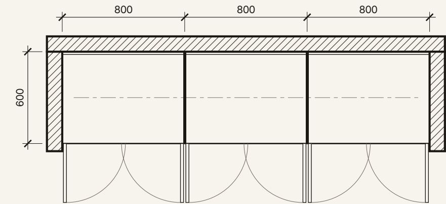
03 PLAN 1 : 25
