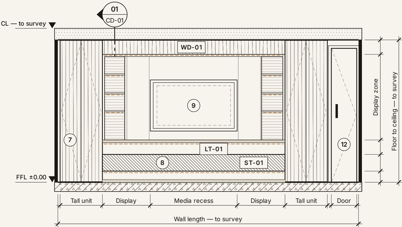
E1 DD-02 MEDIA WALL — ELEVATION
