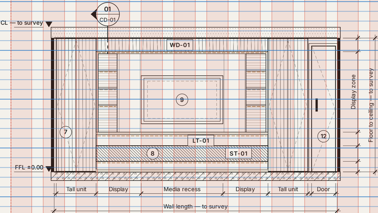
E1 MEDIA WALL — ELEVATION DD-02
