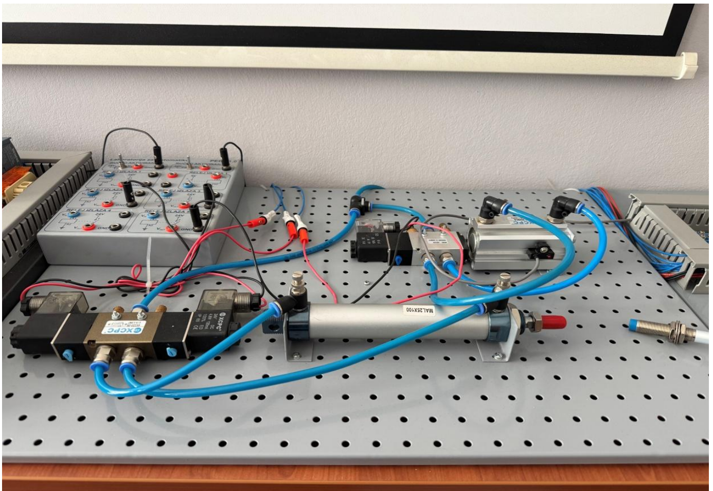
Слика 4.5.1.1. Извршни електропнеуматски систем у лабораторијском окружењу
