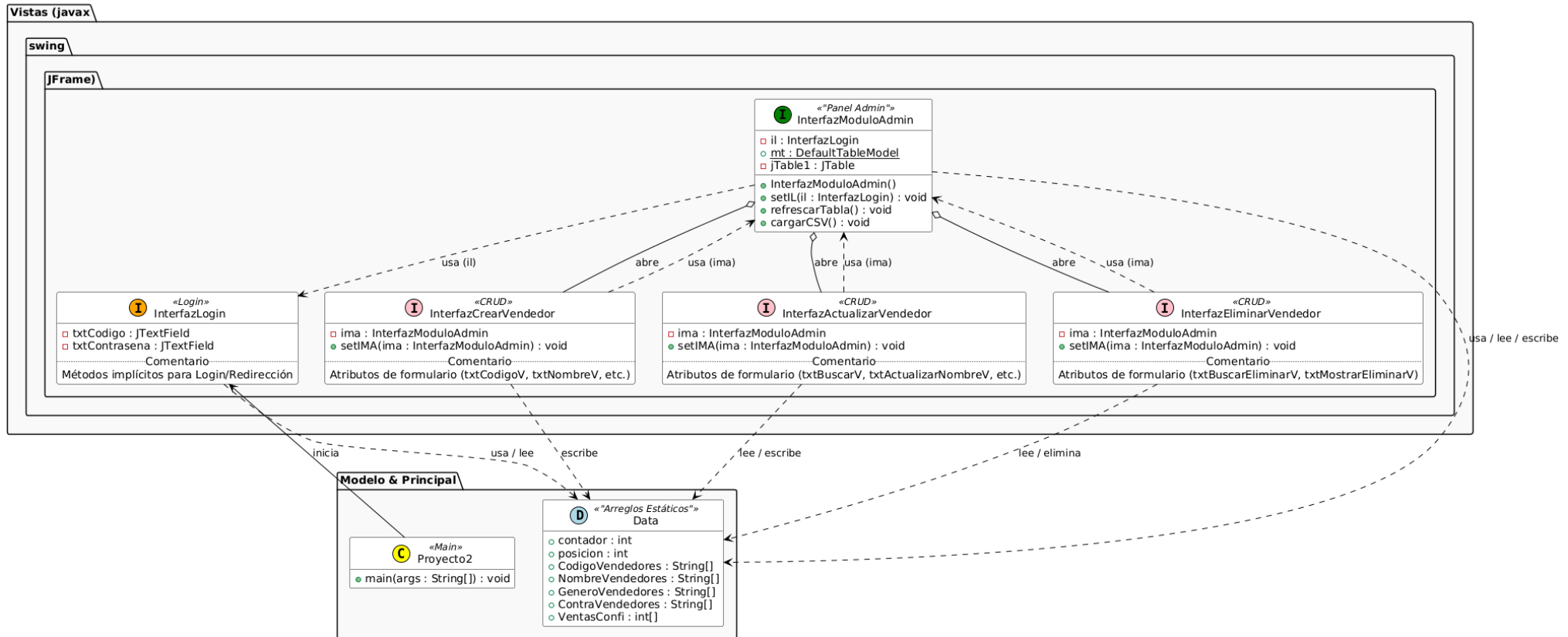
Diagrama de Clases - Código Fuente Actual
