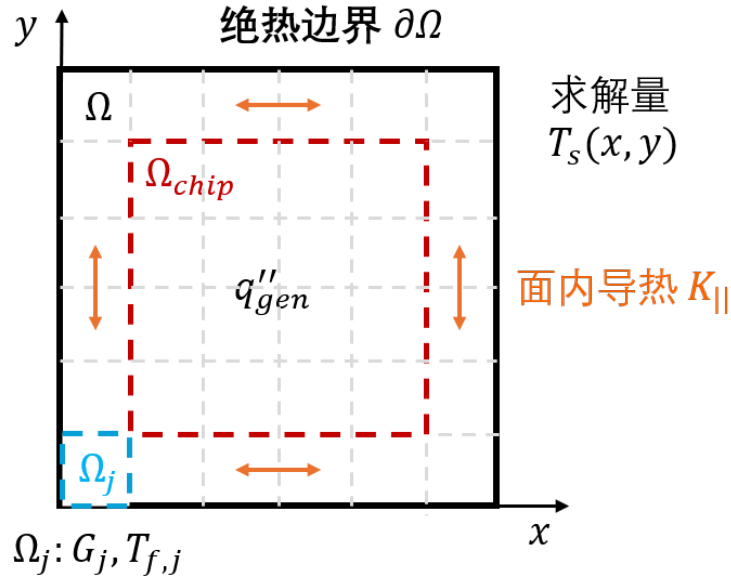
图 5 芯片与衬底的二维导热示意。 \Omega 为整个散热区域，中央 \Omega_{chip} 为芯片热源投影区域，面热源为 q''_{gen} ；每个区域 \Omega_j 的 G_j 表示传热率与固液温差之比， T_{f,j} 为冷却液代表温度。 K_{||} 表示固体的面内导热参数，外边界 \partial\Omega 采用绝热条件，待求的是固体温度场 T_s(x, y) 。
