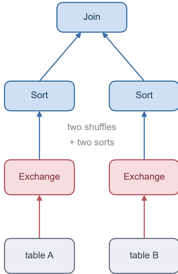
SortMergeJoin
