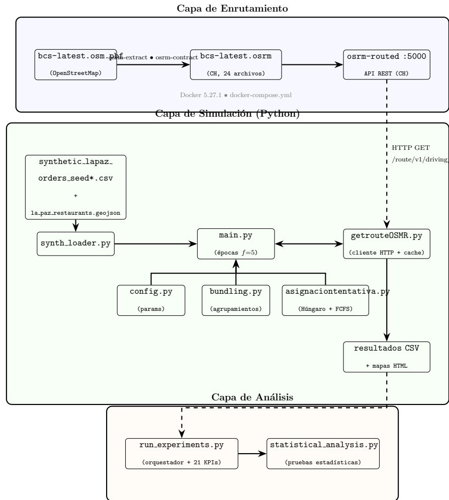
Figura 3.1: Arquitectura de tres capas del entorno de simulación MDRP-BCS.
