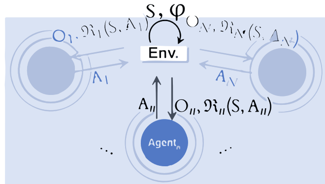
(d) Dec-POMDP
