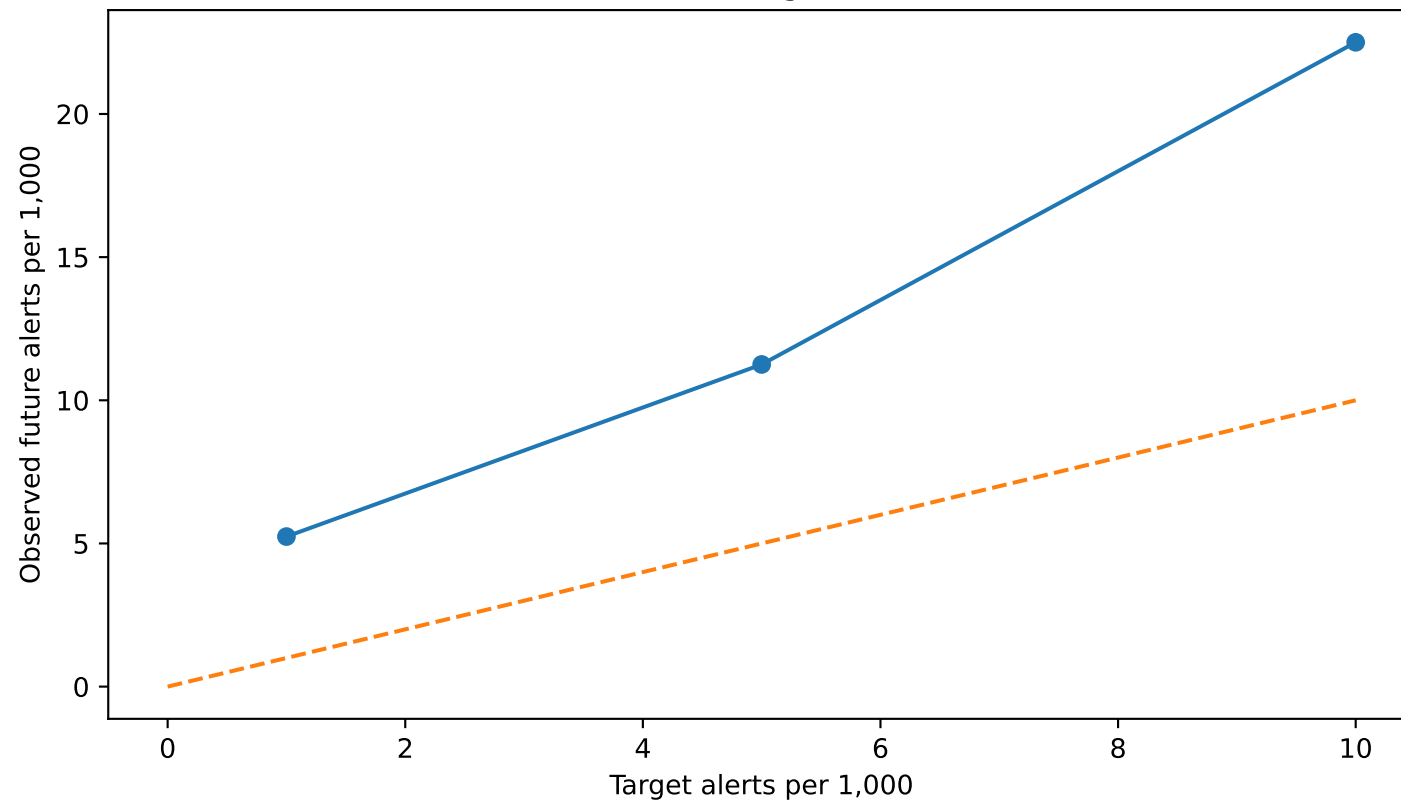
(c) EVT alert-budget calibration
