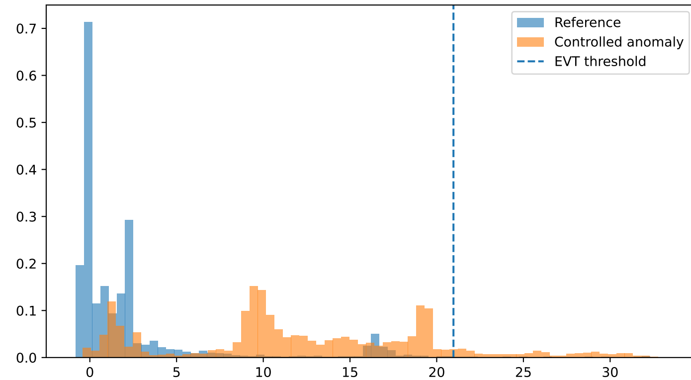
(d) Score distributions and label-free threshold
