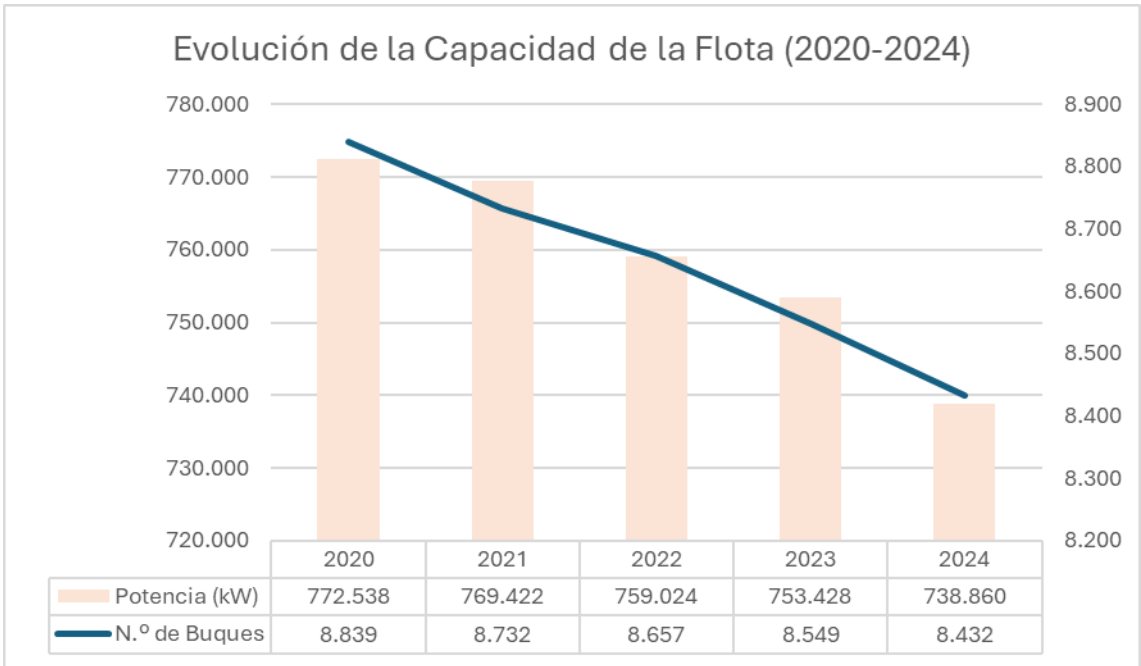
Figura 5. Evolución de la Capacidad de la Flota Pesquera. Elaboración propia. Fuente: Registro General de Flota Pesquera (RGFP)
