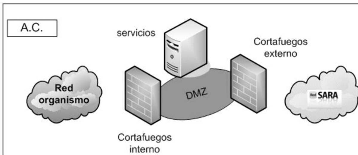
Ilustración 8. Esquema lógico de un área de conexión (AC)
