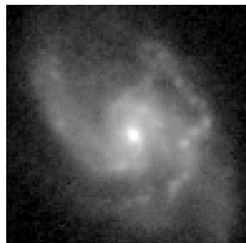
NEXUS F200W
