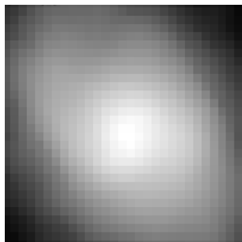
Euclid H_E
