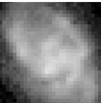
Euclid VIS
