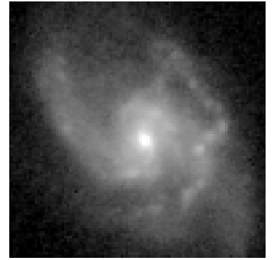
NEXUS F200W
