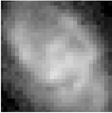
Euclid VIS
