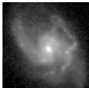
NEXUS F200W
