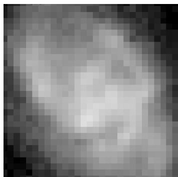
Euclid VIS
